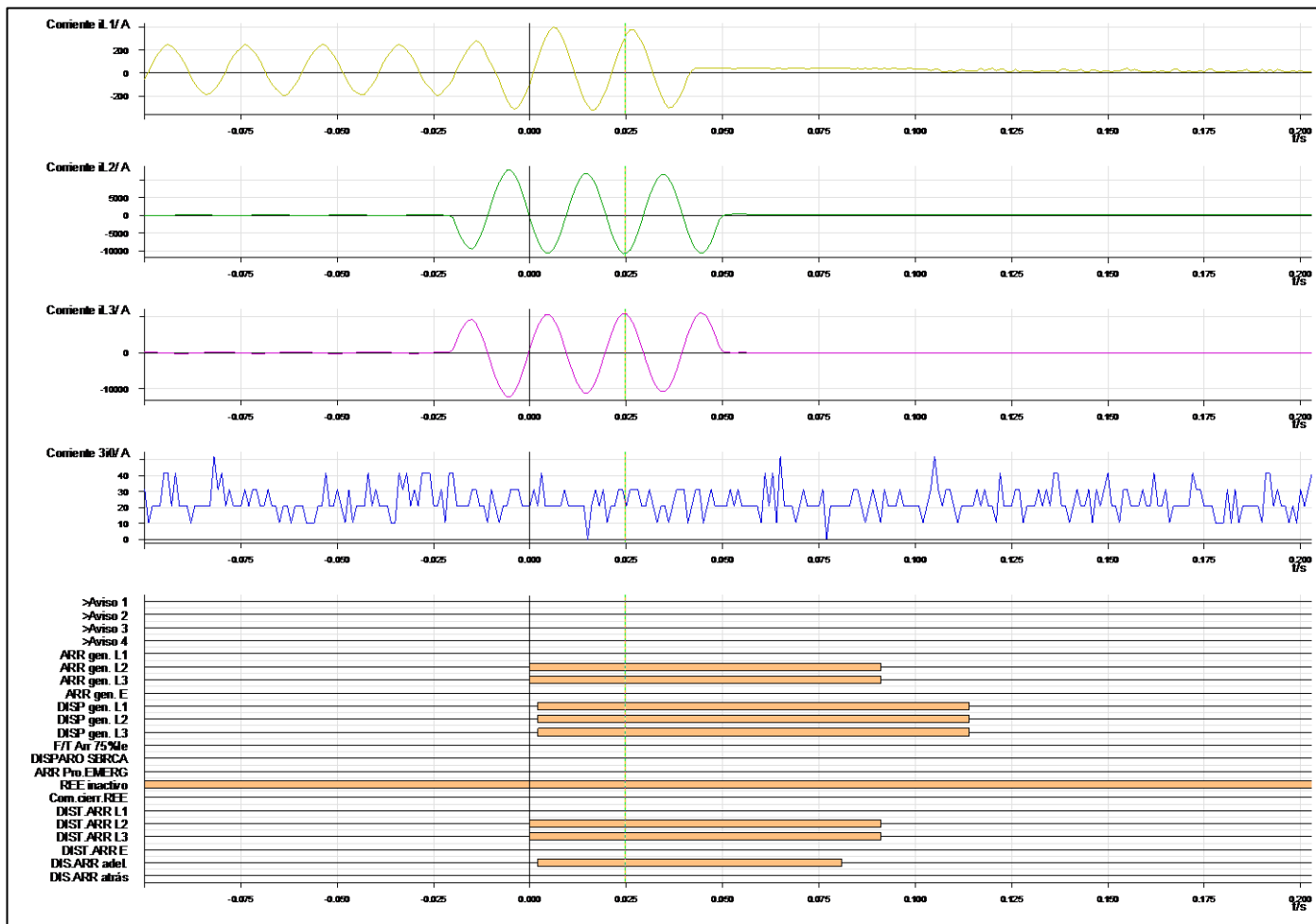
Registro oscilográfico 1
