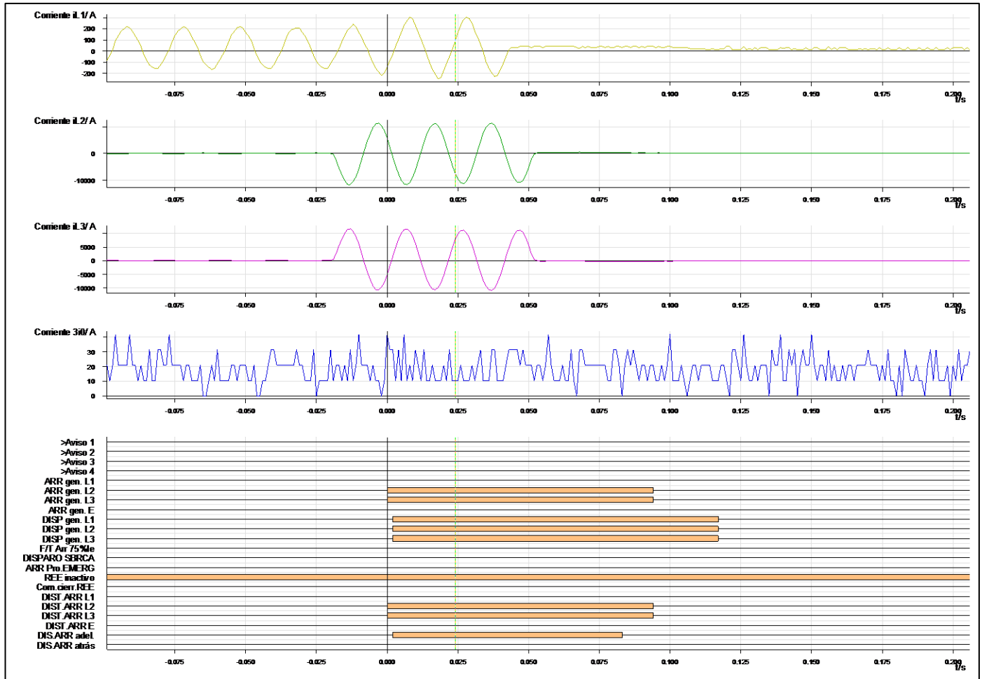
Registro oscilográfico 2
