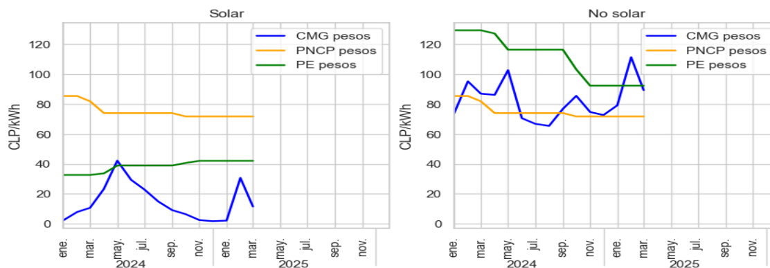
Gráfico 3.2. Comparativa CMg-PNCP-PE barra Quillota 220 kV Enero de 2024 a Marzo de 2025
