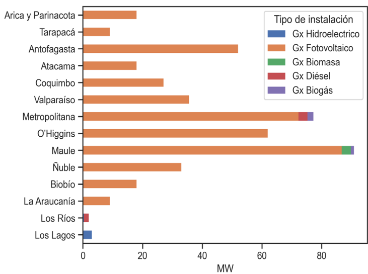
Gráfico 5.2. Proyectos PMGD en proceso de conexión por tecnología y región a marzo de 2025.
