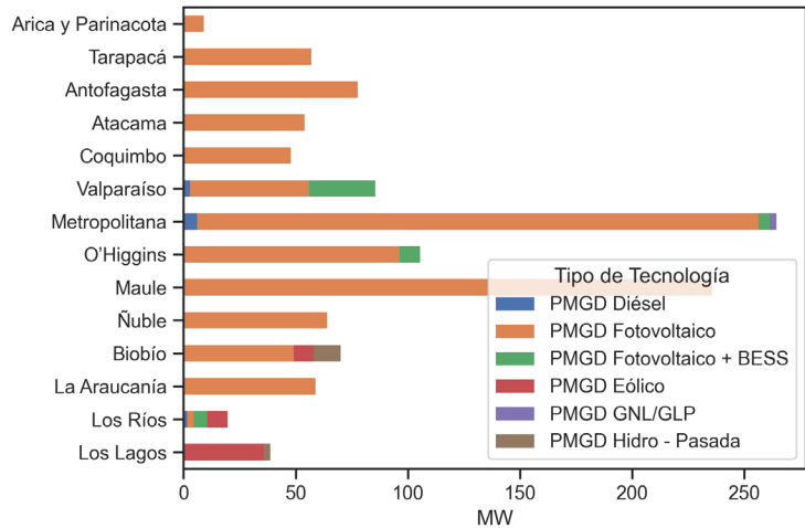
Gráfico 5.1. Proyectos PMGD declarados en construcción por tecnología y región a marzo de 2025.
