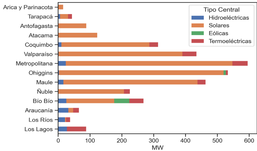
Gráfico 2.2. Potencia instalada PMGD por tipo de tecnología por región actualizado a marzo de 2025
