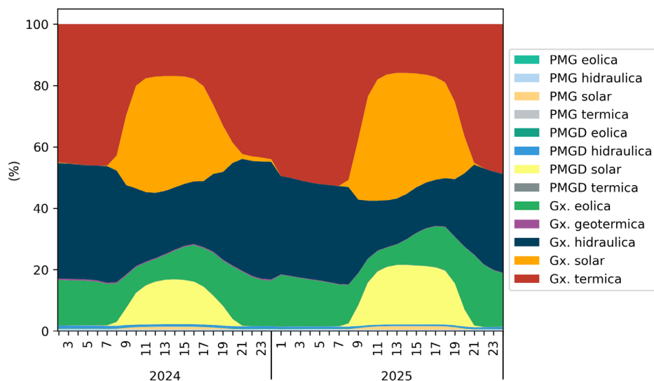
Gráfico 2.4. Generación horaria por tipo de central y tecnología
