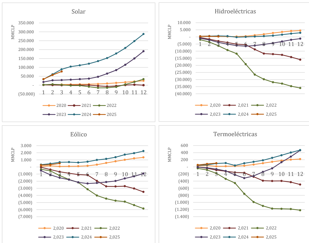
Gráfico 4.2.2 Compensaciones acumuladas por precio estabilizado por año
