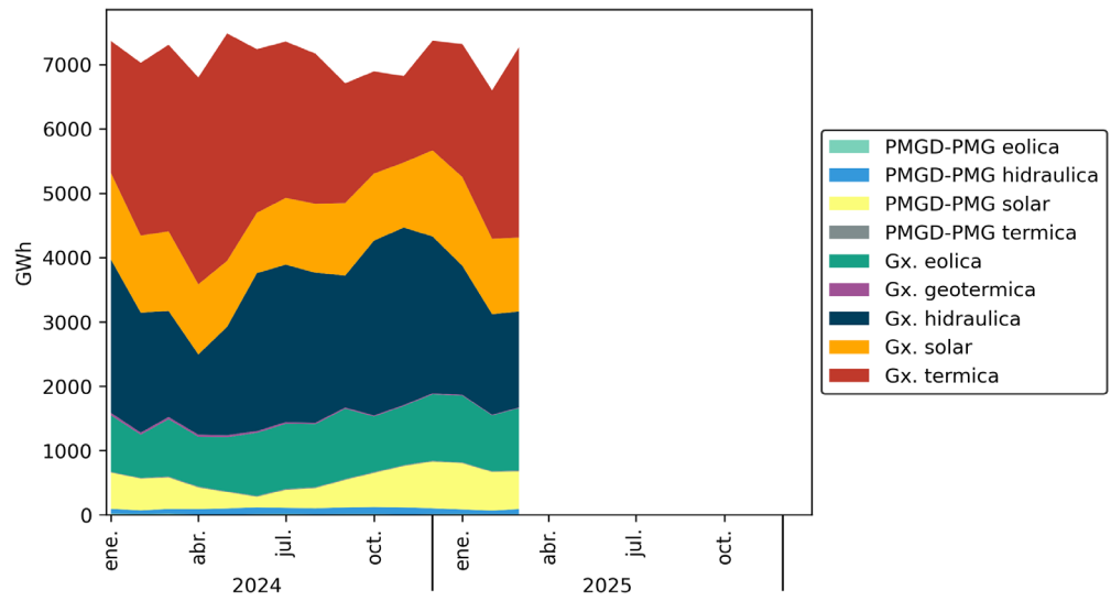
Gráfico 2.3. Generación mensual por tecnología
