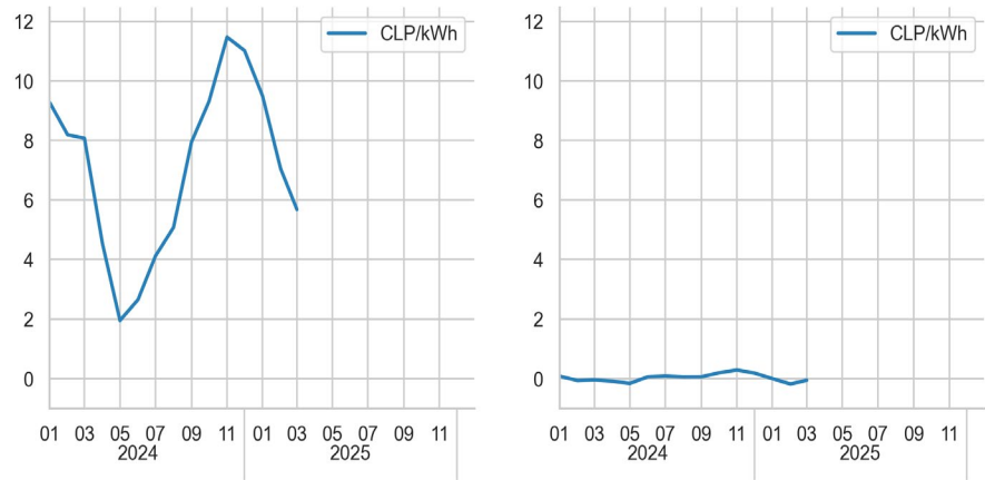
Gráfico 4.4. Costos por compensaciones por kWh de retiro desde enero de 2024 a marzo de 2025, en hora solar y no solar.
