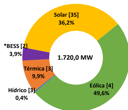
Figura 2: Centrales SEN en pruebas según tecnología.
