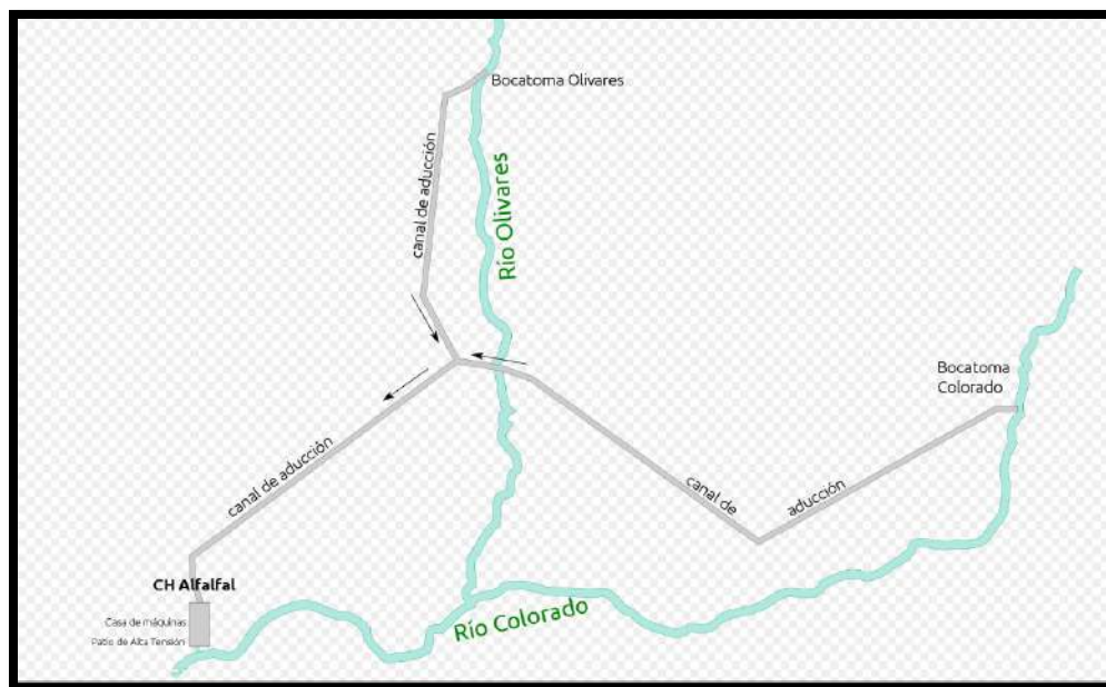
Fig. 2: Esquema de túneles que suministran el caudal de agua provenientes de los ríos Olivares y Colorado a la central Alfalfal.
