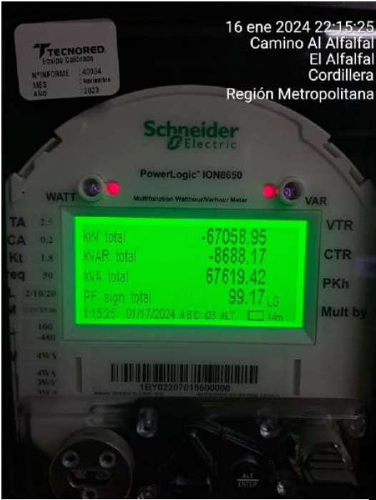
Fig. 4: Medidor de energía conectado a los bornes del generador unidad 1.
