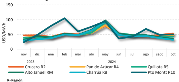
Evolución Costo Marginal Promedio Mensual - Últimos 12 meses
