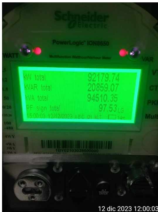
Fig. 3: Medidor de energía facturación.
