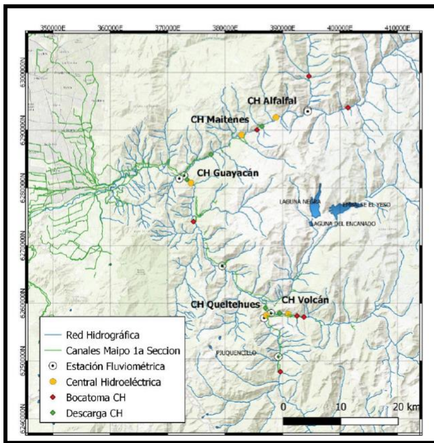
Fig. 1: Ubicación geográfica de Central Alfalfal con respecto a otras centrales hidráulicas en la misma zona.
