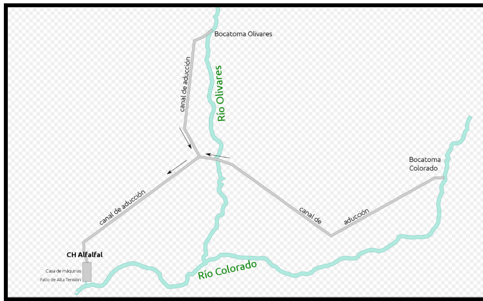
Fig. 2: Esquema de túneles que suministran el caudal de agua provenientes de los ríos Olivares y Colorado a la central Alfalfal.
