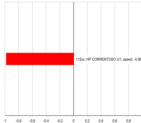
Mode 2083: Participation
