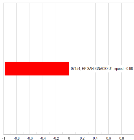
Mode 954: Participation
