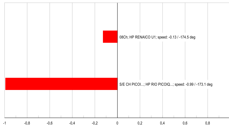
Mode 2180: Participation
