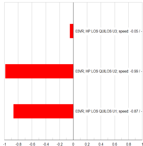
Mode 1059: Participation
