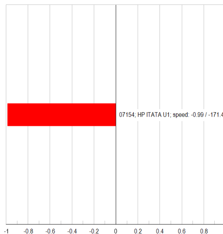
Mode 885: Participation
