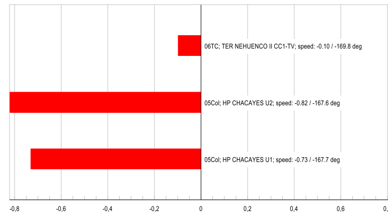
Mode 1661: Participation
