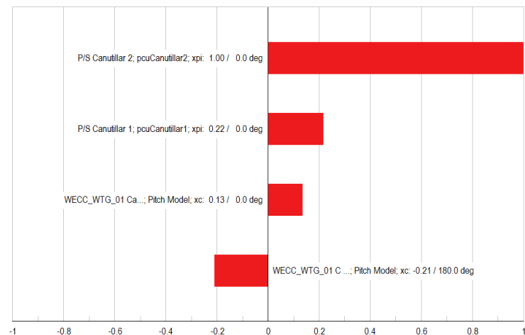
Mode 3: Participation
