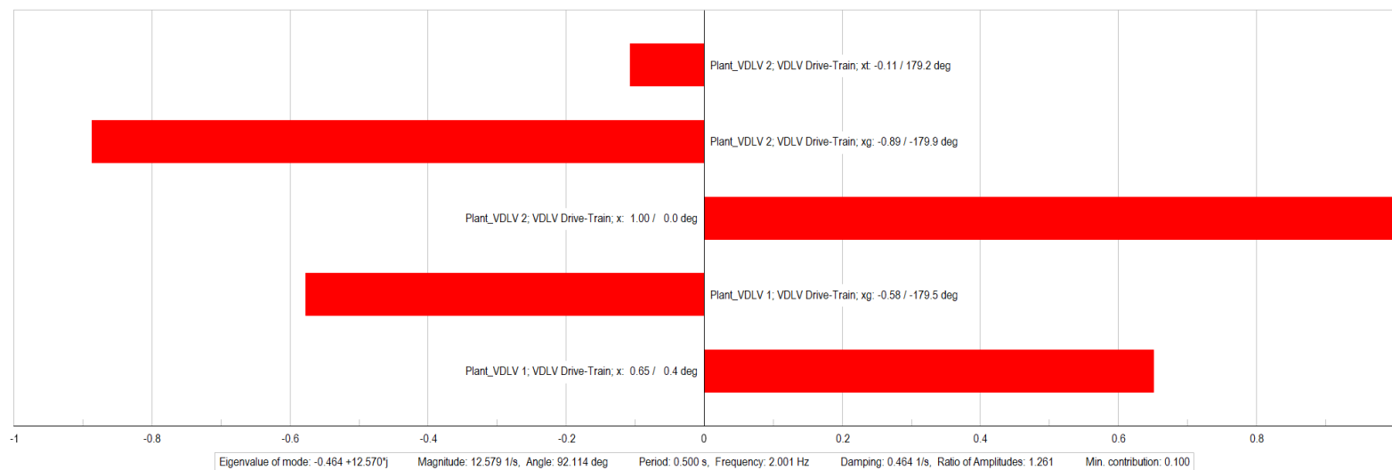
Mode 706: Participation
