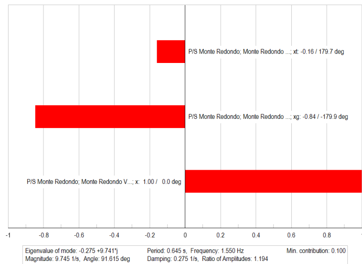
Mode 681: Participation
