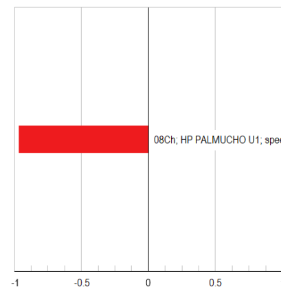
Mode 125: Participation
