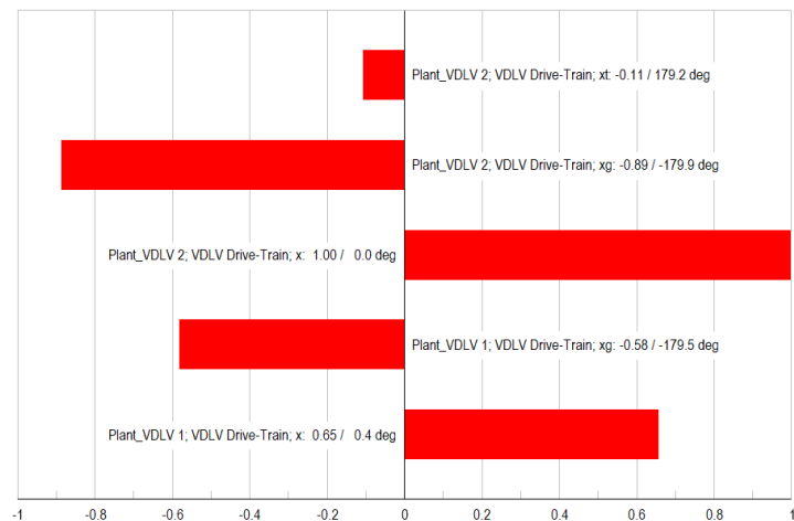
Mode 768: Participation
