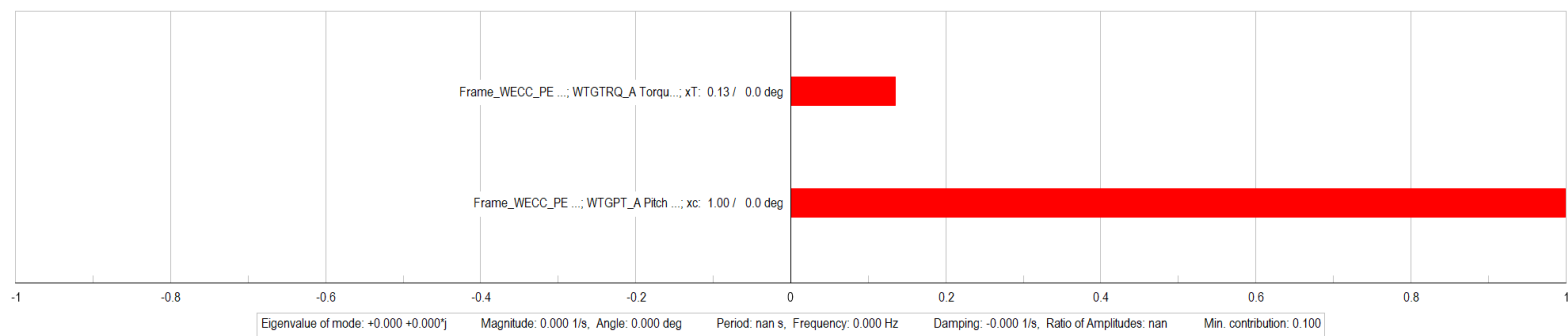
Mode 2: Participation
