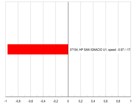
Mode 47: Participation
