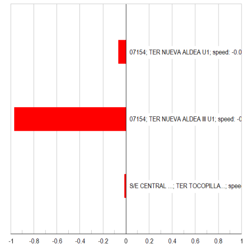
Mode 771: Participation
