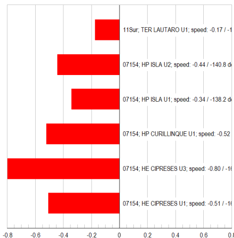
Mode 992: Participation
