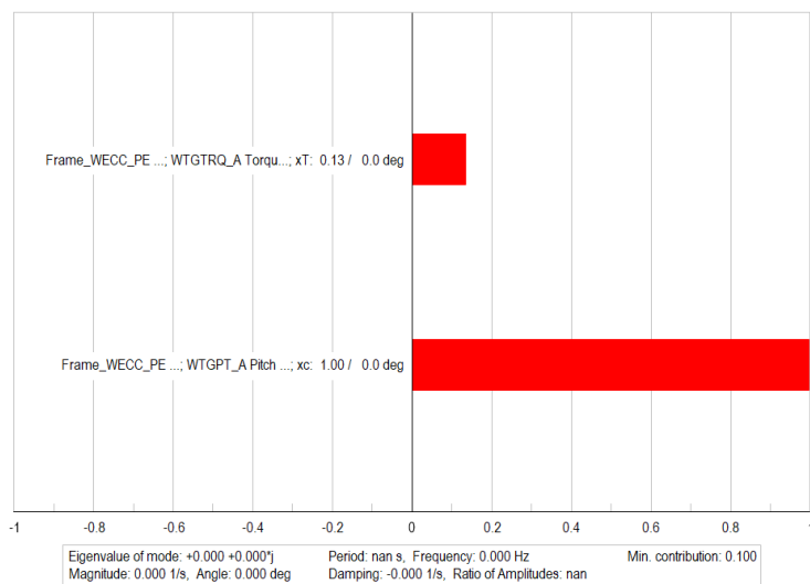
Mode 681: Participation
