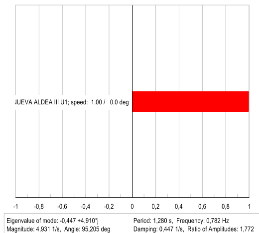
Mode 1537: Participation
