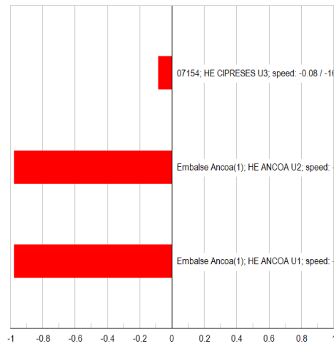
Mode 994: Participation
