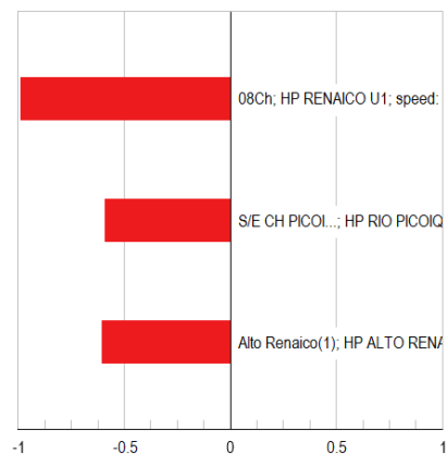
Mode 181: Participation
