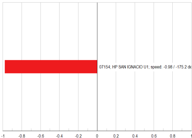
Mode 40: Participation
