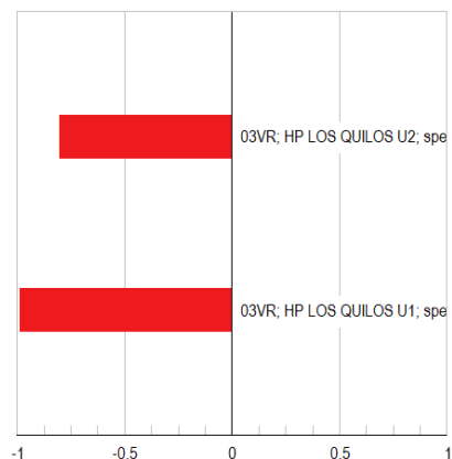
Mode 83: Participation
