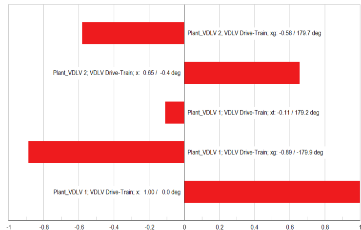
Mode 766: Participation
