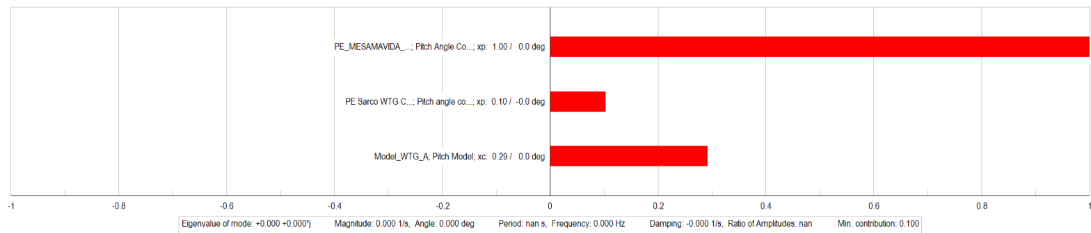
Mode 5: Participation
