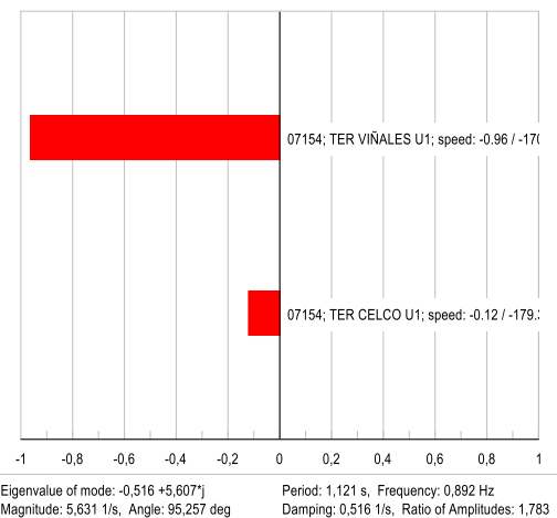
Mode 1657: Participation
