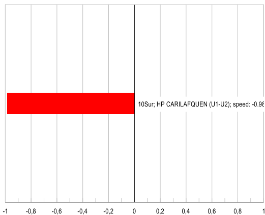
Mode 30: Participation
