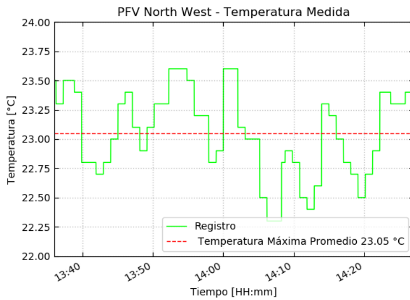
Figura 4-3 – Ensayo de Potencia Máxima – Datos Meteorológicos
