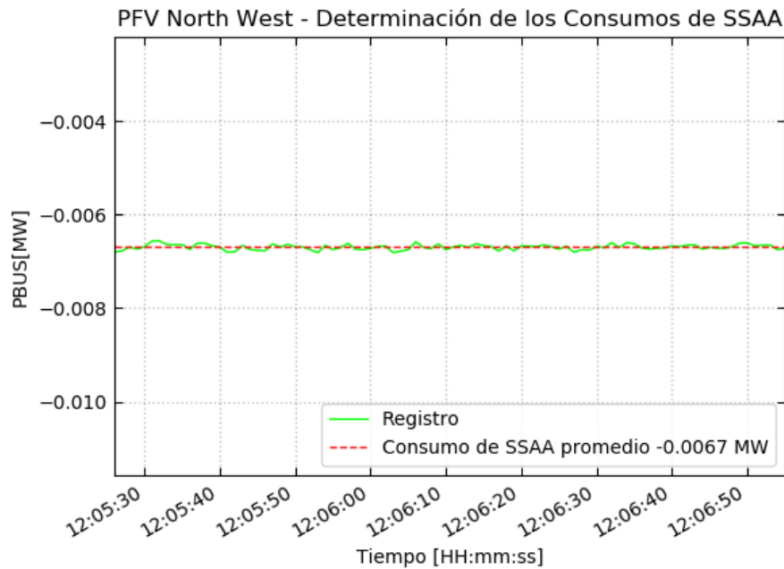
Figura 3-7 – Registro de Consumos de SSAA
