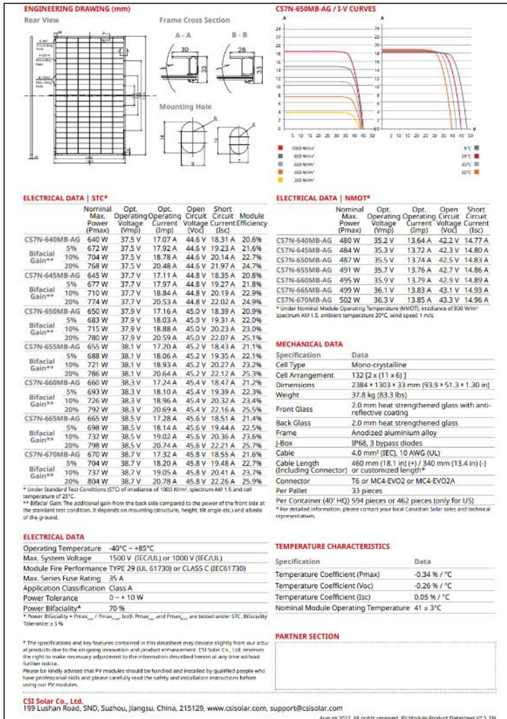
Figura 3-3 – Hoja de Datos – Panel Solar
