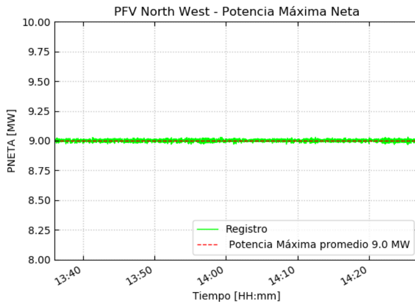
Figura 4-1 – Ensayo de Potencia Máxima – PNETA
