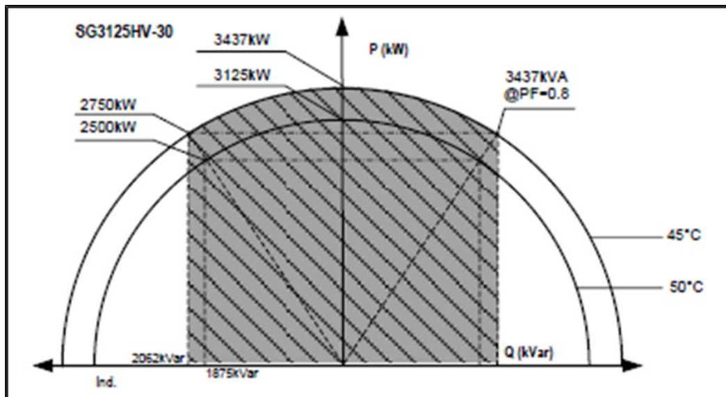
Figura 3-6 – Curva de capacidad del inversor PF mode
