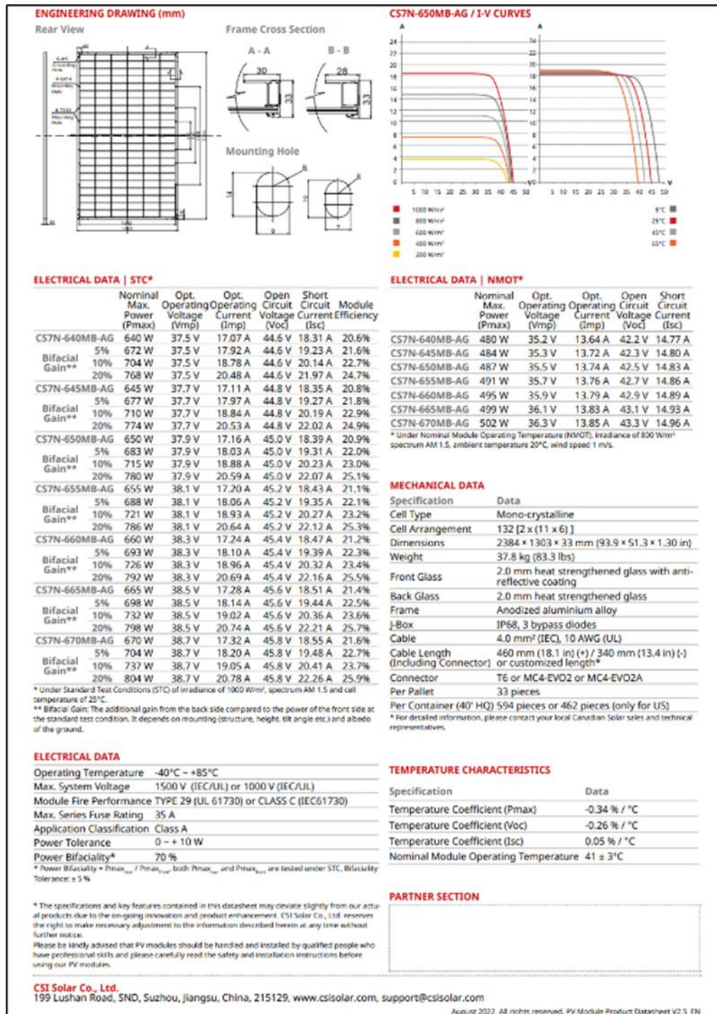
Figura 6-1 – Hoja de datos del panel solar – Valores nominales
