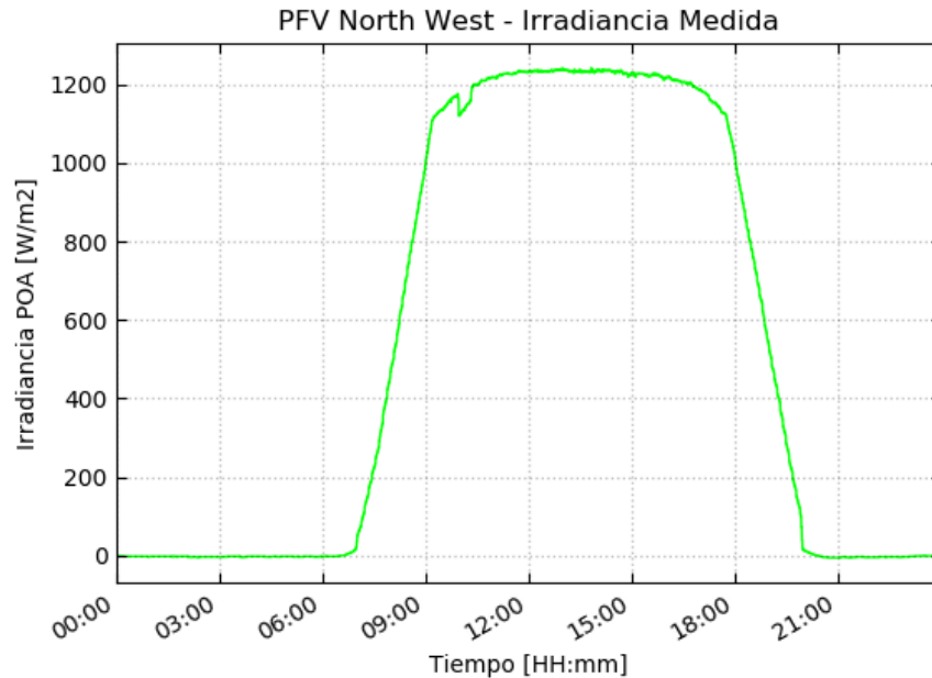
Figura 4-4 – Ensayo de Potencia Máxima – Irradiancia día 21/11/2023
