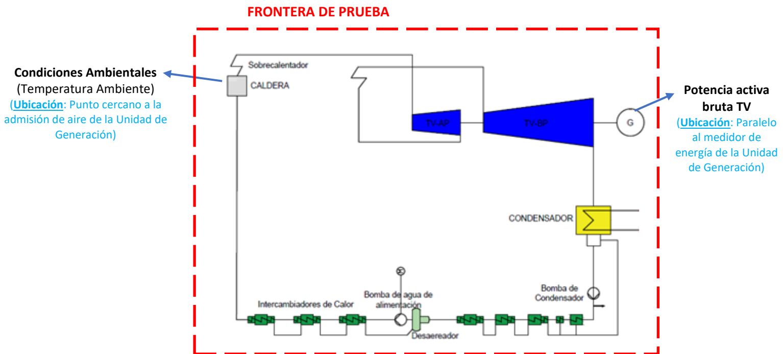
Figura 5-2: Ubicación de Puntos de Medición de la Unidad GEO Cerro Pabellón U1
