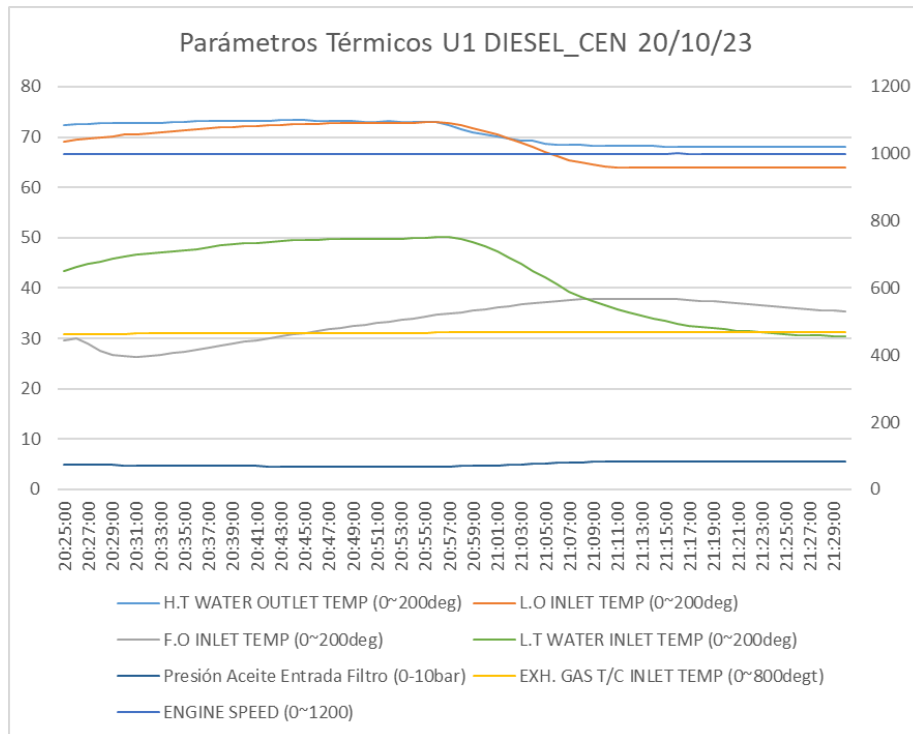
Ilustración 3 Parámetros Térmicos
