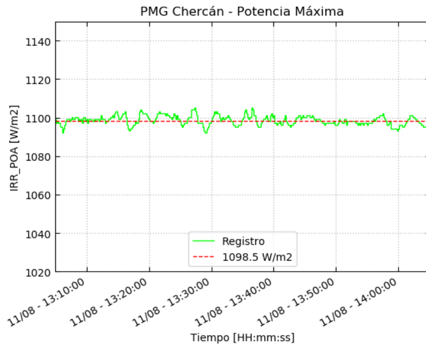
Figura 4.3 – Irradiancia POA – Potencia Máxima
