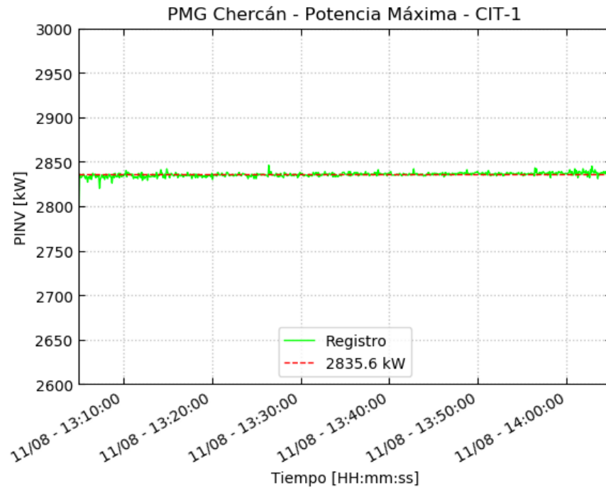
Figura 4.2 – Potencia CIT-1 – Potencia Máxima
