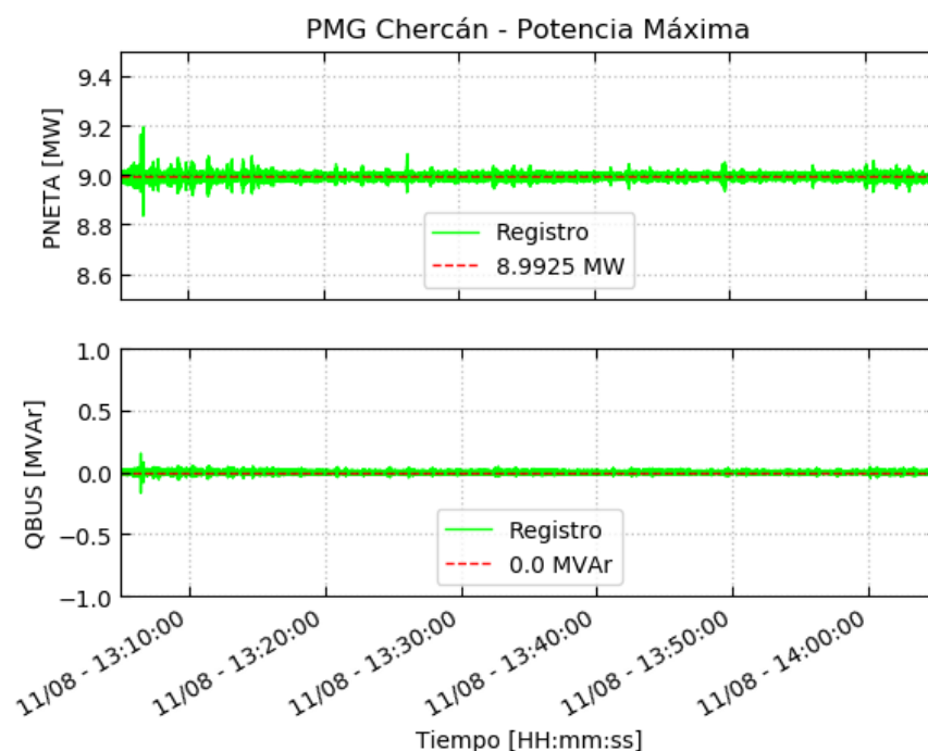
Figura 4.1 – Potencia neta – Potencia Máxima
