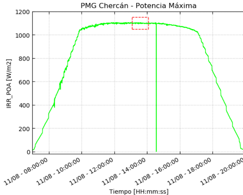
Figura 4.4 – Irradiancia POA día completo – Potencia Máxima
