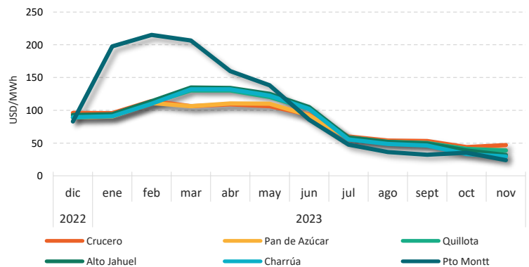
Evolución Costo Marginal Promedio Mensual - Últimos 12 meses
