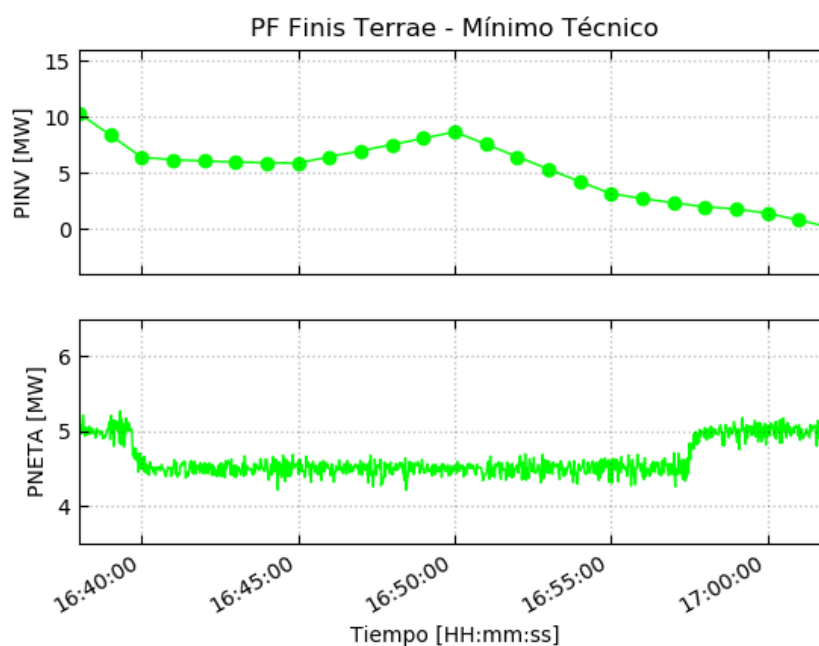
Figura 6.1 – Mínimo Técnico – Operación no estable de los inversores
