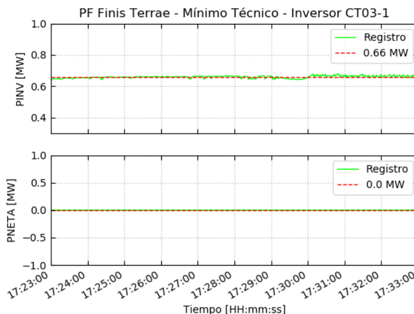
Figura 4.1 – Mínimo Técnico – Inversor CT03-1
