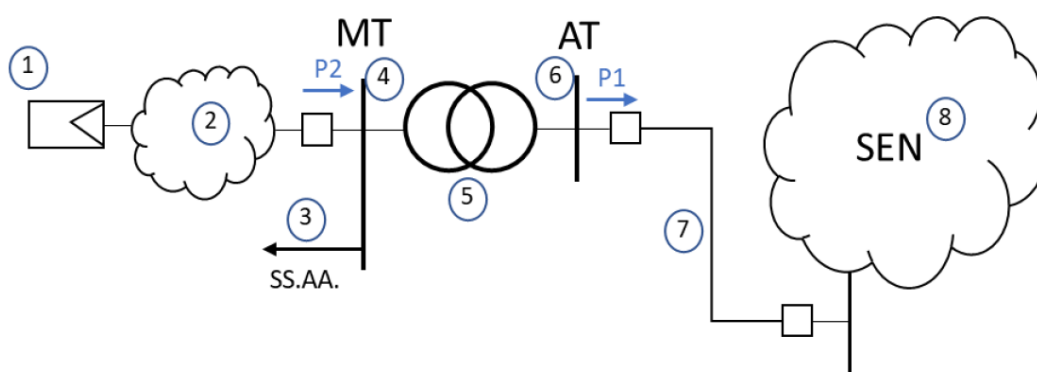
Figura 1.3 – Sistema equivalente parque fotovoltaico
