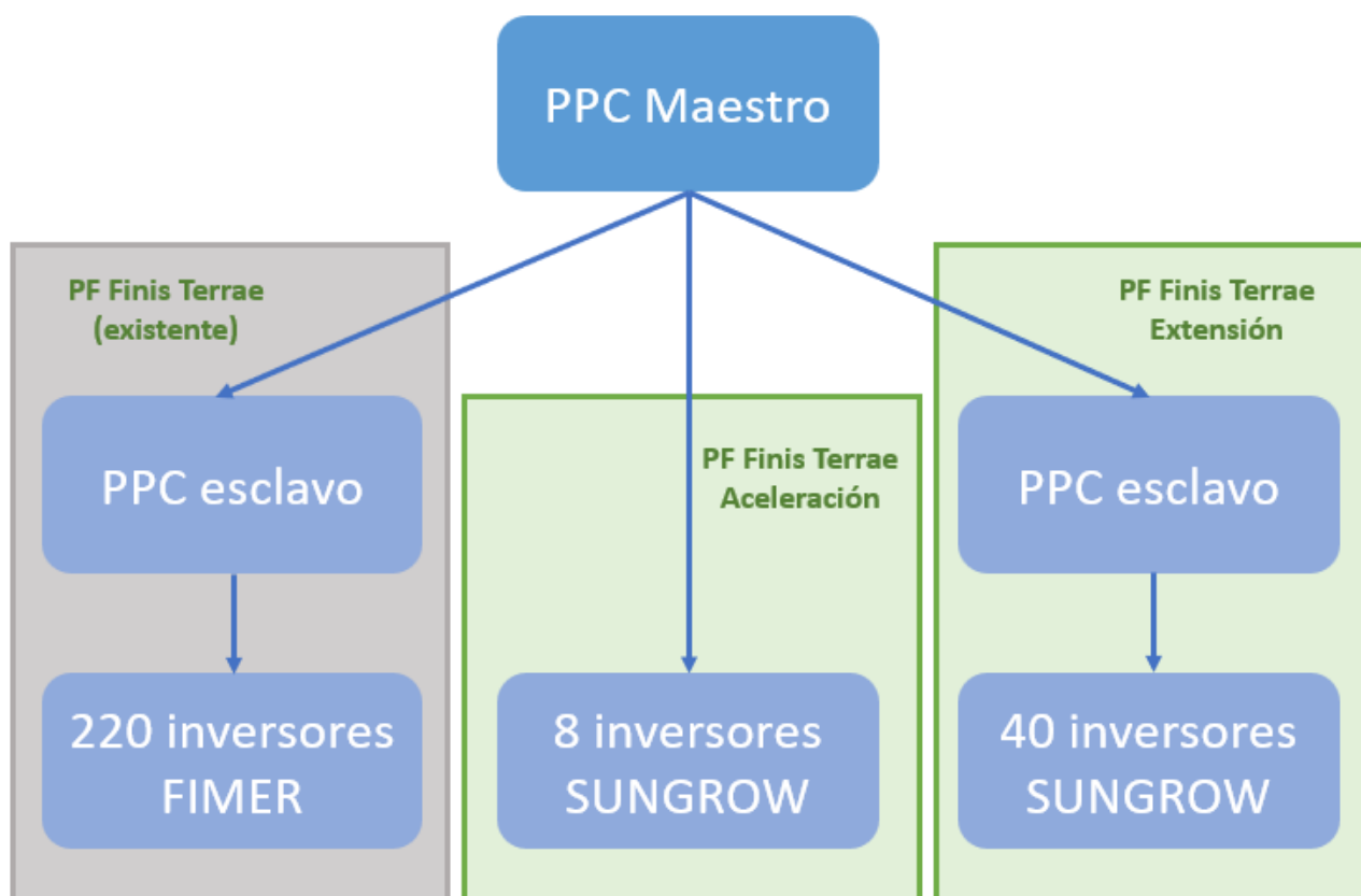
Figura 1.2 – Jerarquía del control conjunto de planta
