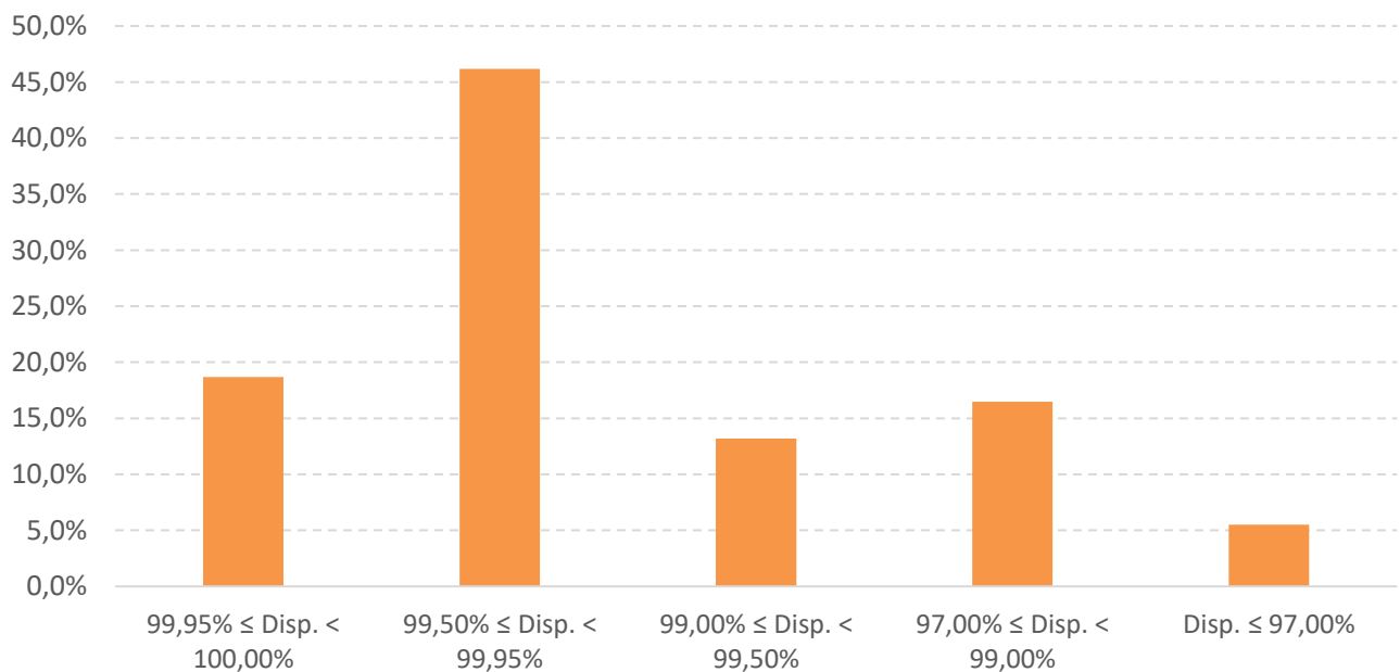
Figura 5: Cumplimiento de Disponibilidad de Canales de Teleprotección en 2022.
