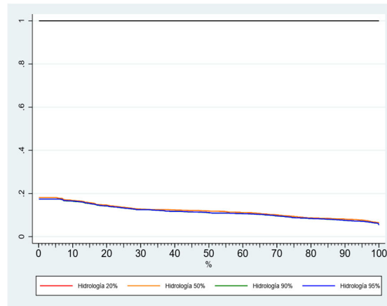
Figura 6-8: Curva duración RSI3 CPF- diferentes hidrologías ajustando disponibilidad por Caso 1 y Caso 2
