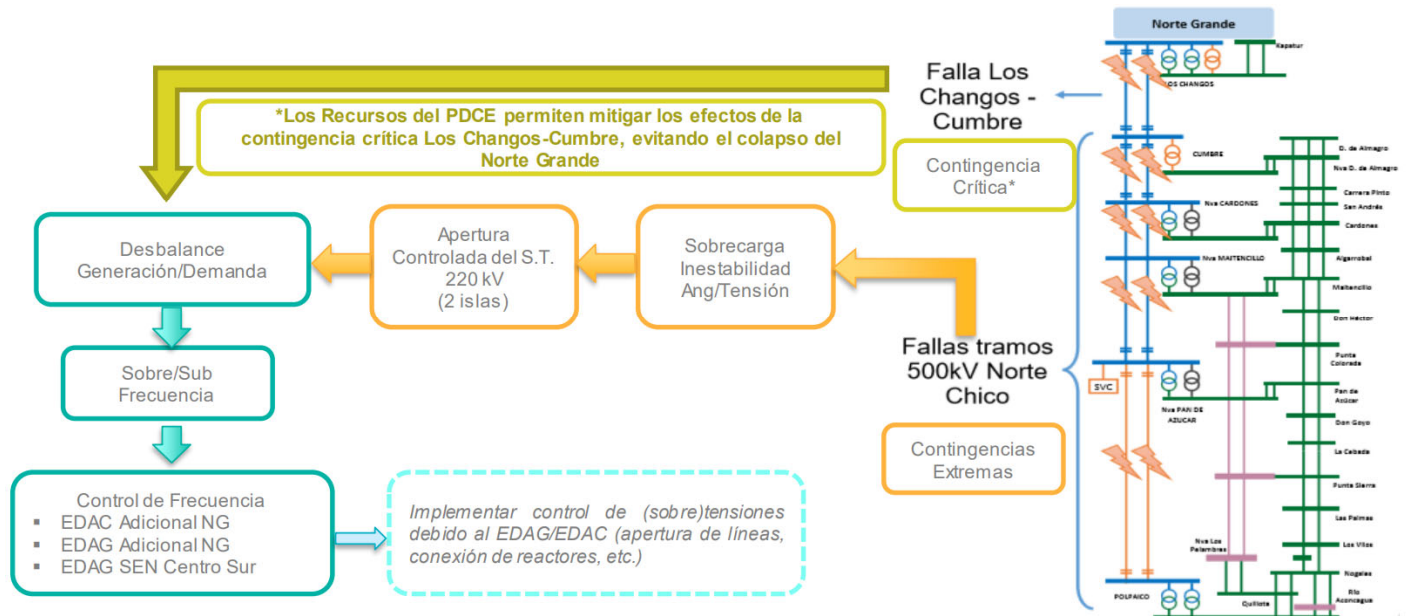
Figura 9-1: Descripción general del PDCE Zona Norte del SEN
