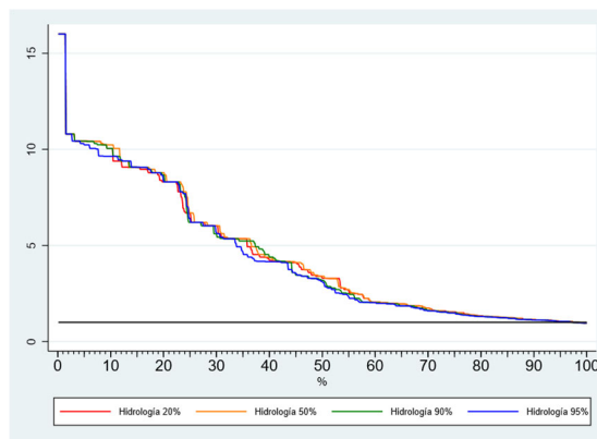
Figura 6-15: Curva duración RSI3 CTF+ diferentes hidrologías ajustando disponibilidad por Caso 1 y Caso 2
