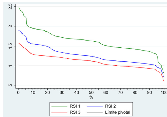
Figura 6-17: Curva duración RSI 1, 2 y 3 para CI
