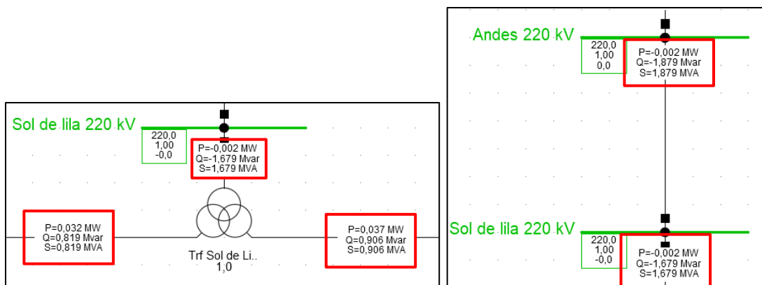
Figura 7-3 Pérdidas en el transformador de poder y línea de transmisión.
