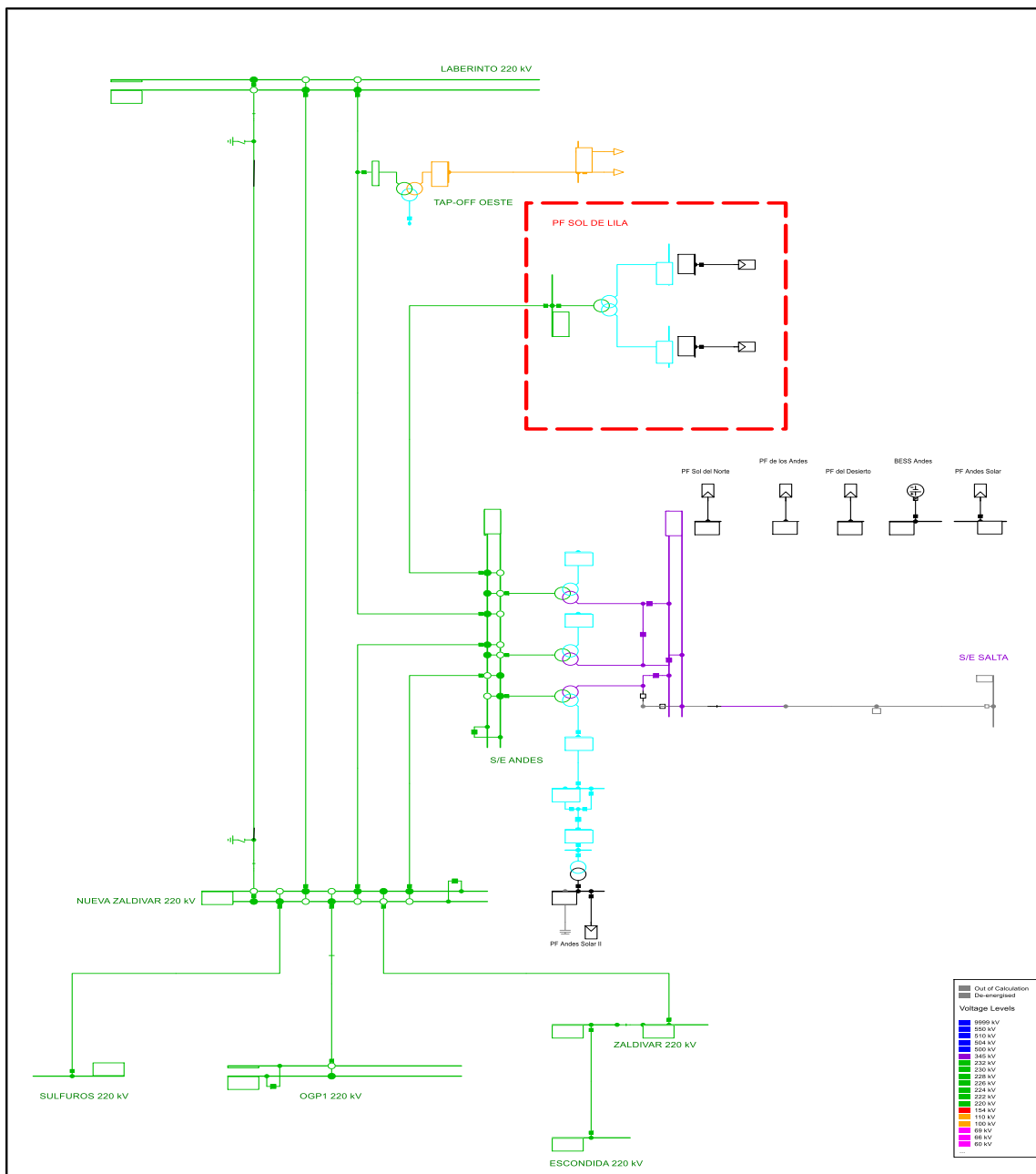
Figura 5-1 Diagrama unilineal de la zona de influencia. 1
