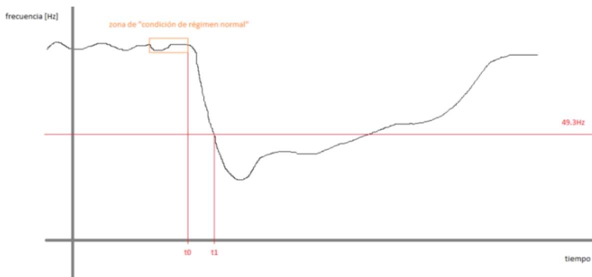
Figura 3. Señal de frecuencia, instantes " t_0 " y " t_1 "
