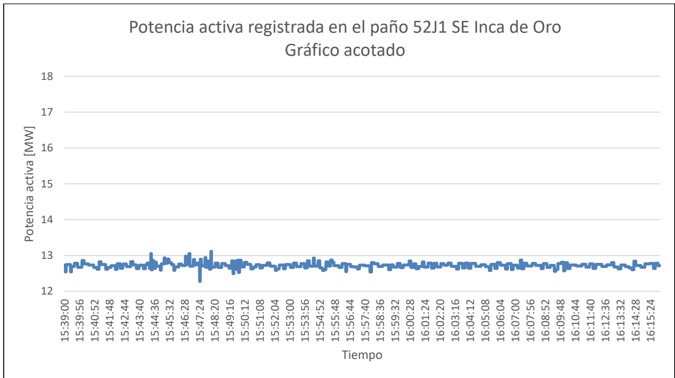
Figura 4.2: Registro de potencia a mínimo técnico [MW] en el paño 52J1 de la SE Inca de Oro, el día 02-06-2022. Gráfico acotado.
