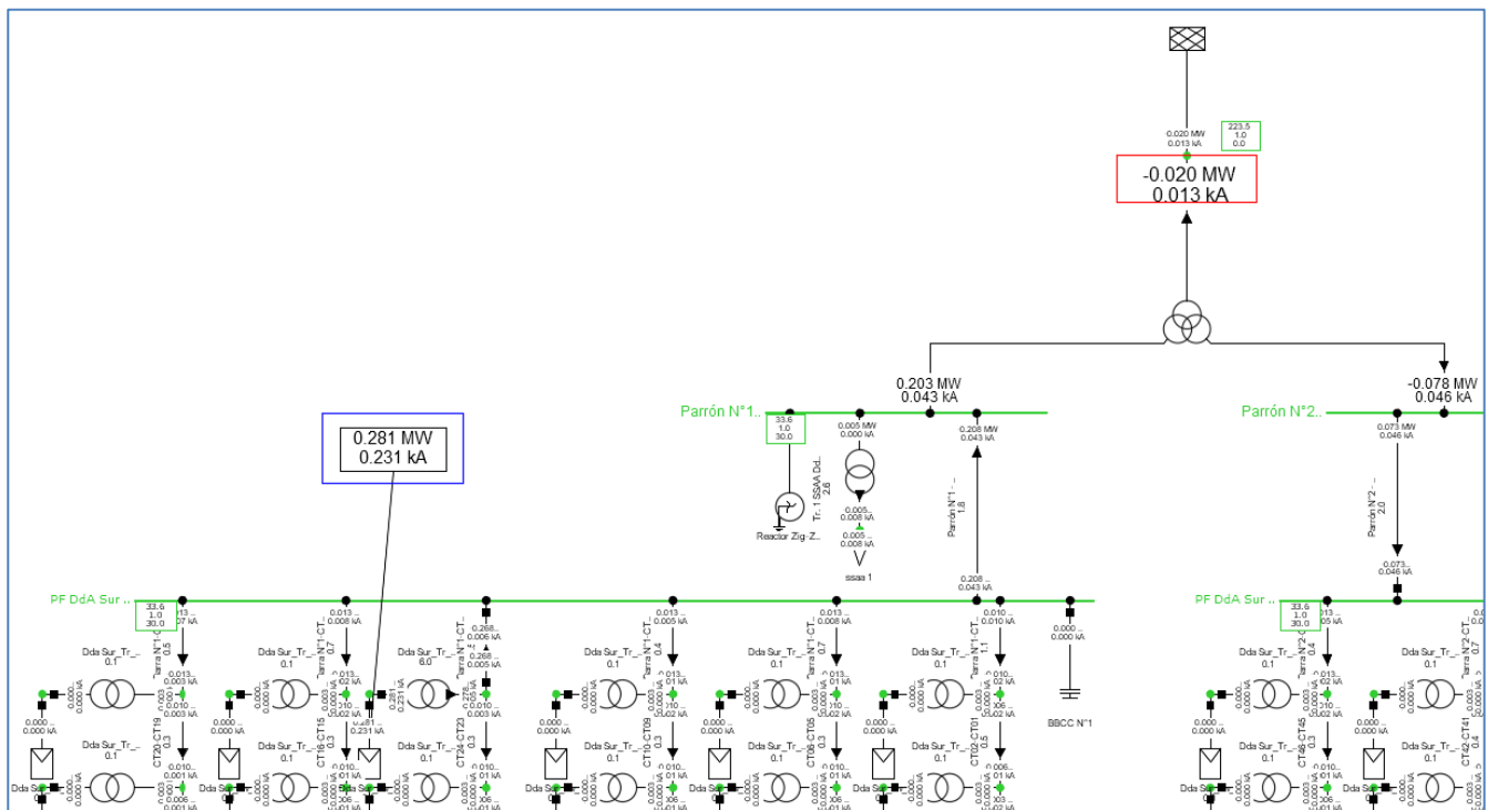
Figura 6.4: Generación de un solo inversor a mínimo técnico en PFV Diego de Almagro Sur.
