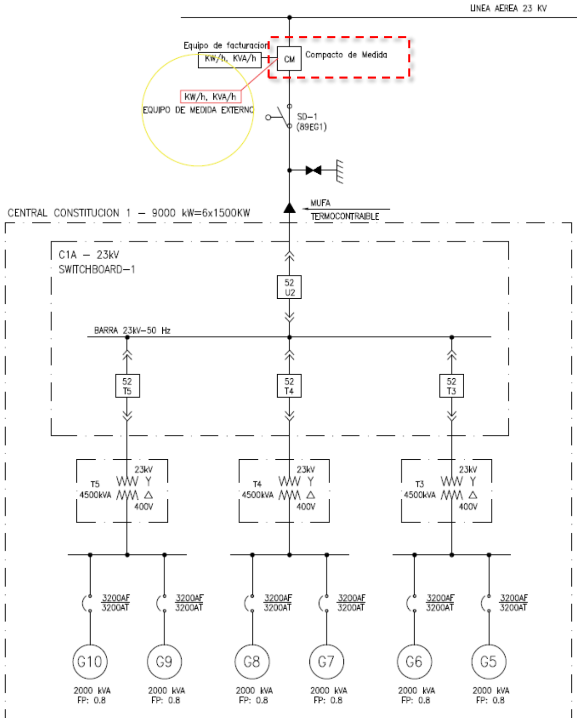
Figura 9-13 – Unilineal para mediciones de potencia neta
