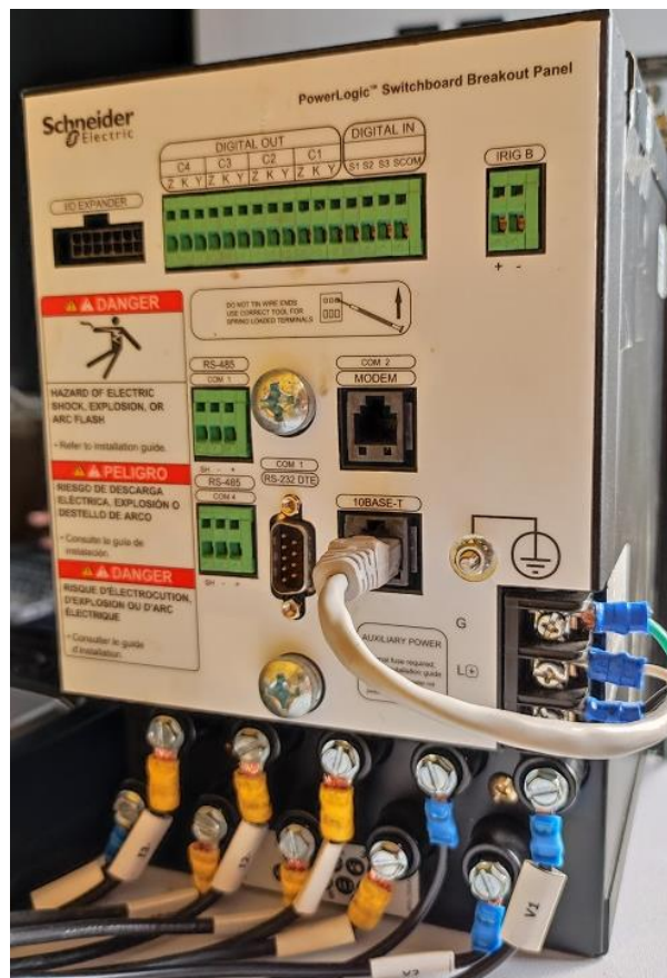
Figura 9-32 – Medidor de potencia bruta/FP unidad G5
