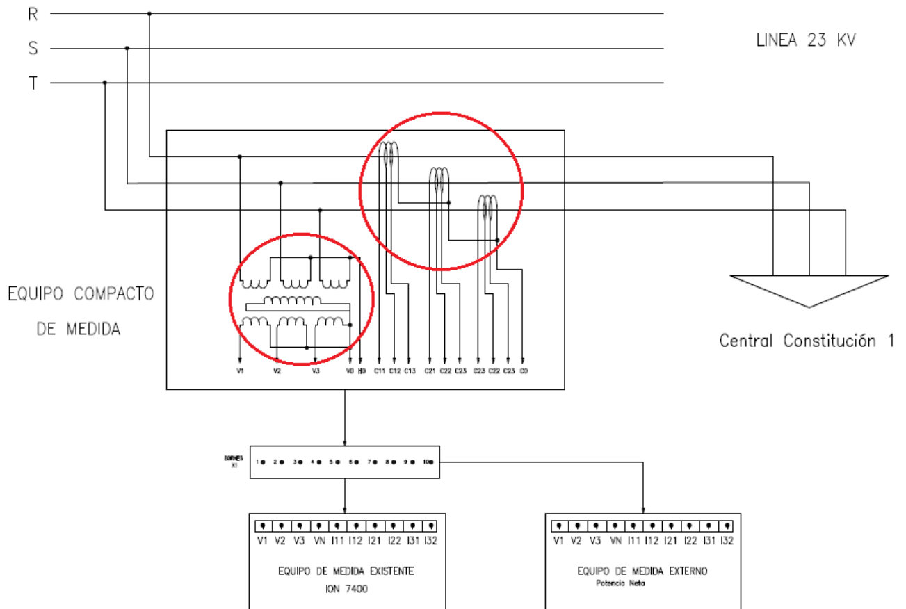
Figura 9-14 – Puntos de medición de tensión y corriente para medidor de Potencia neta y Factor de potencia
