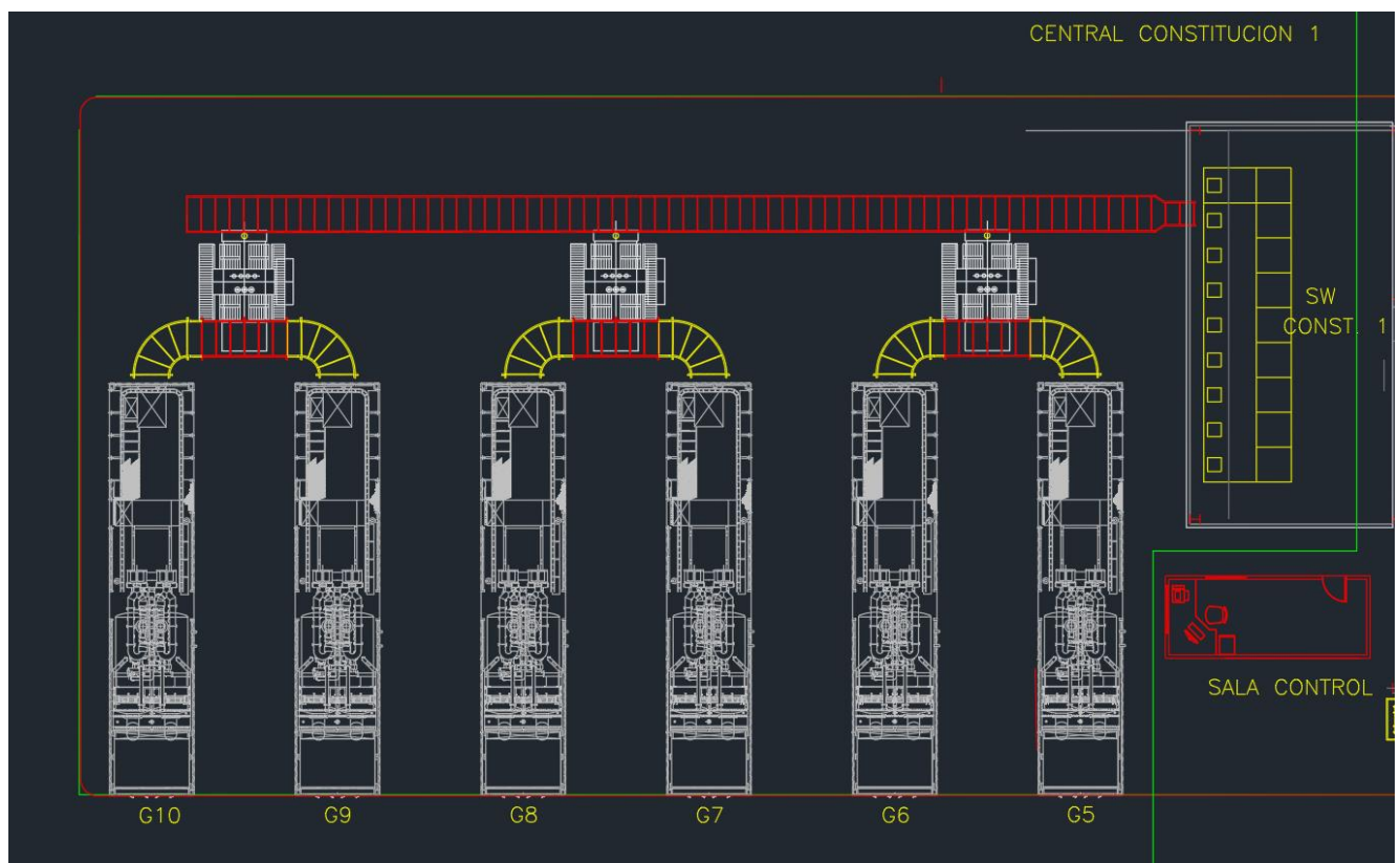
Figura 4-1 – Plano de disposición general de planta
