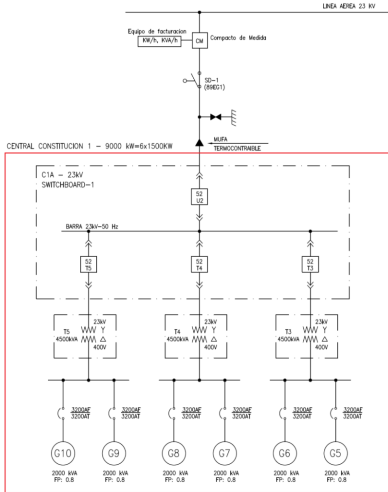
Figura 4-2 – Diagrama unilínea de la Central
