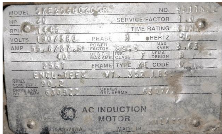
Figura 9-5 – Placa del motor del ventilador
