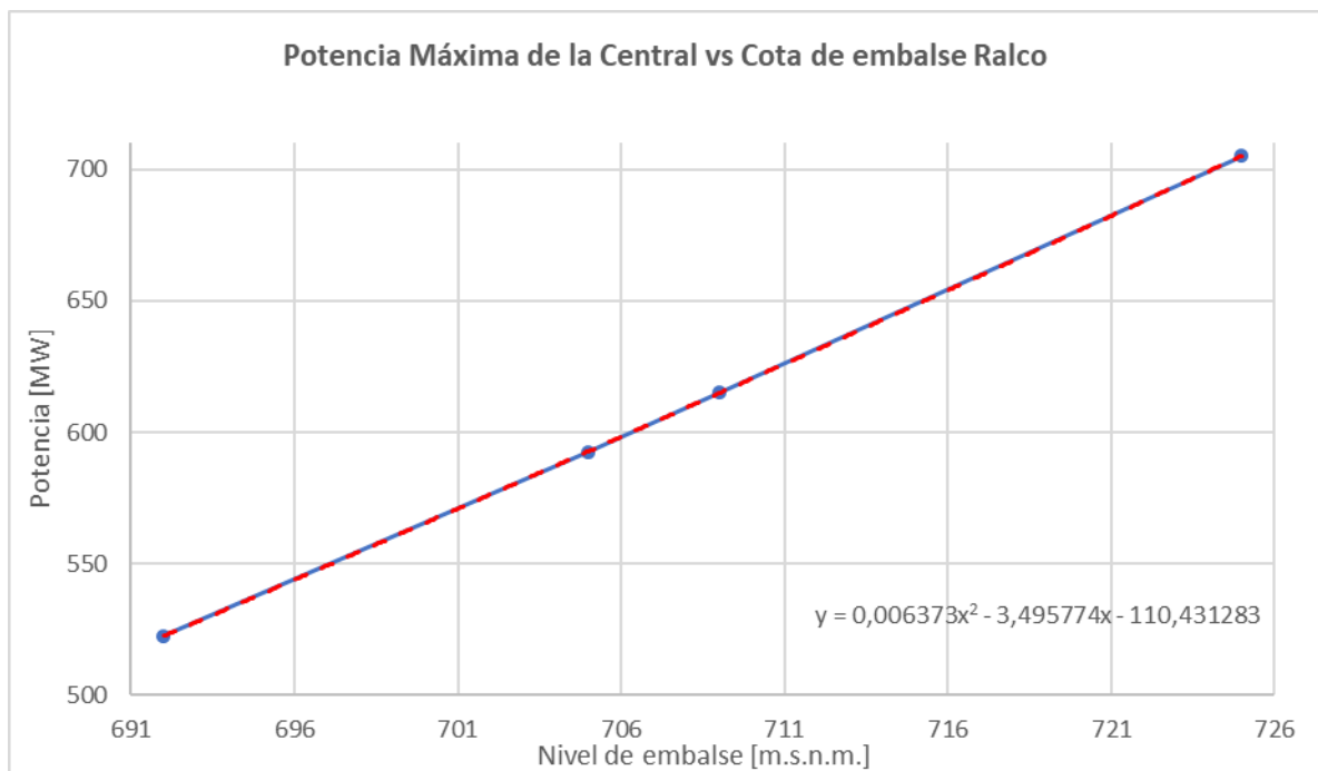
Figura 9-4 - Potencia máxima vs cota embalse Ralco - CH Ralco
