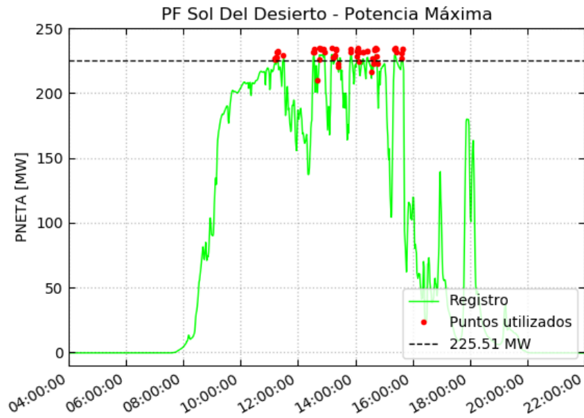
Figura 4.3 – Potencia Máxima – Potencia neta del día completo
