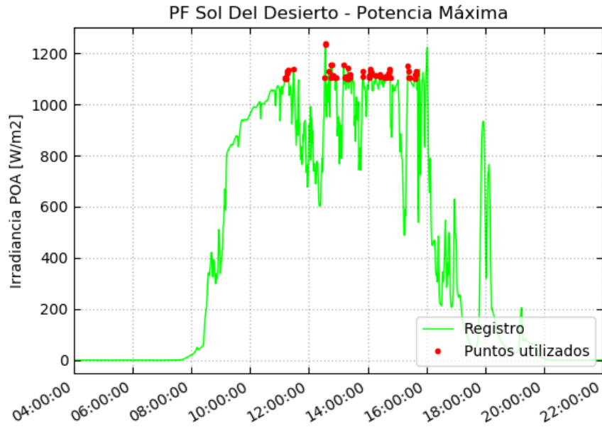
Figura 4.1 – Potencia Máxima – Irradiancia del día completo
