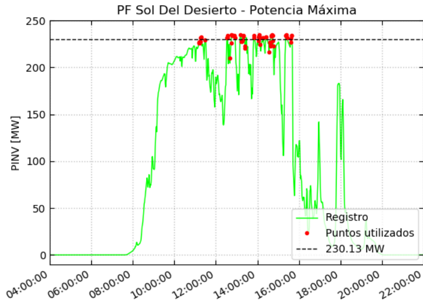
Figura 4.2 – Potencia Máxima – Potencia de inversores del día completo
