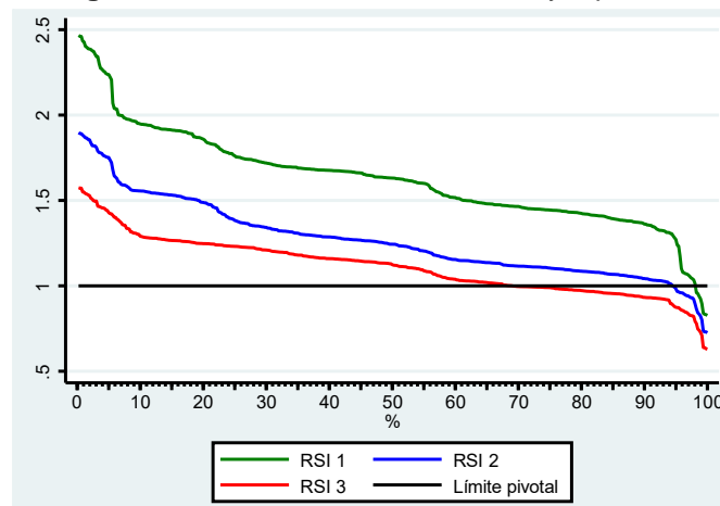
Figura 6-17: Curva duración RSI 1, 2 y 3 para CI
