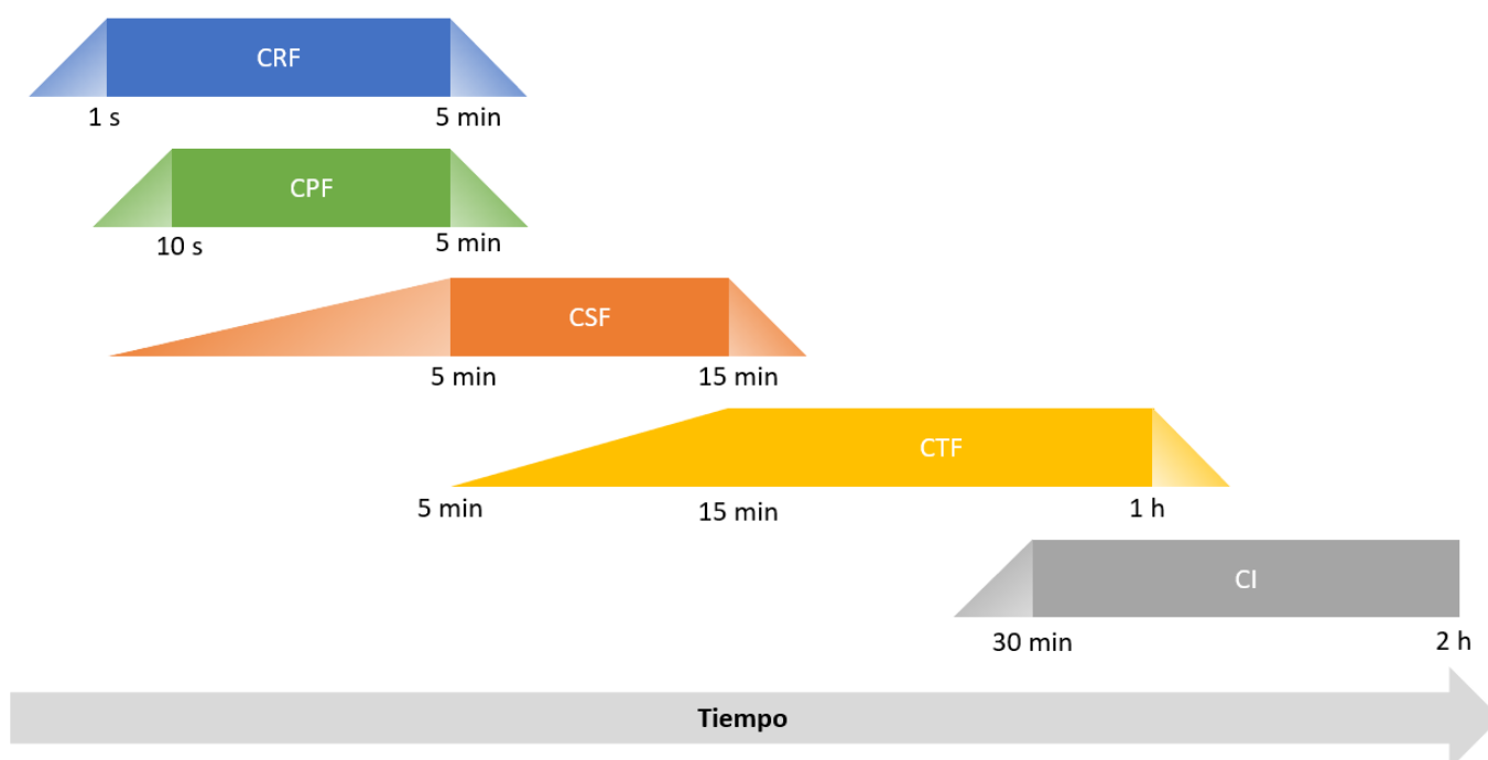
Figura 4-1: Esquema cadena de reservas de Control de Frecuencia.
