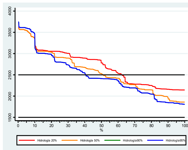
Figura 6-1: Curva duración HHI CPF+ para diferentes hidrologías
