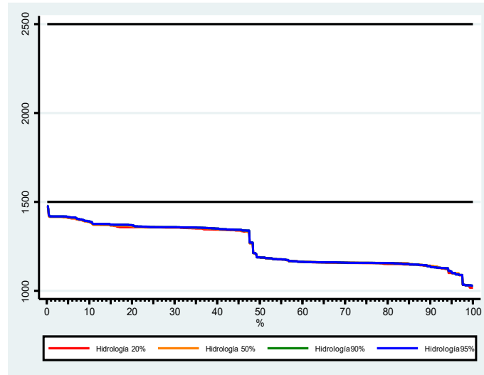
Figura 6-2: Curva duración HHI CPF- para diferentes hidrologías
