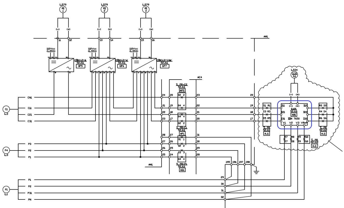
Figura 9-6 – Puntos de medición de corriente y tensión para la medición de potencia neta
