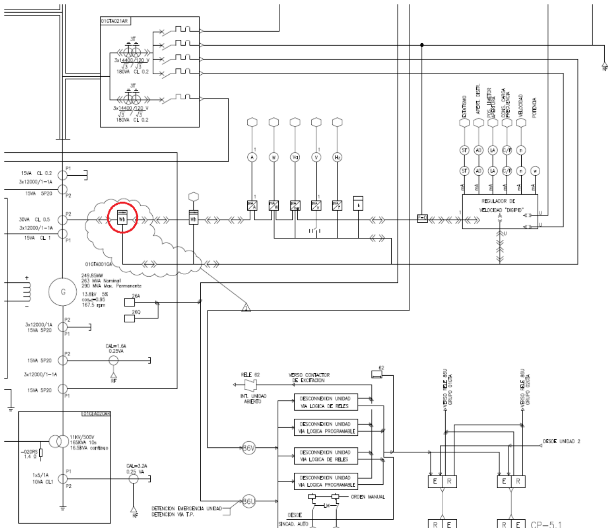
Figura 9-4 - Unilineal para la medición de Potencia Bruta y Factor de Potencia
