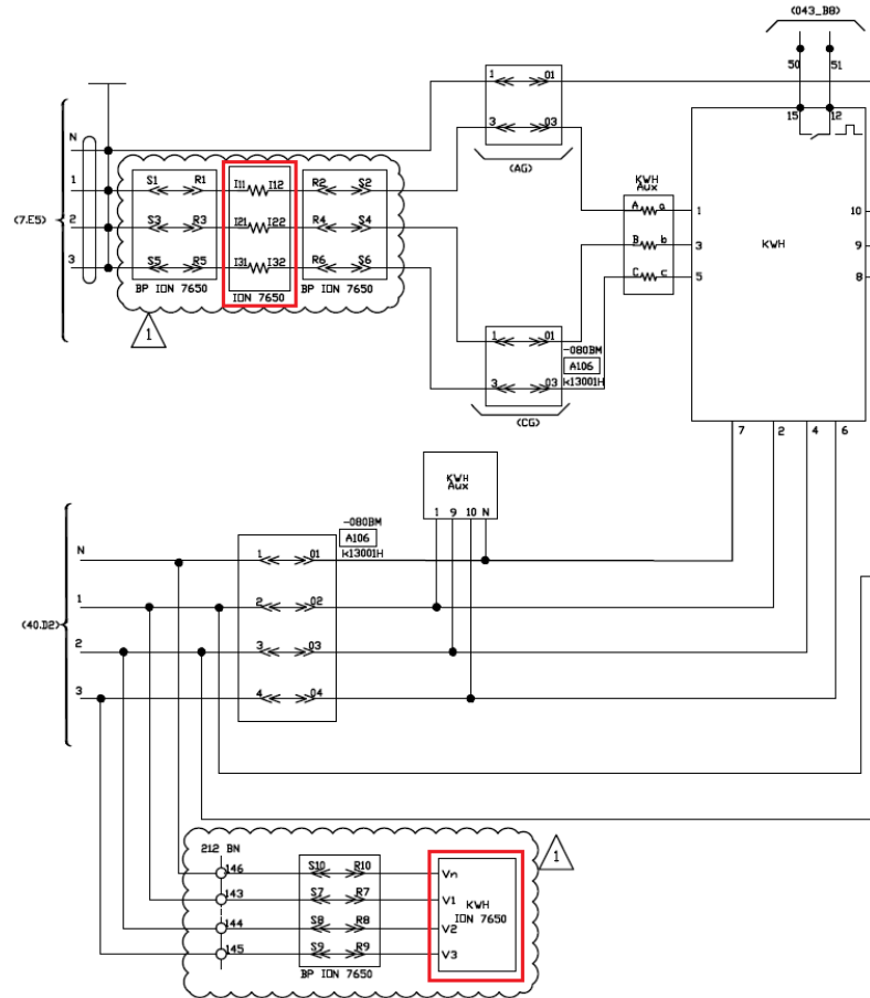
Figura 9-5 – Puntos de medición de corriente y tensión para la medición de Potencia Bruta y Factor de Potencia
