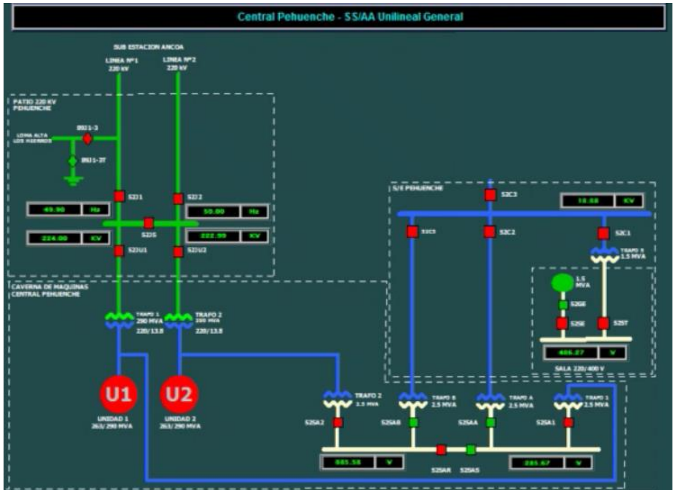
Figura 5-3 - Condiciones operativas durante los ensayos de la Central completa
