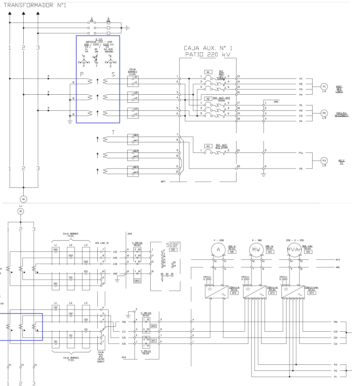
Figura 9-7 – Puntos de medición de corriente y tensión para la medición de potencia neta
