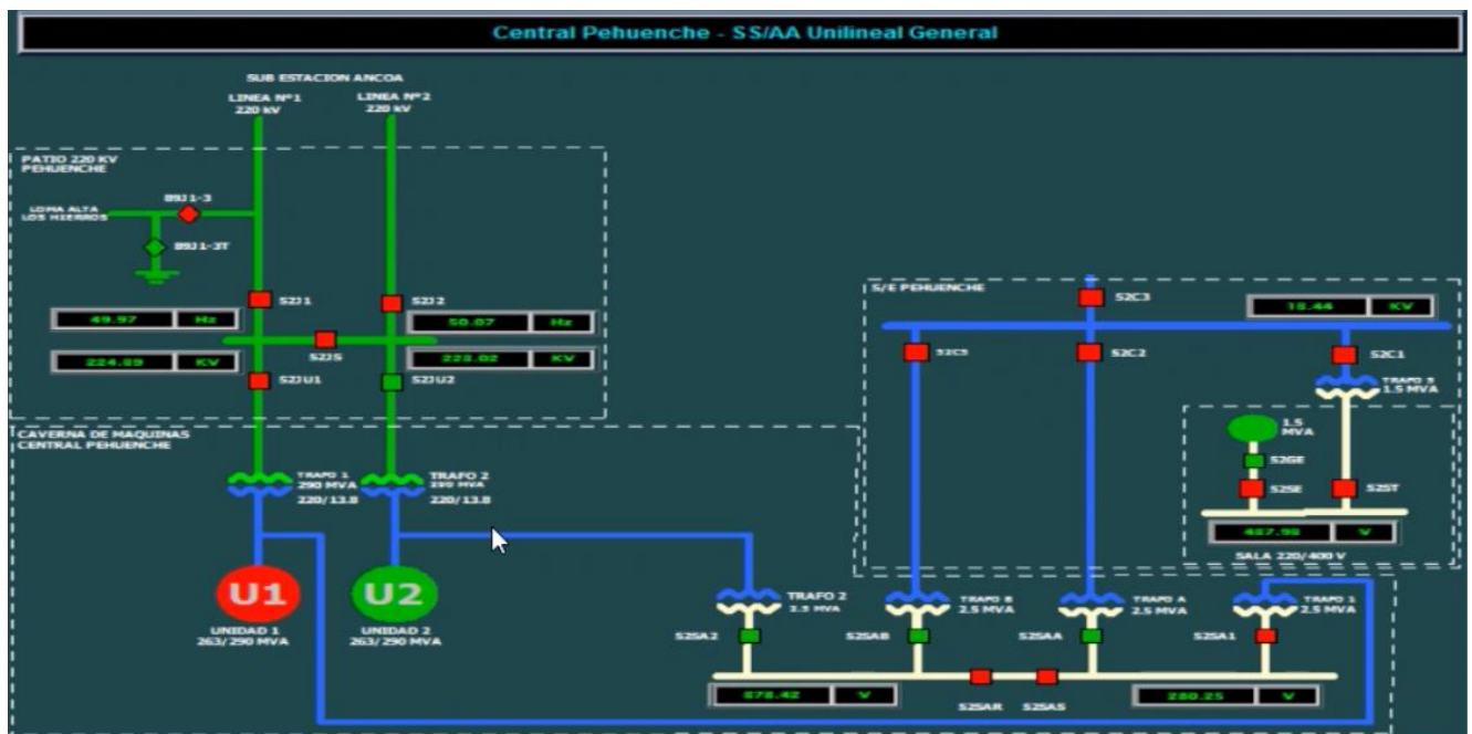
Figura 5-1 - Condiciones operativas durante los ensayos de la Unidad 1
