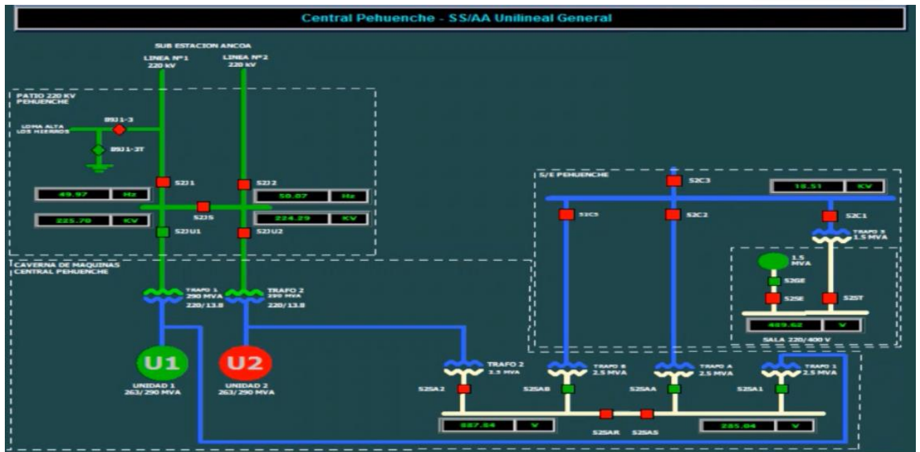
Figura 5-2 - Condiciones operativas durante los ensayos de la Unidad 2
