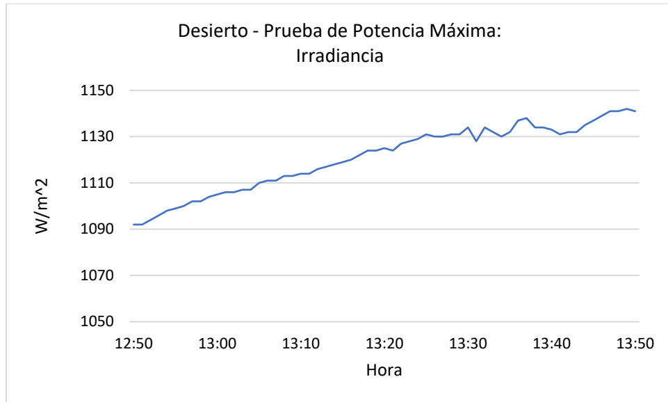
Figura 10: Irradiancia en central Desierto durante la prueba de potencia máxima.
