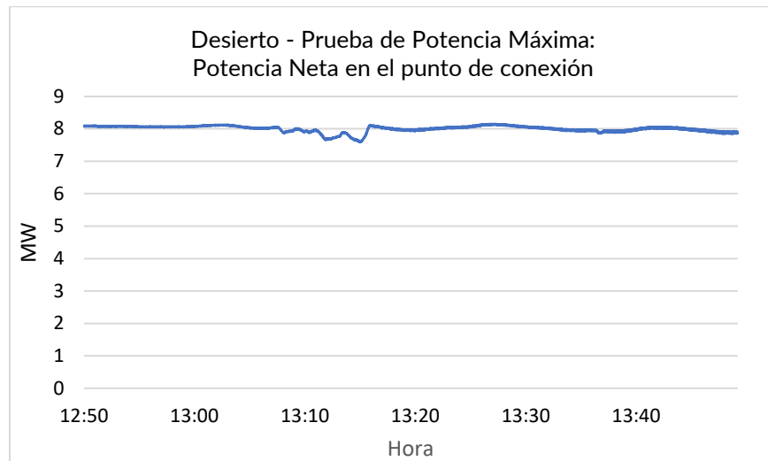
Figura 8: Potencia inyectada por central Desierto durante la prueba de potencia máxima.
