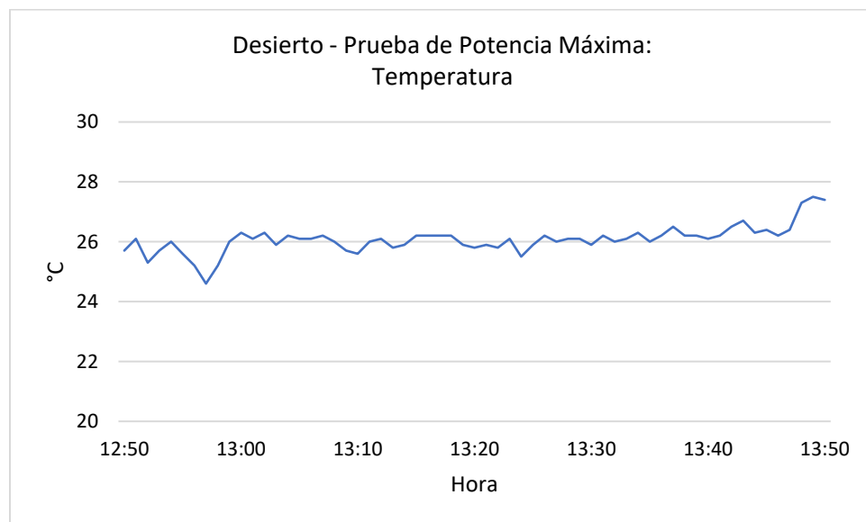
Figura 9: Temperatura ambiente en central Desierto durante la prueba de potencia máxima.
