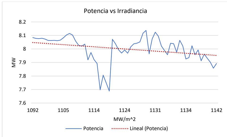
Figura 12: Potencia vs Irradiancia durante la prueba de potencia máxima en central Desierto.
