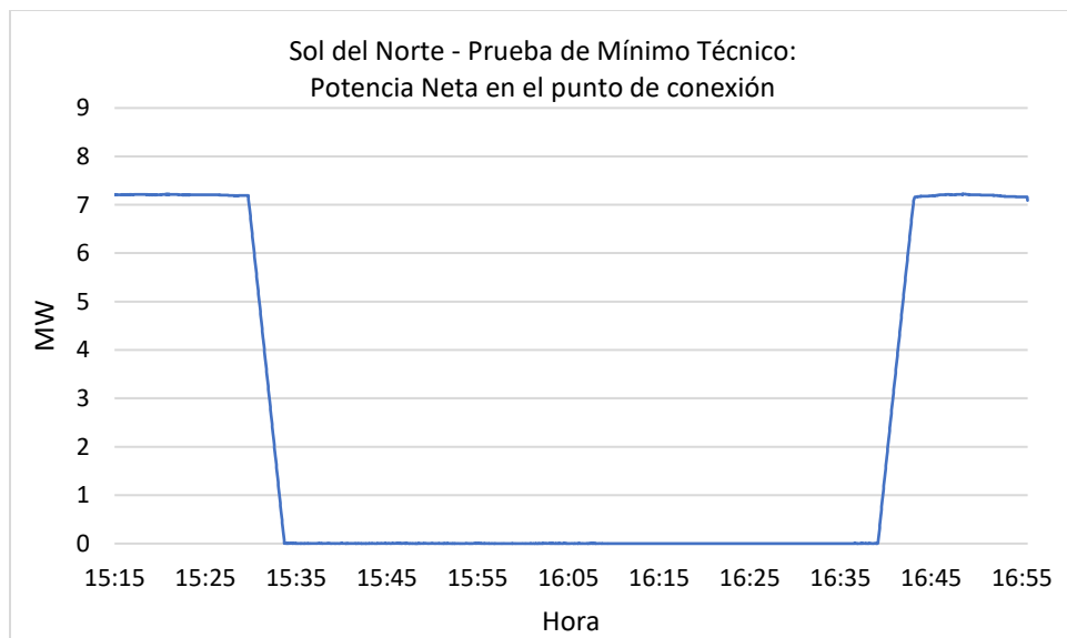
Figura 8: Potencia inyectada por central Sol del Norte durante la prueba de mínimo técnico.
