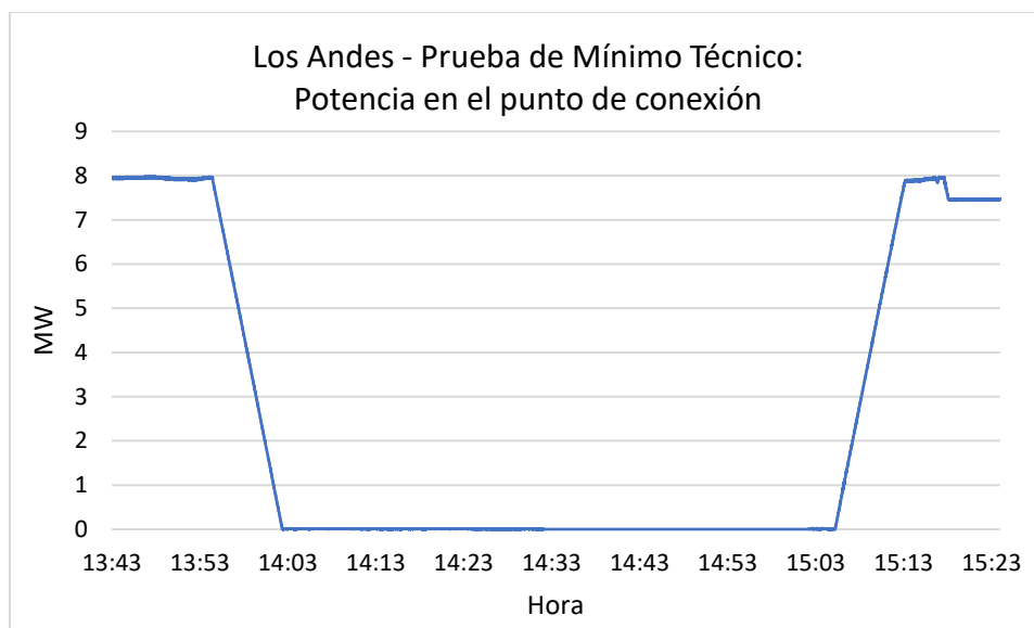
Figura 8: Potencia inyectada por central Los Andes durante la prueba de mínimo técnico.
