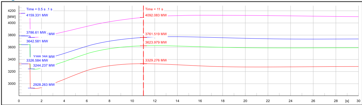
Figura 6: Potencia de Turbina del SEN. Caso 0 (Magenta) 30 [GVAs], Caso 1 (Azul) 27,5 [GVAs], Caso 2 (Verde) 25 [GVAs], Caso 3 (Rojo) 22,5 [GVAs].
