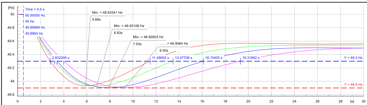
Figura 5: Frecuencia Eléctrica SEN. Caso 0 (Magenta) 30 [GVAs], Caso 1 (Azul) 27,5 [GVAs], Caso 2 (Verde) 25 [GVAs], Caso 3 (Rojo) 22,5 [GVAs].
