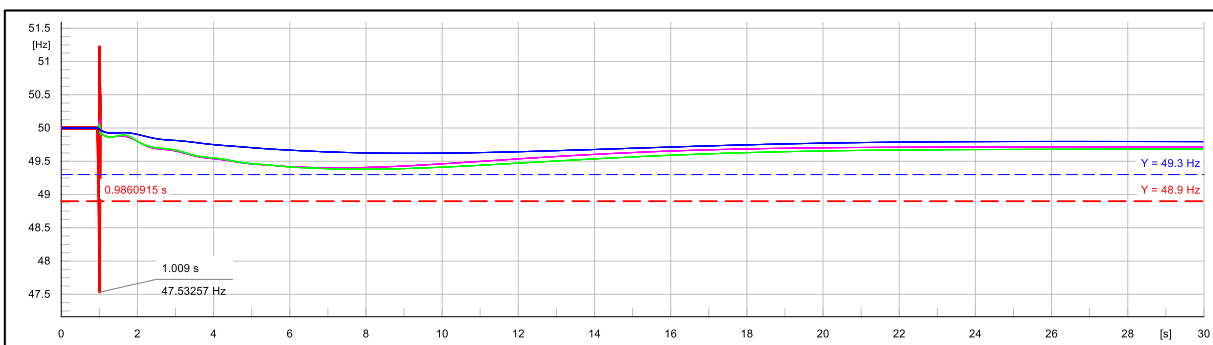
Figura 8: Frecuencia Eléctrica Principales Barras Norte del SEN. Severidad 5 CCH1, Caso 3 (Rojo) 22,5 [GVAs], Caso 2 (Verde) 25 [GVAs], Caso 1 (Azul) 27,5 [GVAs], Caso 0 (Magenta) 30 [GVAs].
