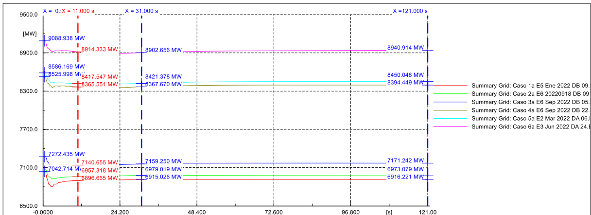
Figura 1: Respuesta Carga Total del SEN para Distintos Casos. Contingencias de Generación.
