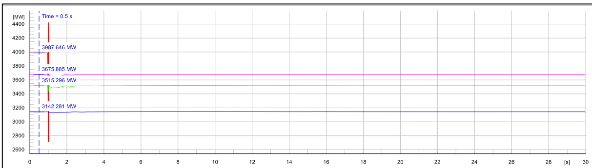
Figura 10: Generación ERV Total del SEN. Contingencia severidad 5 CCH1, Caso A2 (Azul) 25 [GVAs], Caso A3 (Verde) 27,5 [GVAs], Caso A4 (Magenta) 30 [GVAs].
