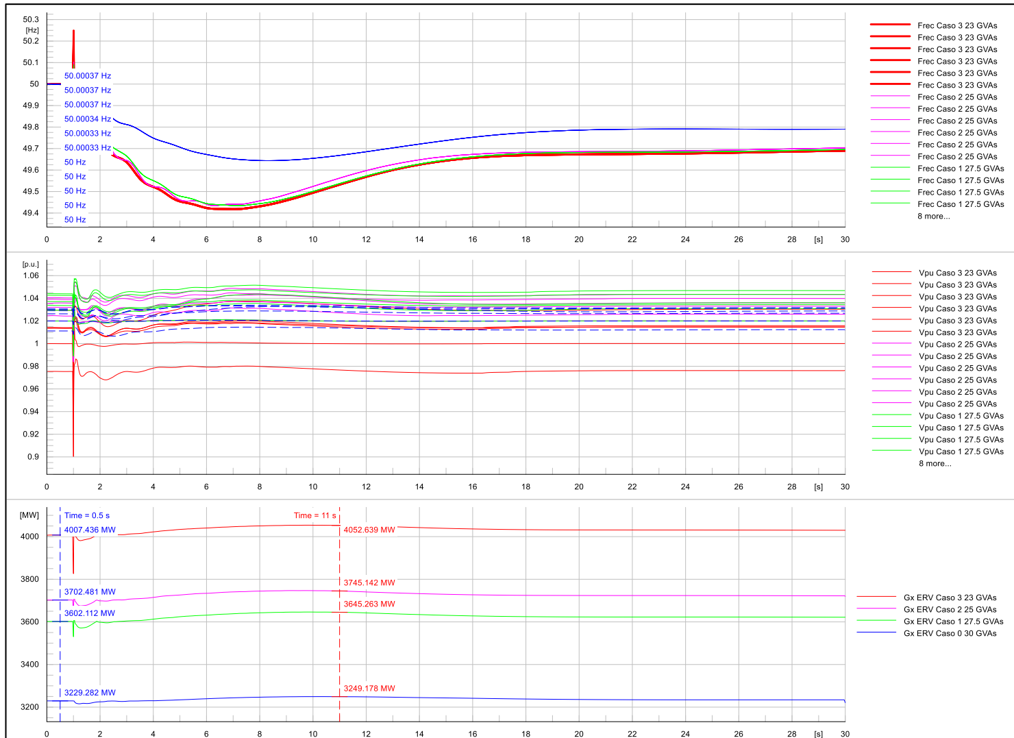
Figura 12: Verificación Norte Grande (Severidad 5 CCH) Condición 2: Plantas ERV participantes en CPF. ante contingencias de Generación.
