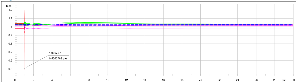
Figura 9: Tensiones Principales Barras Norte del SEN. Caso 3 (Rojo) 22,5 [GVAs], Caso 2 (Verde) 25 [GVAs], Caso 1 (Azul) 27,5 [GVAs], Caso 0 (Magenta) 30 [GVAs].
