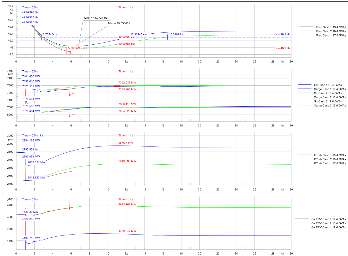
Figura 13: Resultados Condición 3: Participación de Plantas ERV en el CPF ante contingencias de Generación. Contingencia Severidad 5 IEM con 350 MW
