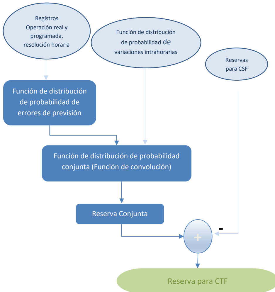
Figura 4: Metodología para la determinación de la reserva para CTF
