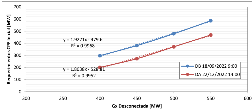
Figura 16: Requerimientos de CPF Inicial vs Gx Desconectada. Escenarios DA 22-12-2022 y DB 18-09-2022.
