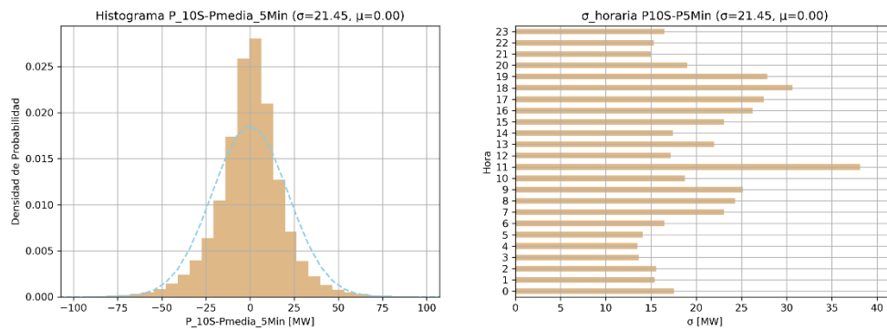
Figura 2: Densidad de probabilidad y desviaciones estándar de las fluctuaciones instantáneas.
