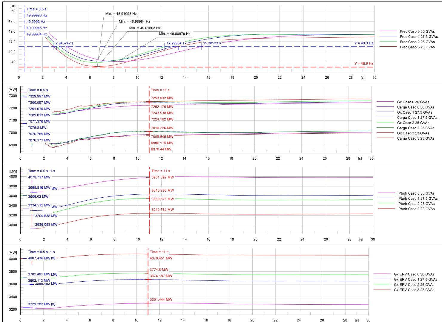
Figura 11: Resultados Condición 2: Plantas ERV participantes en CPF ante contingencias de Generación.
