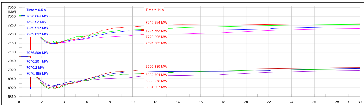
Figura 7: Generación y Carga Total del SEN. Caso 0 (Magenta) 30 [GVAs], Caso 1 (Azul) 27,5 [GVAs], Caso 2 (Verde) 25 [GVAs], Caso 3 (Rojo) 22,5 [GVAs].
