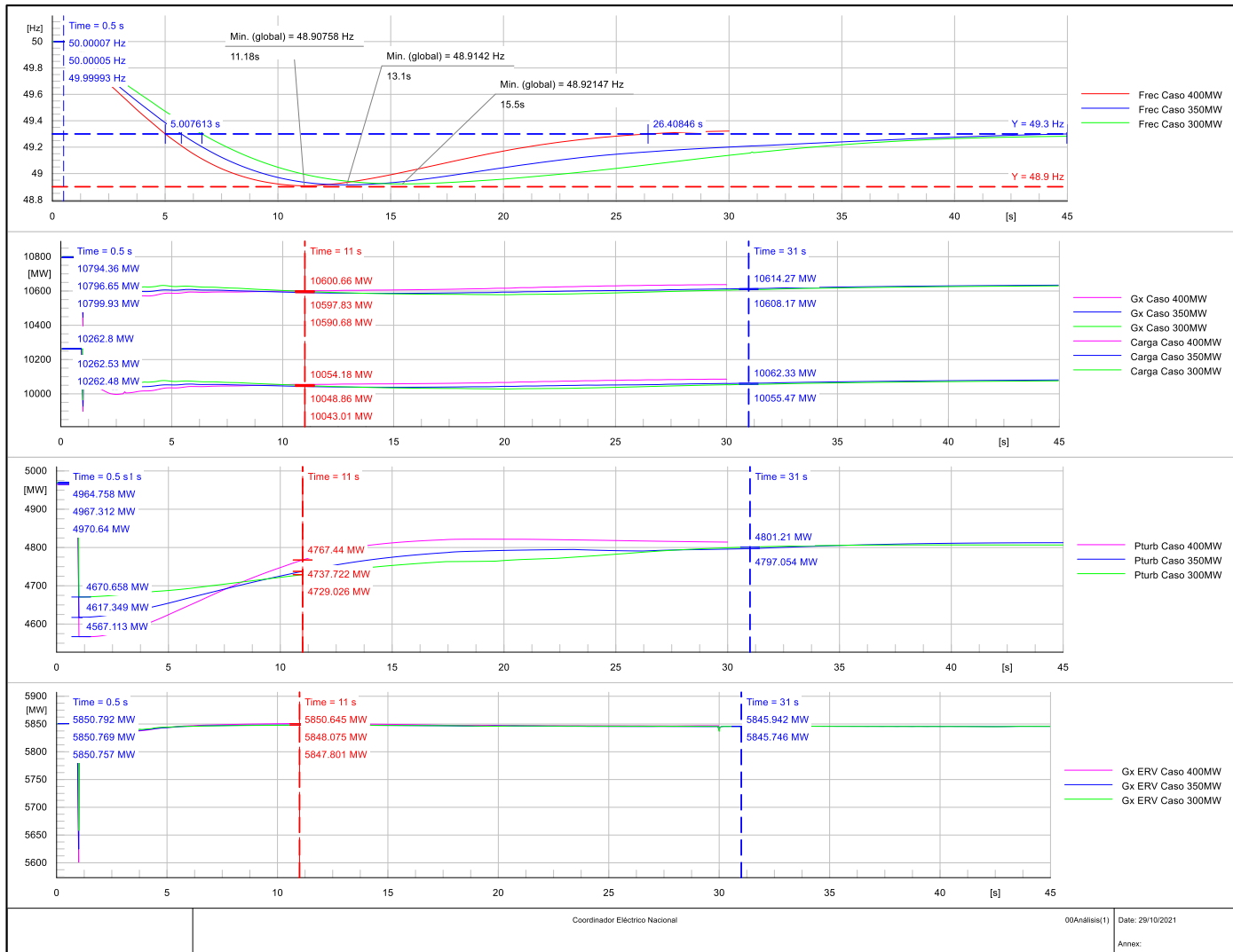
Figura 18: Resultados Análisis Requerimientos de CPF ante Montos Mayores de Desconexión. Caso DA 22-12-2022.
