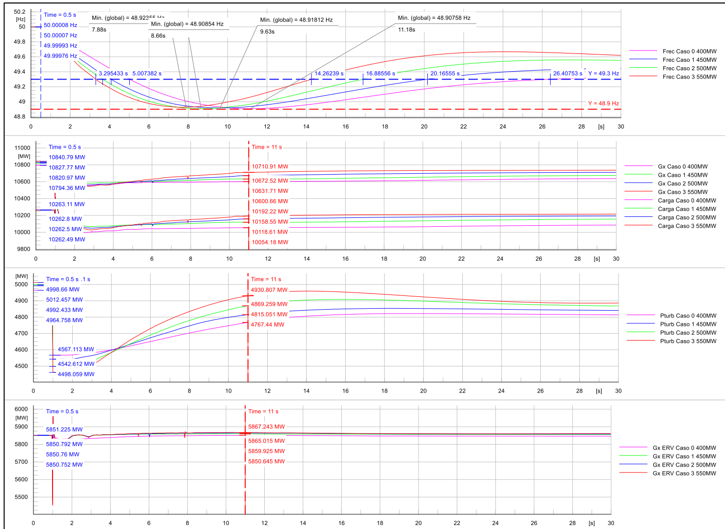
Figura 15: Resultados Análisis Requerimientos de CPF ante Montos Mayores de Desconexión. Caso DA 22-12-2022.
