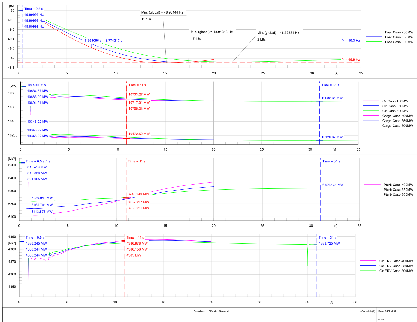
Figura 19: Resultados Análisis Requerimientos de CPF ante Montos Mayores de Desconexión. Caso DA 22-12-2022.
