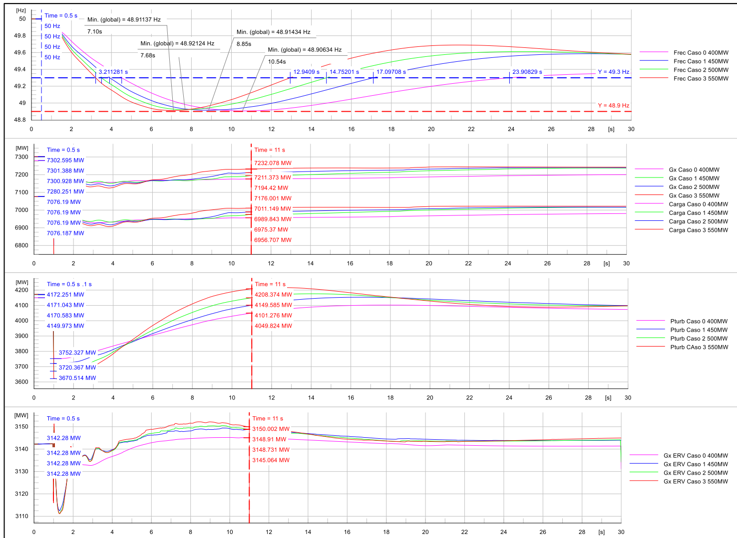
Figura 14: Resultados Análisis Requerimientos de CPF ante Montos Mayores de Desconexión. Caso DB 18-09-2022.
