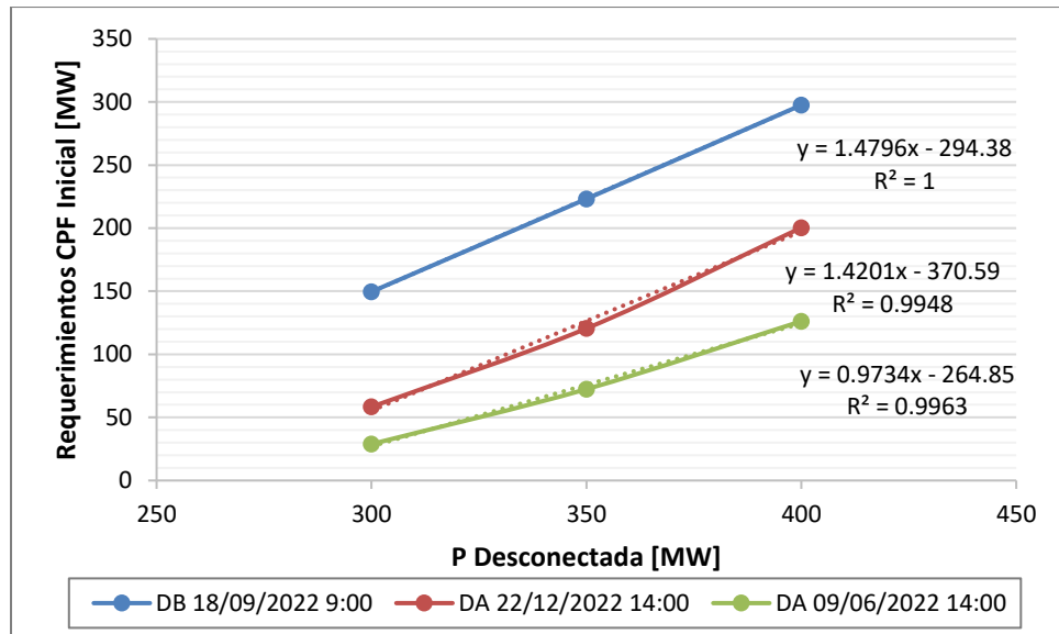
Figura 20: Requerimientos de CPF Inicial vs Gx Desconectada. Escenarios DA 22-12-2022 y DB 18-09-2022.
