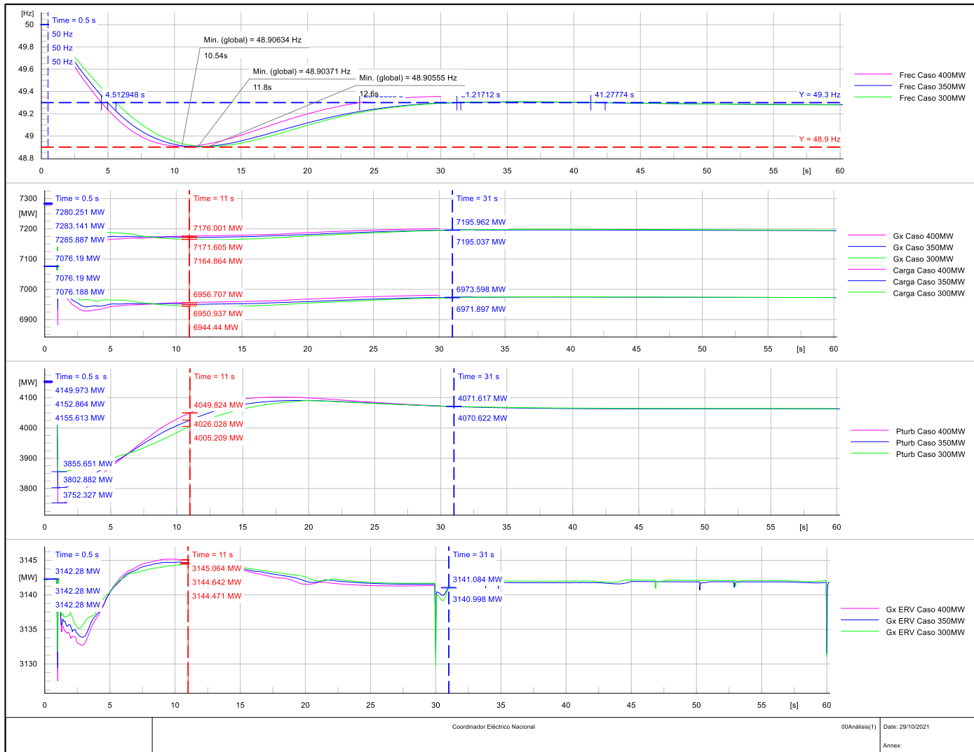
Figura 17: Resultados Análisis Requerimientos de CPF ante Montos Mayores de Desconexión. Caso DB 18-09-2022.
