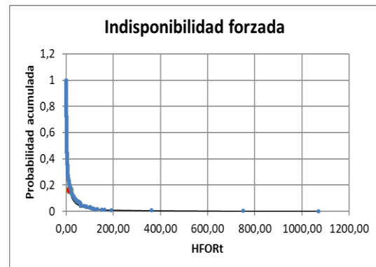
Figura 10: Resultado de índices de indisponibilidad de transmisión Líneas mayor o igual que 100 kV y menor a 220 kV; a) Tabla de índices de indisponibilidad, b) Indisponibilidad programada, c) Frecuencia forzada, d) Indisponibilidad forzada.
