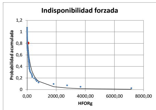
Figura 5: Resultado de índices de indisponibilidad de generación Turbina a Gas; a) Tabla de índices de indisponibilidad, b) Frecuencia Indisponibilidad forzada, c) Indisponibilidad programada, d) Indisponibilidad forzada.
