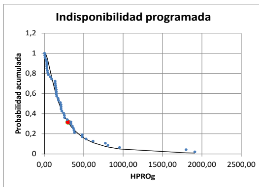
Figura 5: Resultado de índices de indisponibilidad de generación Turbina a Gas; a) Tabla de índices de indisponibilidad, b) Frecuencia Indisponibilidad forzada, c) Indisponibilidad programada, d) Indisponibilidad forzada.
