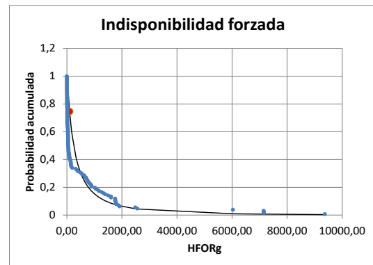
Figura 6: Resultado de índices de indisponibilidad de generación de Motores Diésel; a) Tabla de índices de indisponibilidad, b) Frecuencia Indisponibilidad forzada, c) Indisponibilidad programada, d) Indisponibilidad forzada.
