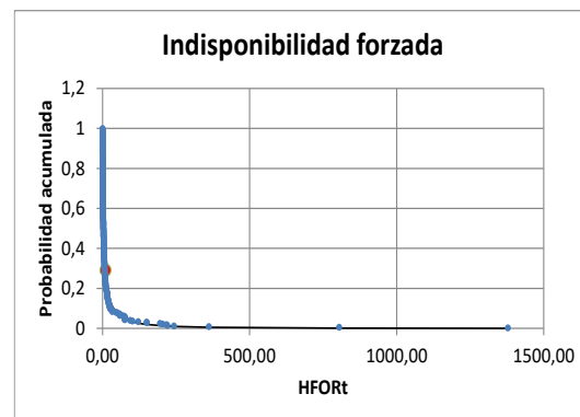
Figura 11: Resultado de índices de indisponibilidad de transmisión Líneas mayor o igual que 220 kV y menor a 500 kV; a) Tabla de índices de indisponibilidad, b) Frecuencia Indisponibilidad forzada, c) Indisponibilidad programada, d) Indisponibilidad forzada.
