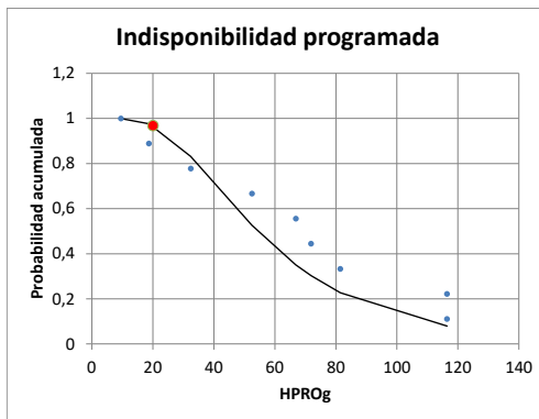
Figura 7: Resultado de índices de indisponibilidad de generación Parque de Motores Diésel; a) Tabla de índices de indisponibilidad, b) Frecuencia Indisponibilidad forzada, c) Indisponibilidad programada, d) Indisponibilidad forzada.
