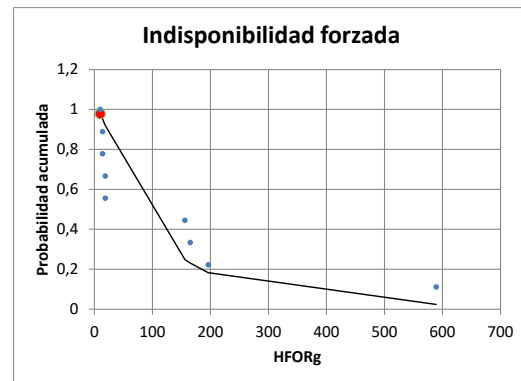
Figura 7: Resultado de índices de indisponibilidad de generación Parque de Motores Diésel; a) Tabla de índices de indisponibilidad, b) Frecuencia Indisponibilidad forzada, c) Indisponibilidad programada, d) Indisponibilidad forzada.
