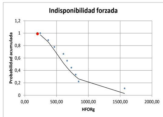
Figura 3: Resultado de índices de indisponibilidad de generación Térmica de Ciclo Combinado; a) Tabla de índices de indisponibilidad, b) Frecuencia Indisponibilidad forzada, c) Indisponibilidad programada, d) Indisponibilidad forzada.
