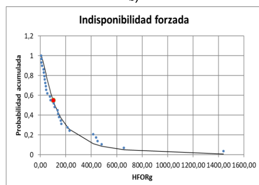
Figura 1: Resultado de índices de indisponibilidad de generación Hidráulica de Embalse; a) Tabla de índices de indisponibilidad, b) Frecuencia Indisponibilidad forzada, c) Indisponibilidad programada, d) Indisponibilidad forzada.
