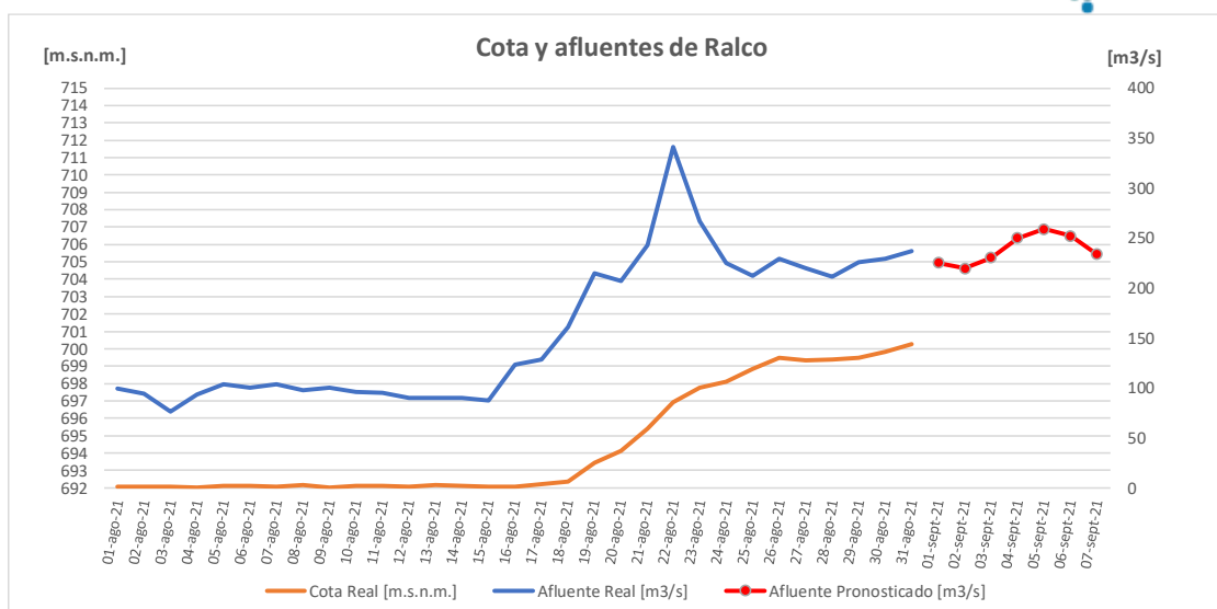
Figura 10. Cota, afluentes reales y proyectados de Ralco al 30 de agosto de 2021
