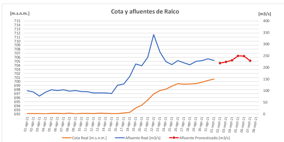
Figura 11. Cota, afluentes reales y proyectados de Ralco al 31 de agosto de 2021
