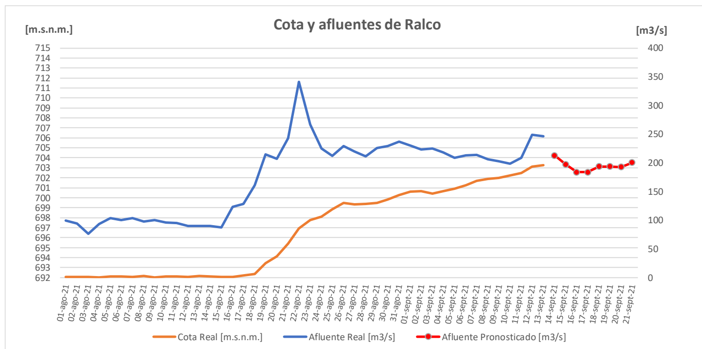
Figura 12. Cota, afluentes reales y proyectados de Ralco al 14 de septiembre de 2021
