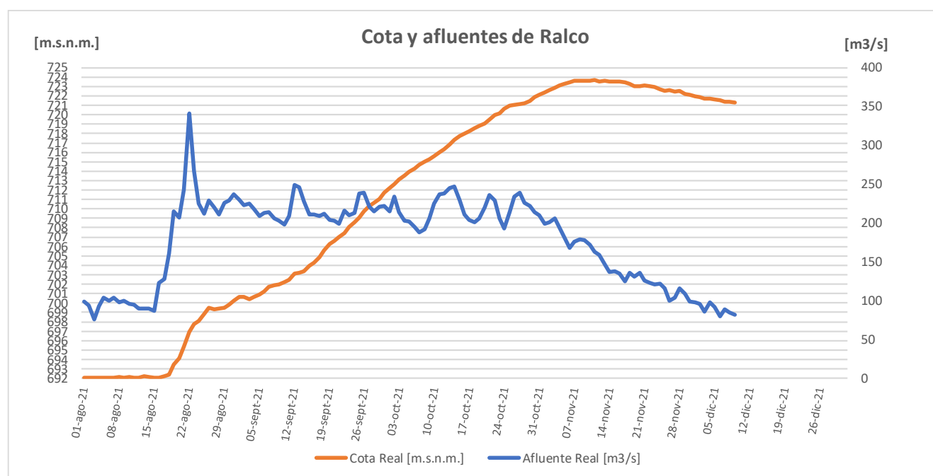
Figura 13. Cota y afluentes reales de Ralco al 09 de diciembre de 2021
