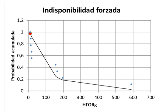
Figura 7: Resultado de índices de indisponibilidad de generación Parque de Motores Diésel; a) Tabla de índices de indisponibilidad, b) Frecuencia Indisponibilidad forzada, c) Indisponibilidad programada, d) Indisponibilidad forzada.
