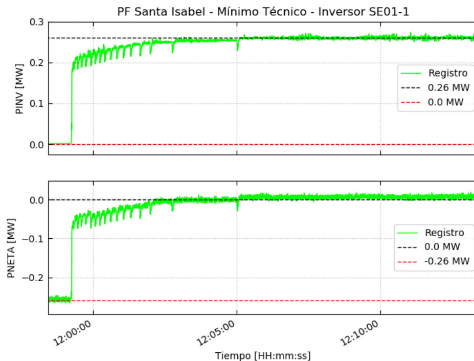
Figura 4.1 – Mínimo Técnico – Inversor SE01-1
