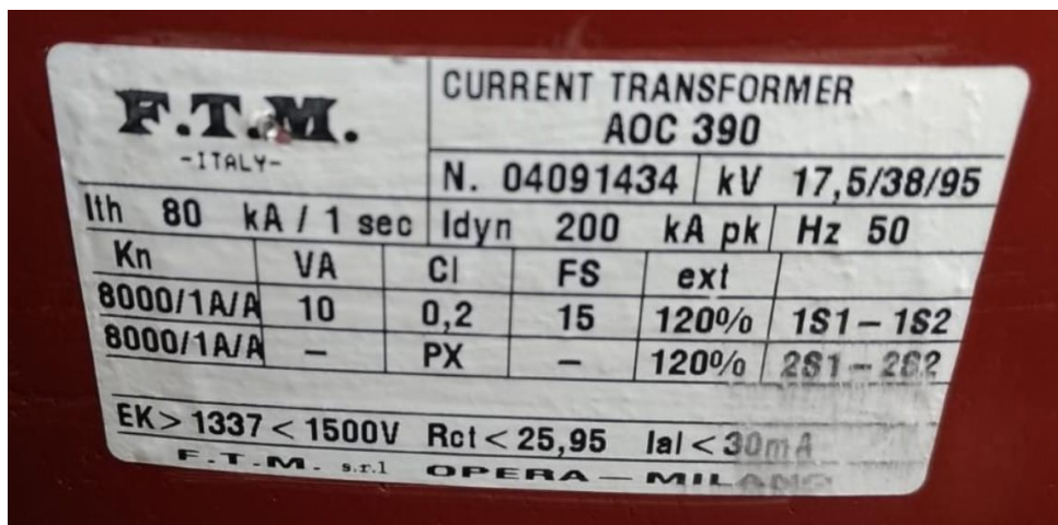
Figura 9.5 – Datos de placa del transformador de corriente para medición de potencia bruta
