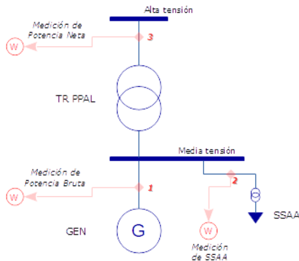
Figura 4.13 – Unilineal de planta esquemático
