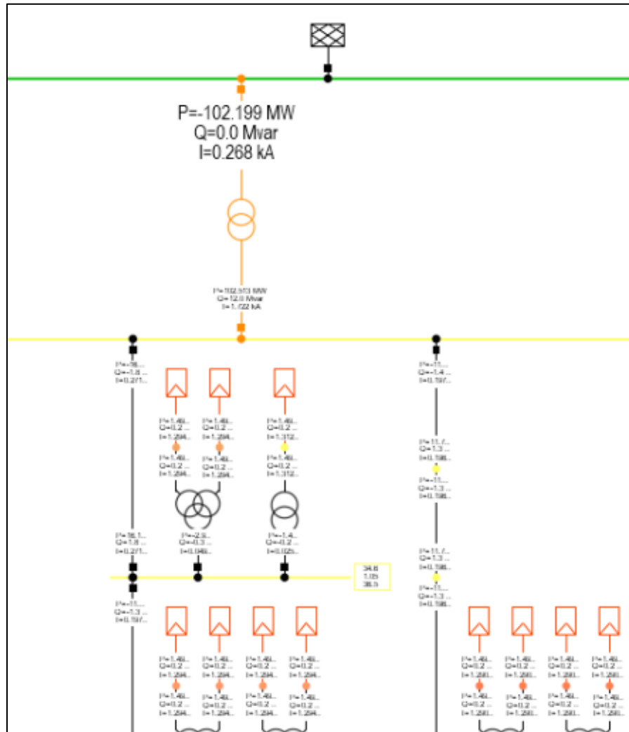
Figura 7-3 Simulación de la condición registrada en terreno en PowerFactory.
