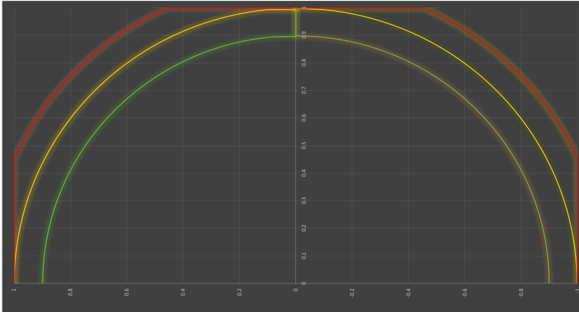
Figura 0-1 Curva de capacidad del inversor.
