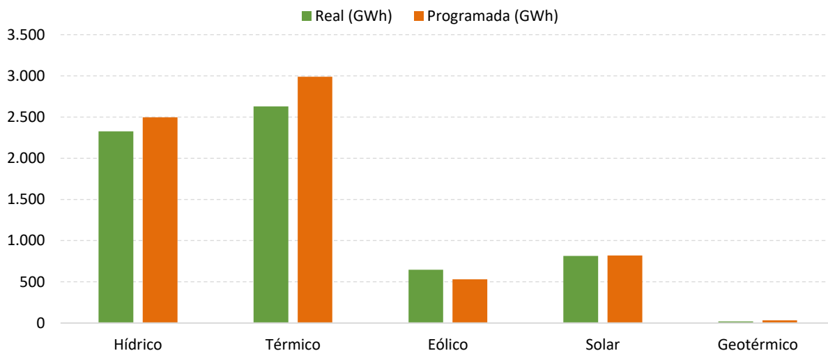
Figura 4: Comparación Generación Real y Programada por fuente.
