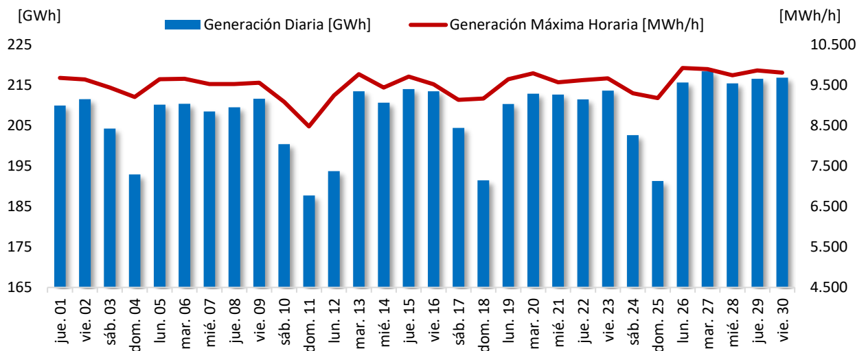
Figura 6: Generación de energía diaria y demanda máxima diaria SEN.
