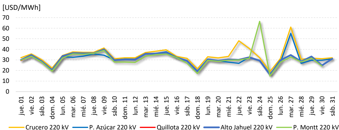
Figura 3: Costos Marginales Promedio Diarios en el SEN.
