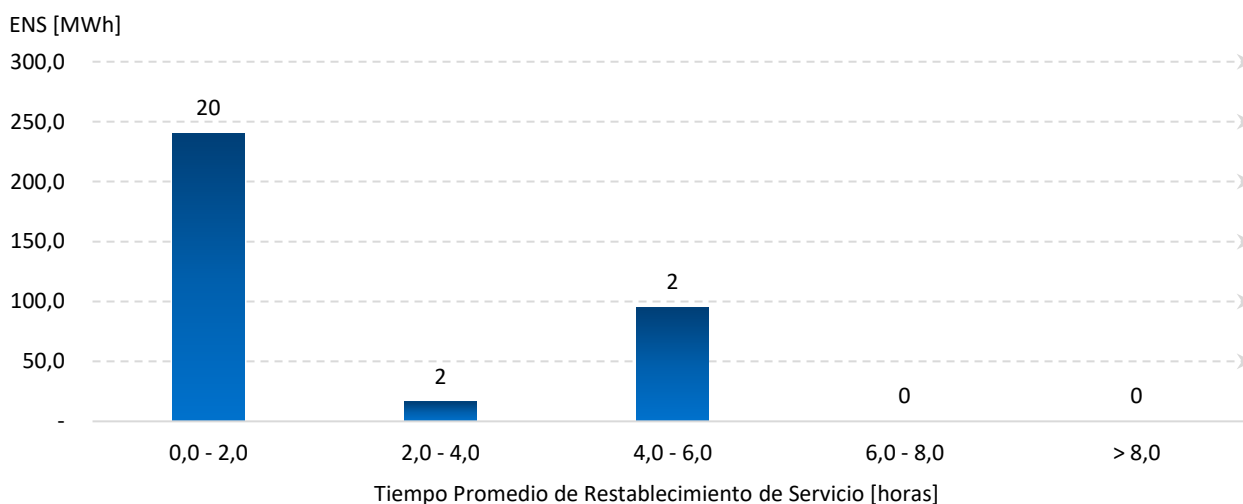
Figura 8: ENS según duración promedio de falla durante octubre (resultados preliminares).
