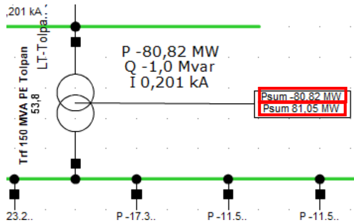
Figura 5.4: Cálculo de flujo de potencia en la línea de transmisión de 220 entre S/E Tolpán Sur y S/E Mulchén [3].
