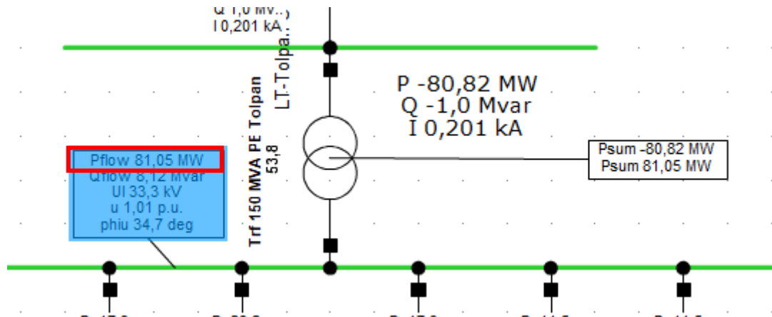
Figura 5.6: Cálculo de flujo de potencia en la barra colectora de 33 kV del praque eólico Tolpán Sur, considerando la modelación de la red de media tensión de 33 kV [3].
