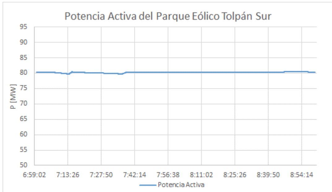
Figura 5.1: Gráfico de potencia activa del parque eólico Tolpán Sur – fecha de realización 30/08/2020-.
