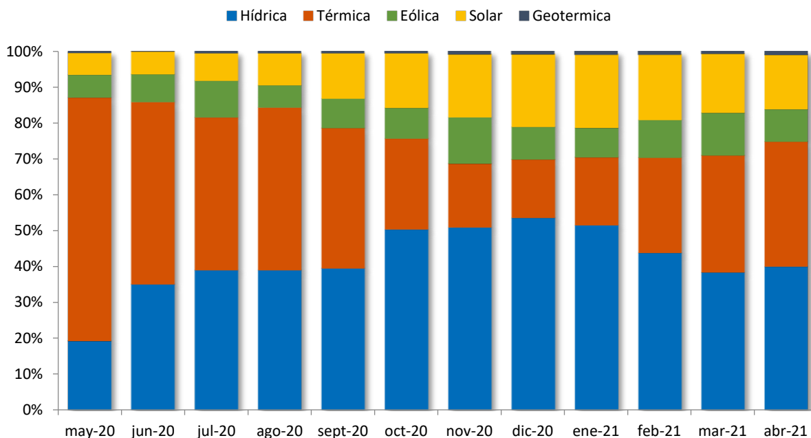
Figura 15: Abastecimiento esperado hidrología húmeda en el SEN.
