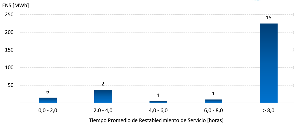
Figura 10: ENS según duración promedio de falla durante abril (resultados preliminares).
