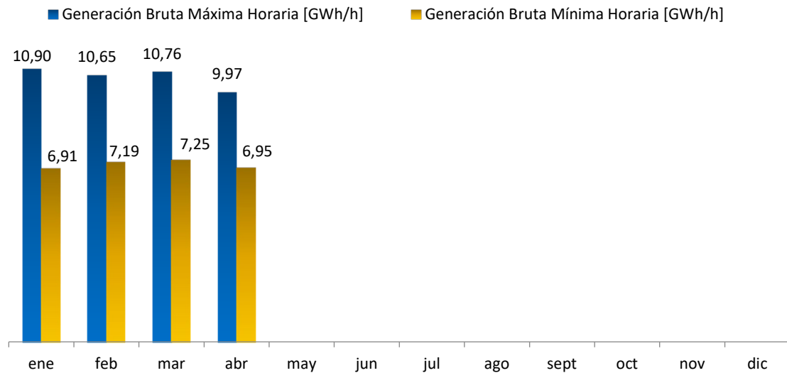
Figura 8: Generación bruta horaria Mín/Máx del SEN 2020.
