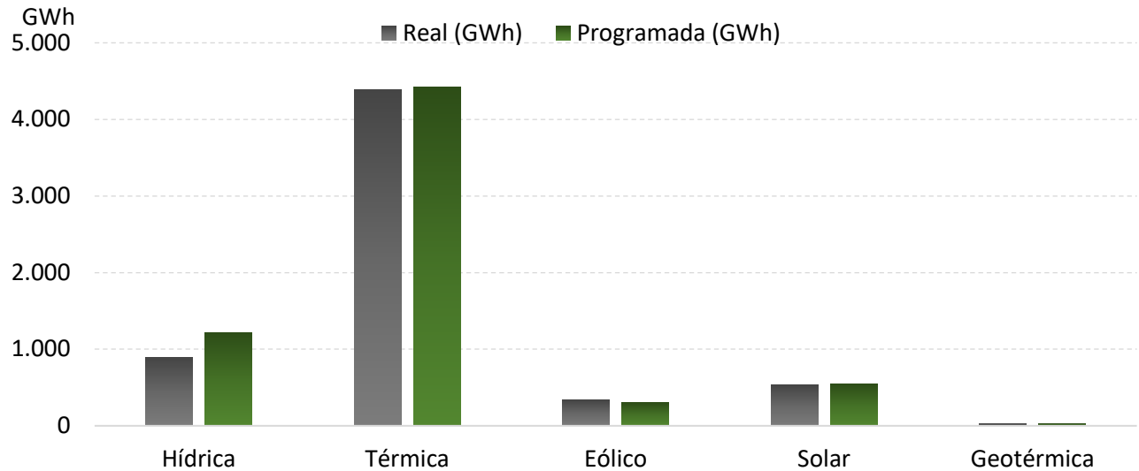
Figura 5: Comparación Generación Real y Programada por fuente.
