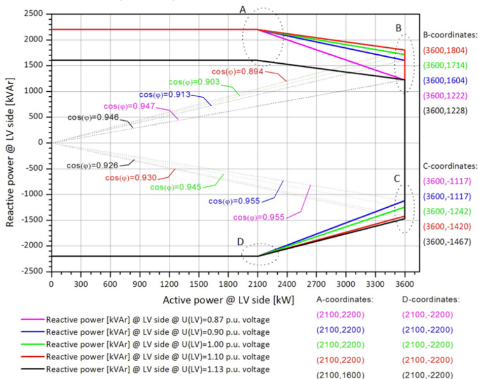
Figura 6: Curva PQ de aerogenerador V136-3.6MW PO1 La Flor.
