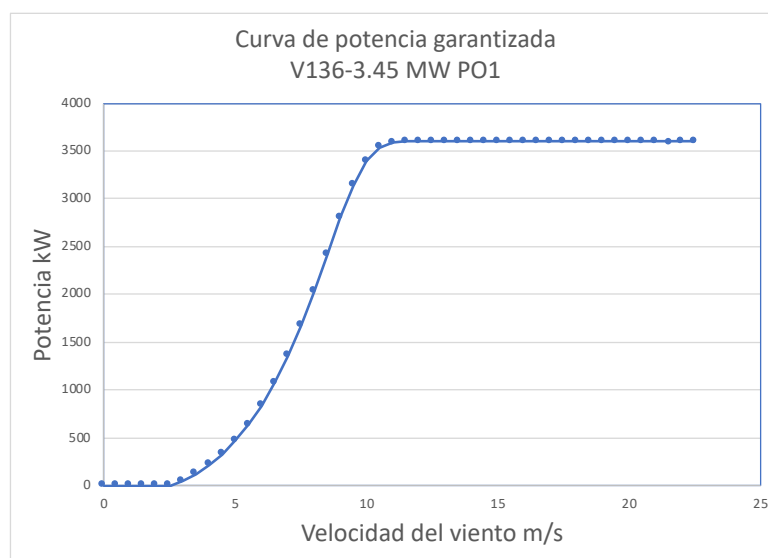
Figura 3: Curva de potencia para aerogenerador V136 – 3.6MW PO1 La Flor.
