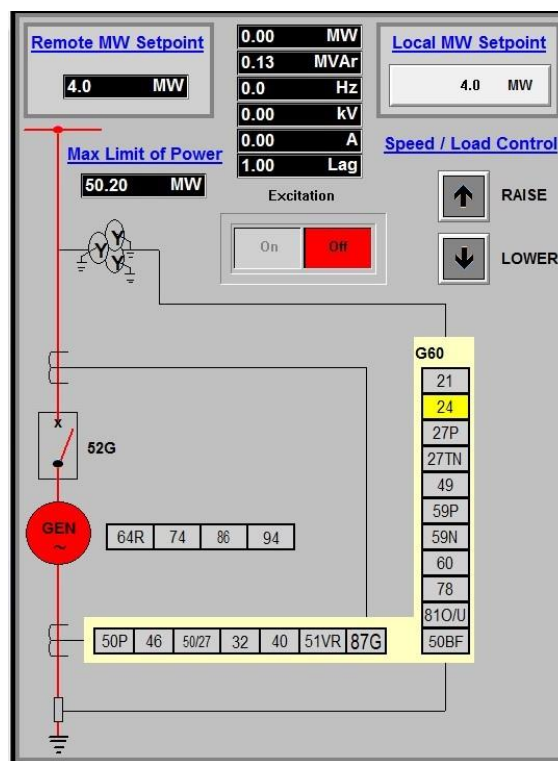
Figura 6-1: Captura de pantalla del sistema de control del generador.
