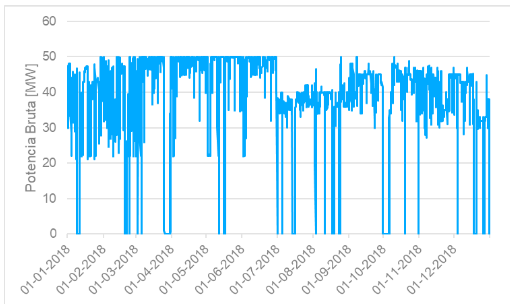
Figura 6-2: Registro de potencia bruta horario año 2018.
