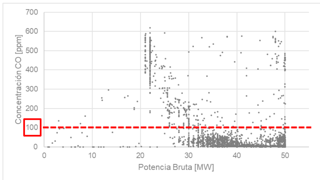
Figura 6-7: Registro de emisiones de CO y Potencia Bruta durante el año 2018.
