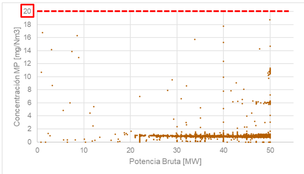
Figura 6-6: Detalle de registro de emisiones de MP según Potencia Bruta durante el año 2018.
