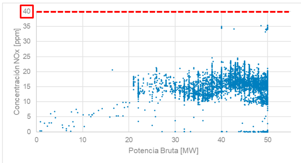
Figura 6-4: Registro de emisiones de NO x según Potencia Bruta durante el año 2018.
