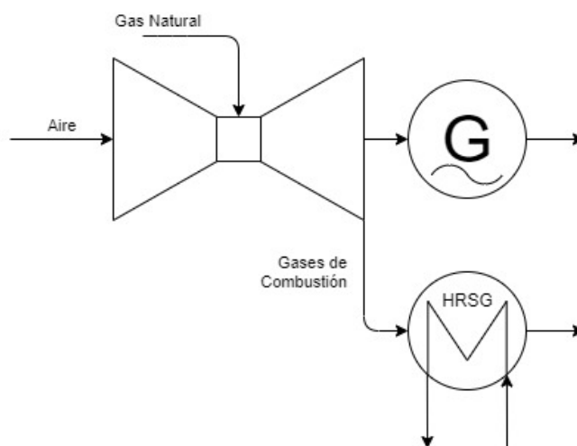
Figura 5-1: Diagrama simplificado de la central CMPC Cordillera.
