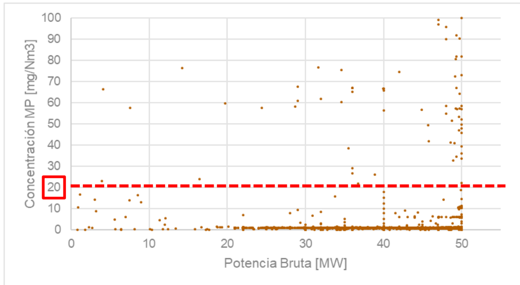
Figura 6-5: Registro de emisiones de MP según Potencia Bruta durante el año 2018.
