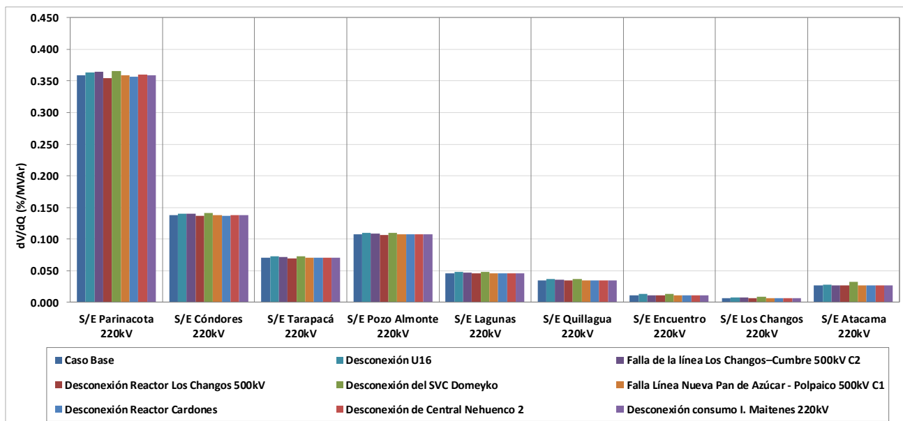
Figura 12 Sensibilidad de tensión ( dV/dQ ) en barras de 220kV de la Zona Norte Grande en E2.
