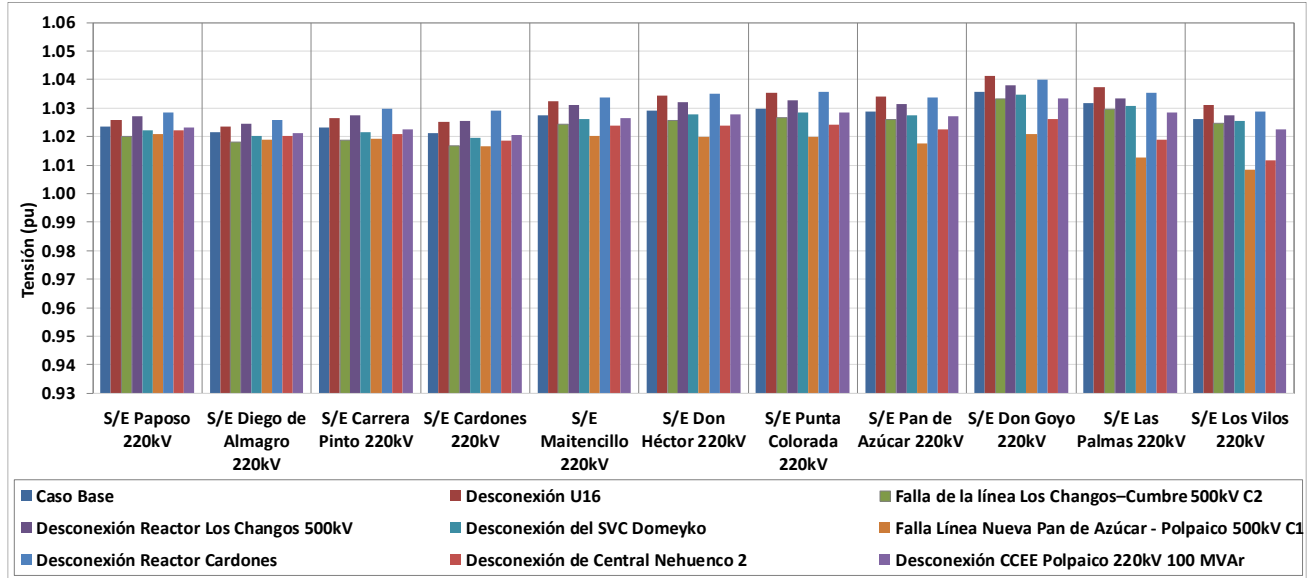
Figura 15 Tensiones en barras de 220kV de la Zona Norte Chico en E1.
