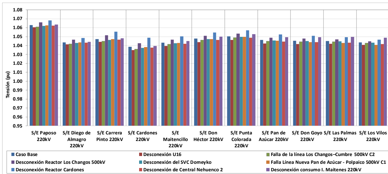
Figura 17 Tensiones en barras de 220kV de la Zona Norte Chico en E2.
