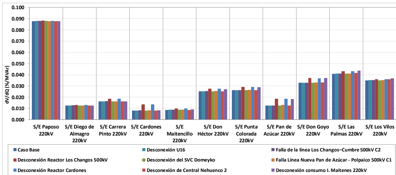
Figura 16 Sensibilidad de tensión ( dV/dQ ) en barras de 220kV de la Zona Norte Chico en E2.
