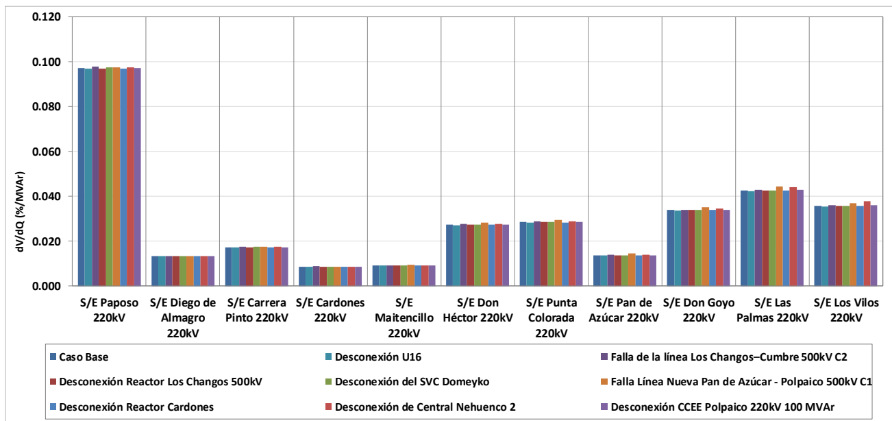
Figura 14 Sensibilidad de tensión ( dV/dQ ) en barras de 220kV de la Zona Norte Chico en E1.
