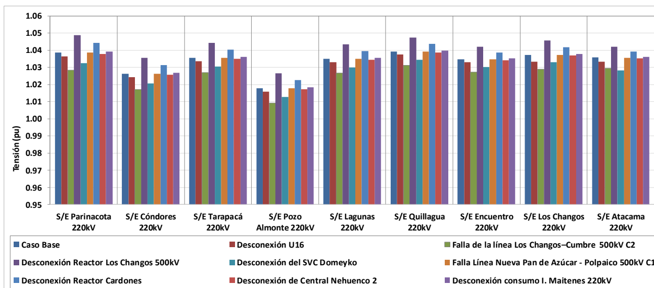
Figura 13 Tensiones en barras de 220kV de la Zona Norte Grande en E2.
