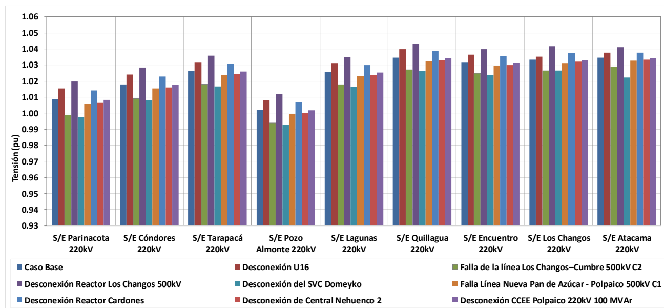
Figura 11 Tensiones en barras de 220kV de la Zona Norte Grande en E1.
