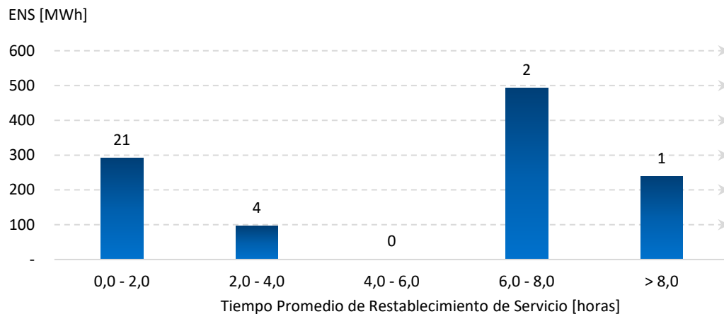
Figura 12: ENS según duración promedio de falla durante octubre (resultados preliminares).
