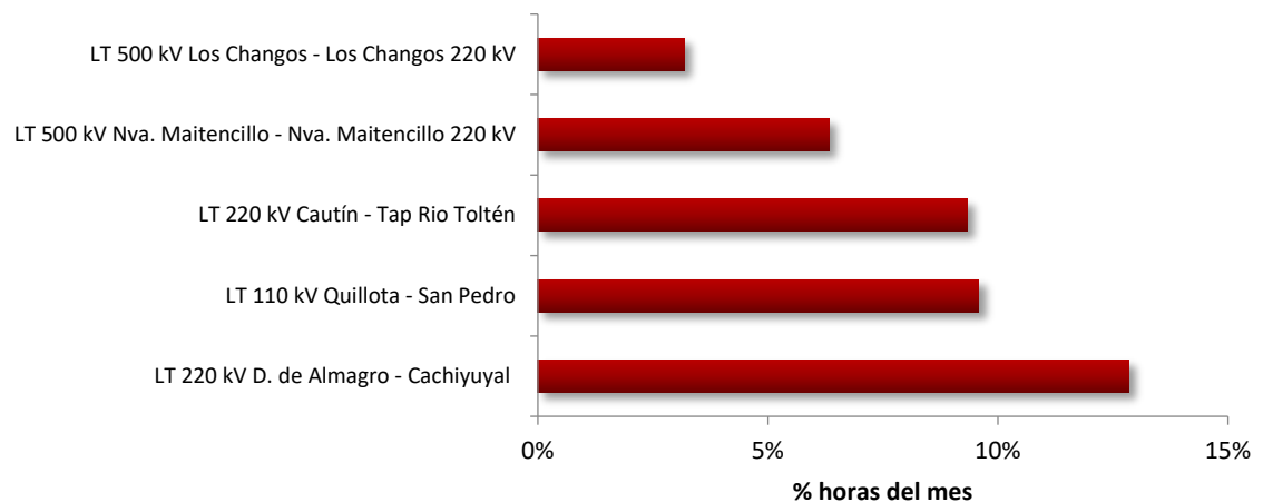
Figura 2: Mayores Tiempos de Desacople en el SEN.
