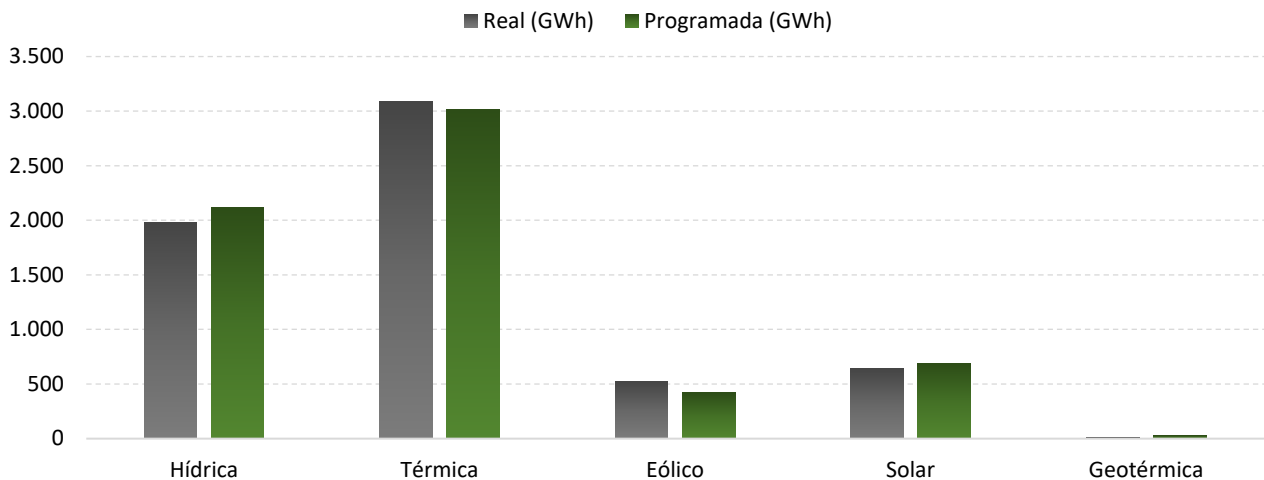
Figura 6: Comparación Generación Real y Programada por fuente.
