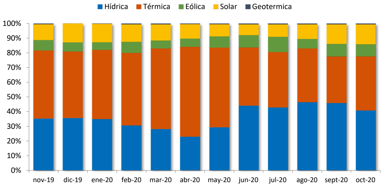
Figura 16: Abastecimiento esperado hidrología media en el SEN.
