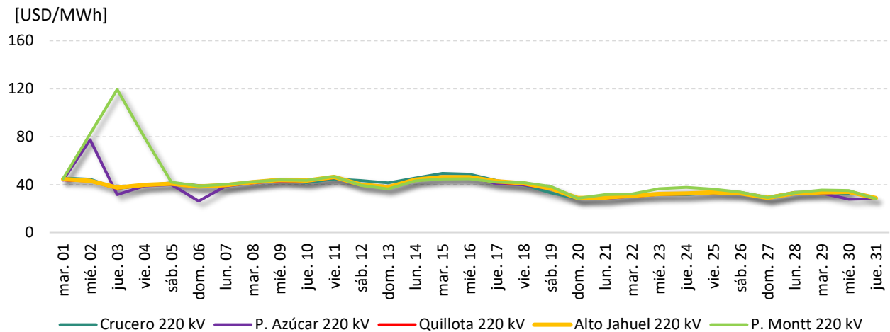
Figura 4: Costos Marginales Promedio Diarios en el SEN.
