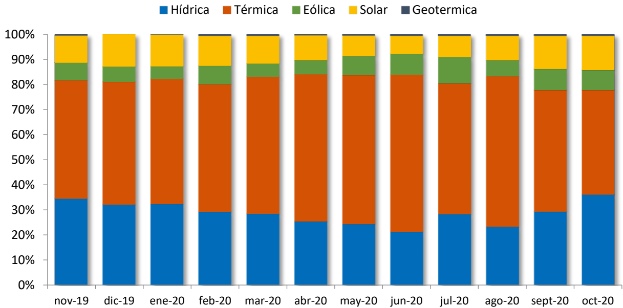
Figura 15: Abastecimiento esperado hidrología seca en el SEN.
