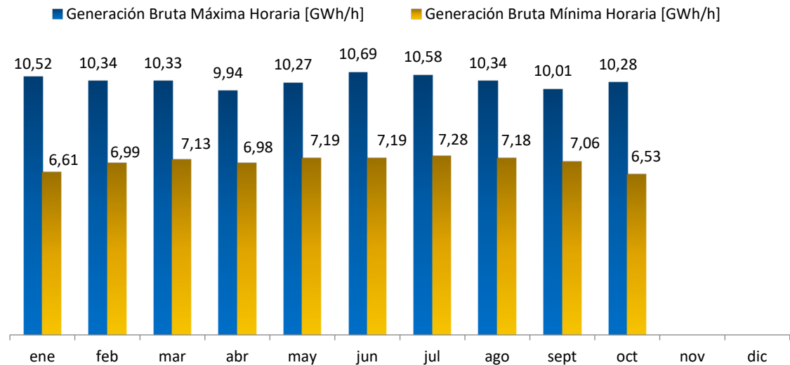
Figura 9: Generación bruta horaria Mín/Máx del SEN 2019.
