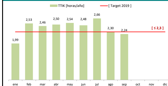
Figura 1.4. Tiempo Total de Interrupciones de Suministro - TTIK
