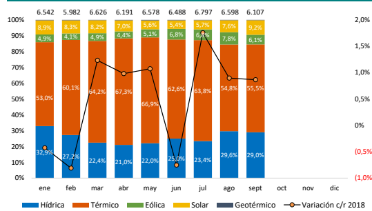
Figura 2.2. Producción Real de Energía [GWh]
