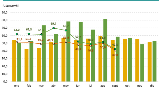
Figura 2.8. CMg Promedio Mensual [USD/MWh]: SS/EE Quillota y Cruceo
