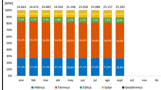
Figura 2.1. Capacidad Instalada de Generación [MW]
