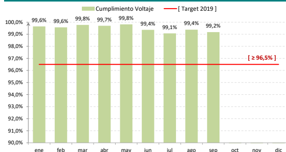
Figura 1.2. Control de Tensión - Cumplimiento
