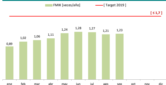
Figura 1.5. Frecuencia Media de Interrupciones de Suministro - FMIK
