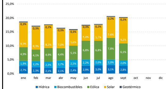
Figura 2.4. Producción de ERNC [GWh]
