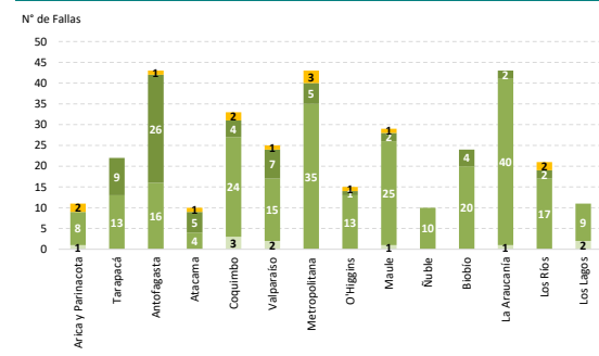
Figura 1.9. Fallas en el SEN (por Región y Segmento de Origen)
