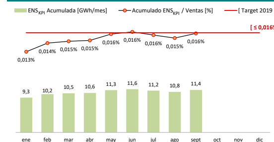
Figura 1.6. Energía No Suministrada por Fallas
