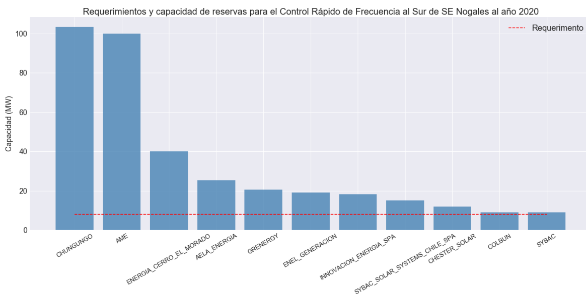
Figura 24. Requerimientos y Capacidad de Control Rápido de Frecuencia al Sur de la S/E Nogales al año 2020
