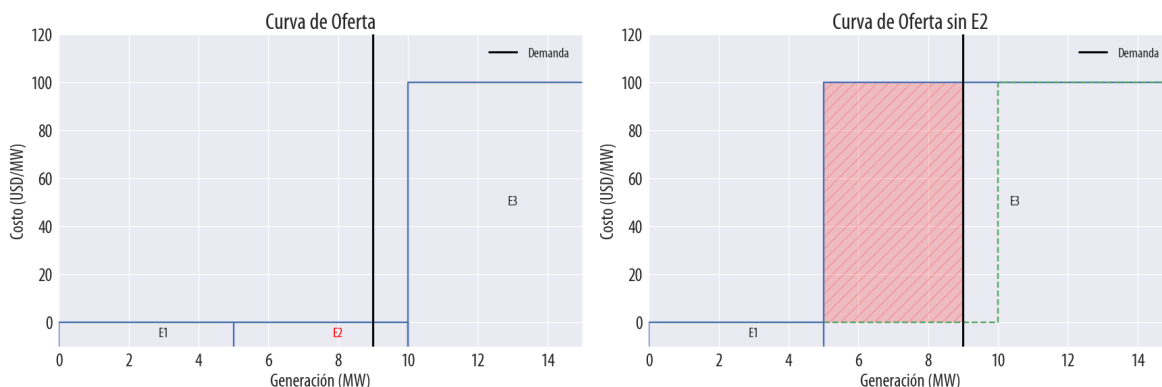
Figura A4. Curva de oferta del Ejemplo 4 con (izquierda) y sin (derecha) un generador.
