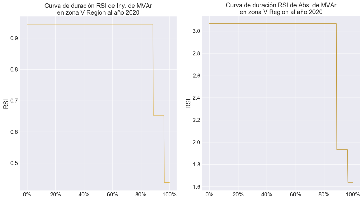
Figura 97. Curva de duración RSI para el Control de Tensión - Inyección de Reactivos (izquierda) y Absorción de Reactivos (derecha) en zona V Región al año 2020
