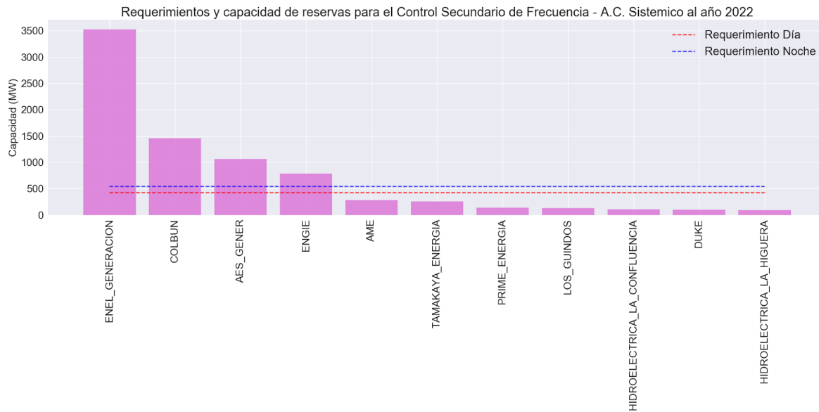
Figura 45. Requerimientos y capacidad de reservas para el Control Secundario de Frecuencia - Aumento de Carga a nivel Sistémico al año 2022
