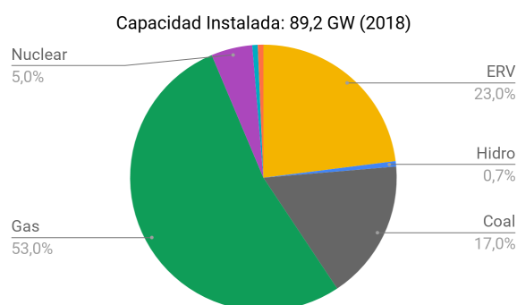
Figura 4: Composición de la matriz energética de ERCOT
