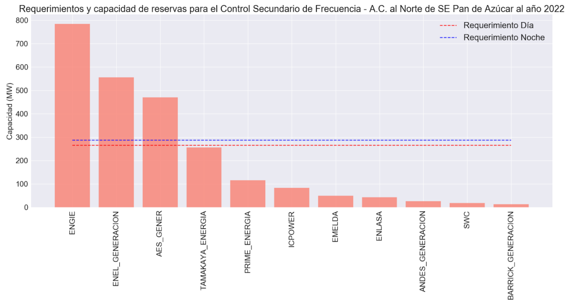
Figura 48. Requerimientos y capacidad de reservas para el Control Secundario de Frecuencia - Aumento de Carga al Norte de la S/E Pan de Azúcar al año 2022
