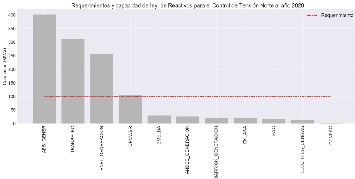
Figura 92. Requerimientos y capacidad de reservas para el Control de Tensión - Inyección de Reactivos en zona Norte al año 2020
