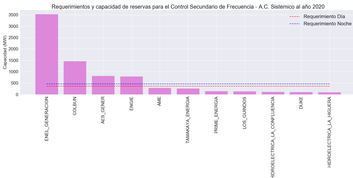
Figura 44. Requerimientos y capacidad de reservas para el Control Secundario de Frecuencia - Aumento de Carga a nivel Sistémico al año 2020
