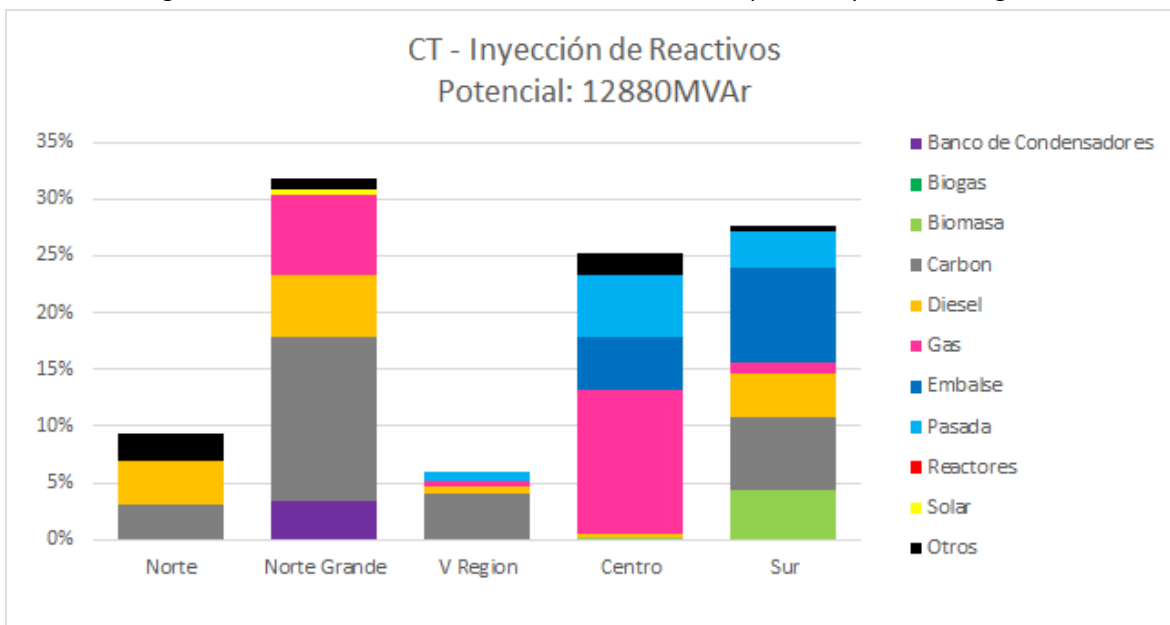
Figura 105. Potencial oferta CT - Inyección de Reactivos por zona y mix tecnológico
