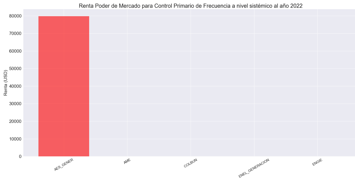
Figura 38. Renta Poder de Mercado para el Control Primario de Frecuencia a nivel sistémico al año 2022
