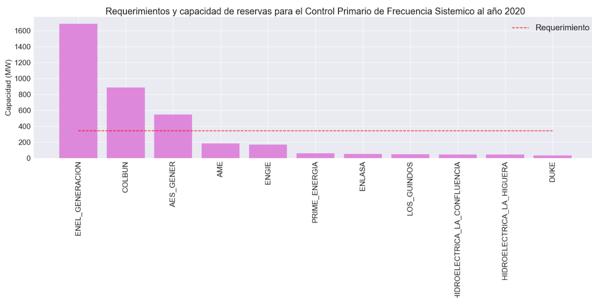
Figura 26. Requerimientos y capacidad de reservas para el Control Primario de Frecuencia a nivel Sistémico al año 2020
