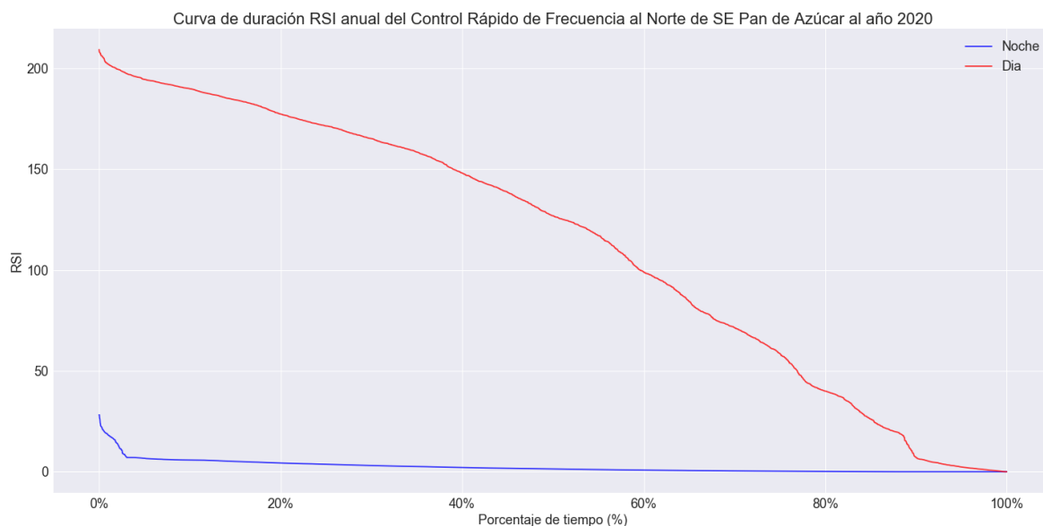
Figura 23. Curva de Duración RSI anual del Control Rápido de Frecuencia al Norte de la S/E Pan de Azúcar al año 2020
