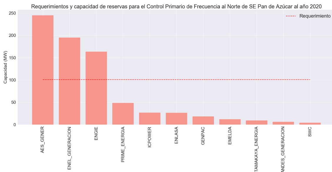
Figura 29. Requerimientos y capacidad de reservas para el Control Primario de Frecuencia al Norte de la S/E Pan de Azúcar al año 2020
