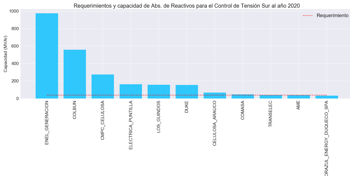
Figura 102. Requerimientos y capacidad de reservas para el Control de Tensión - Absorción de Reactivos en zona Sur al año 2020
