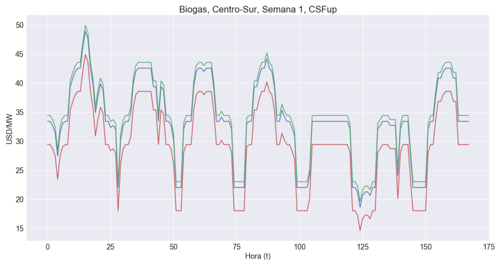
Figura 108. Banda de Precios de Reserva Secundaria - Aumento de Carga para unidades de Biogás en zona Centro-Sur para la primera semana representativa.
