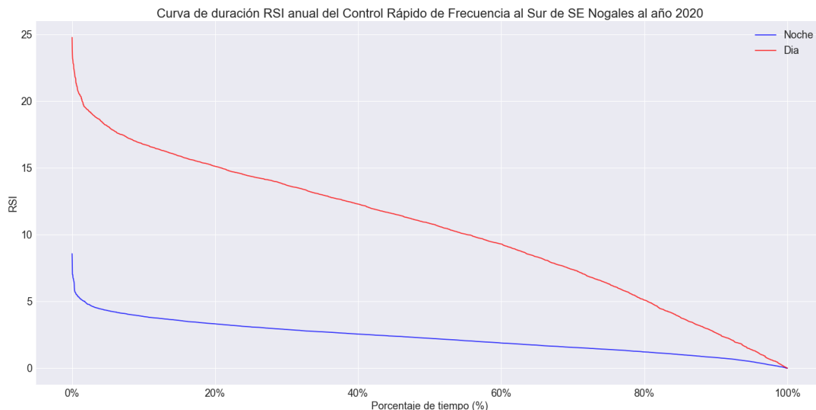
Figura 25. Curva de Duración RSI anual del Control Rápido de Frecuencia al Sur de la S/E Nogales al año 2020
