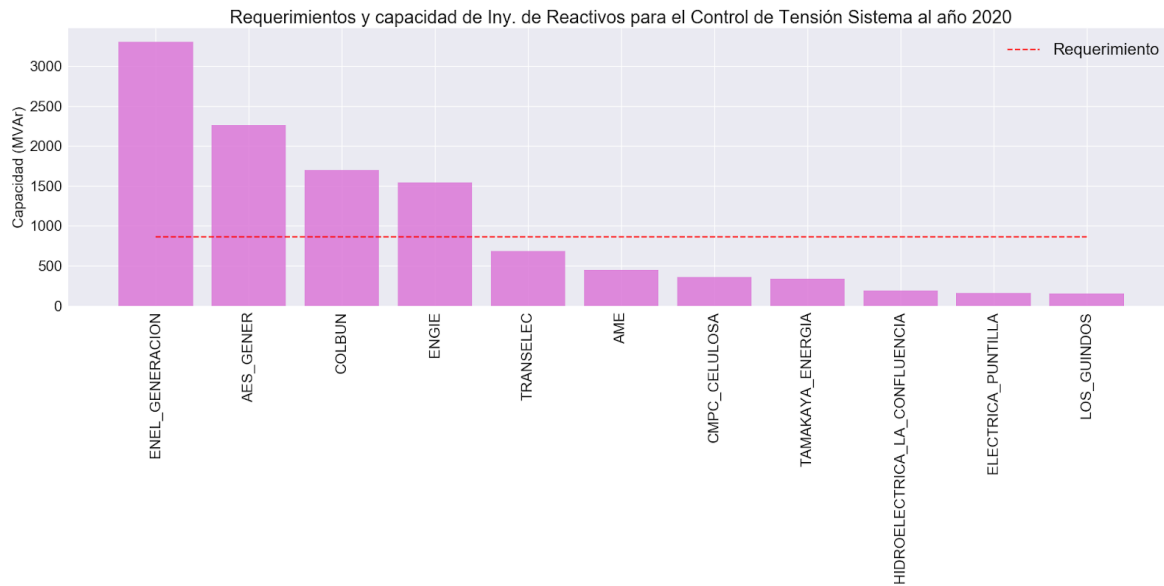
Figura 86. Requerimientos y capacidad de reservas para el Control de Tensión - Inyección de Reactivos a nivel Sistémico al año 2020
