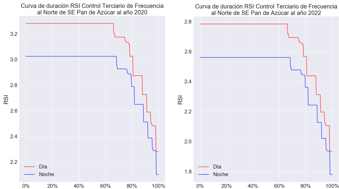
Figura 76. Curva de duración RSI del Control Terciario de Frecuencia al Norte de la S/E Pan de Azúcar al año 2020 (izquierda) y 2022 (derecha)
