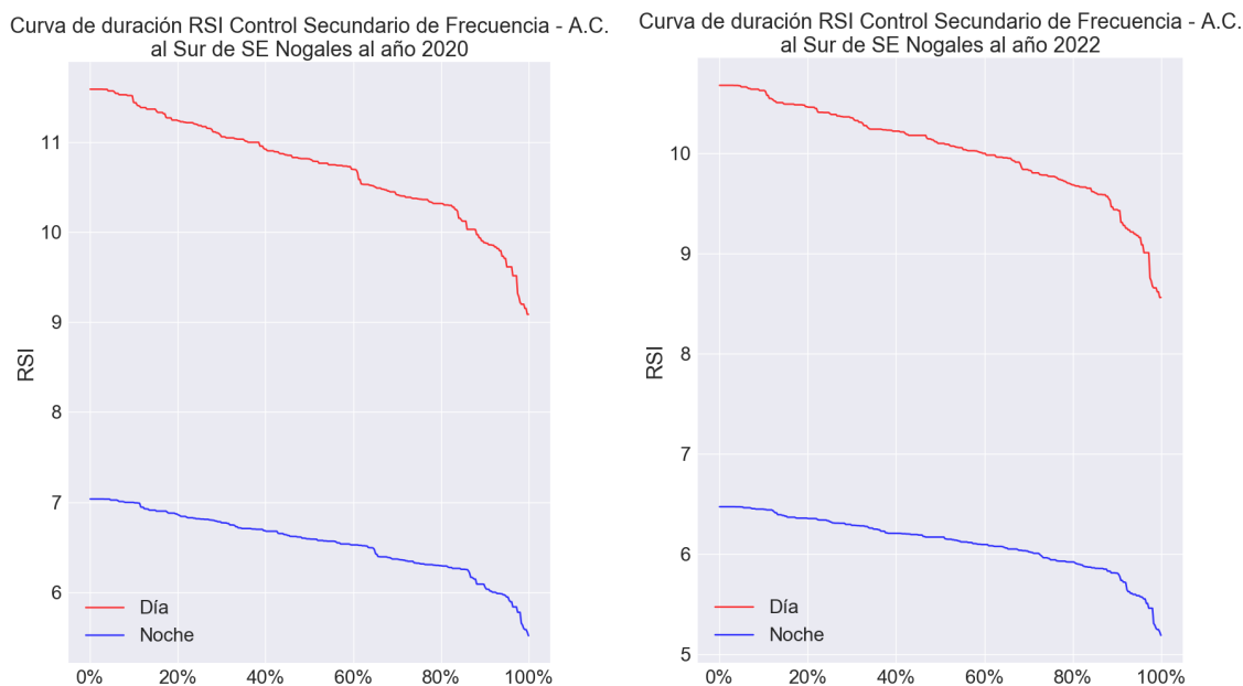
Figura 52. Curva de duración RSI del Control Secundario de Frecuencia - Aumento de Carga al Sur de la S/E Nogales al año 2020 (izquierda) y 2022 (derecha)
