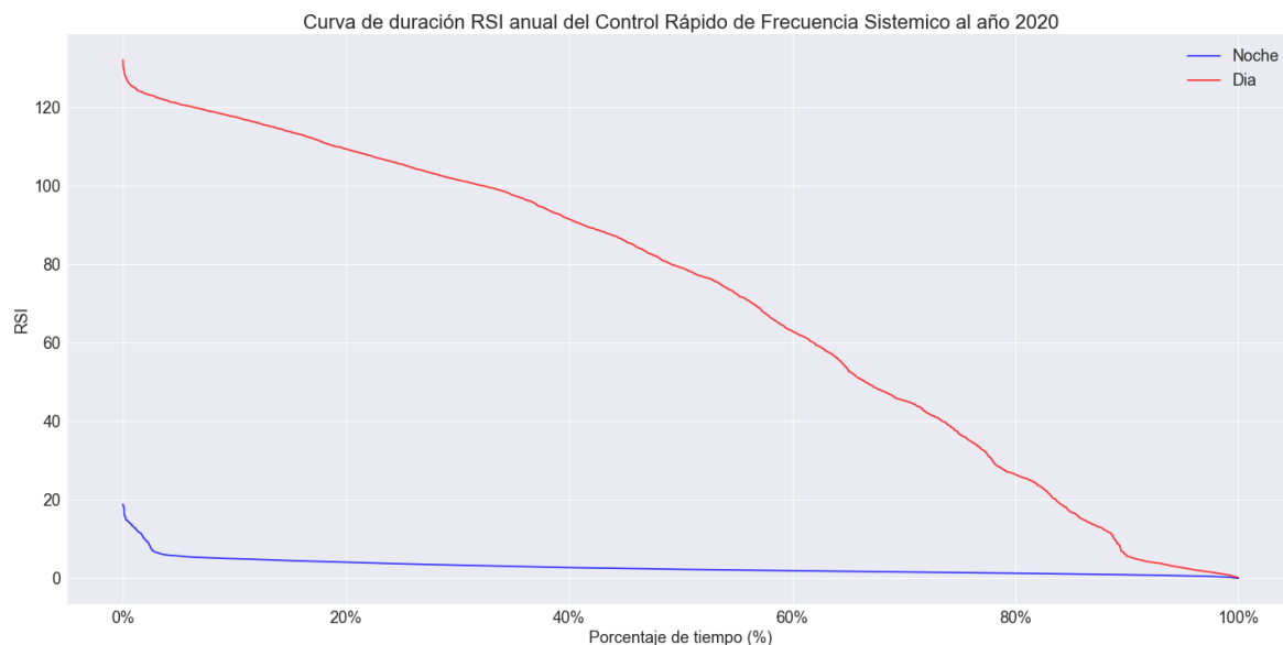
Figura 21. Curva de Duración RS anual de Control Rápido de Frecuencia a Nivel Sistémico al año 2020
