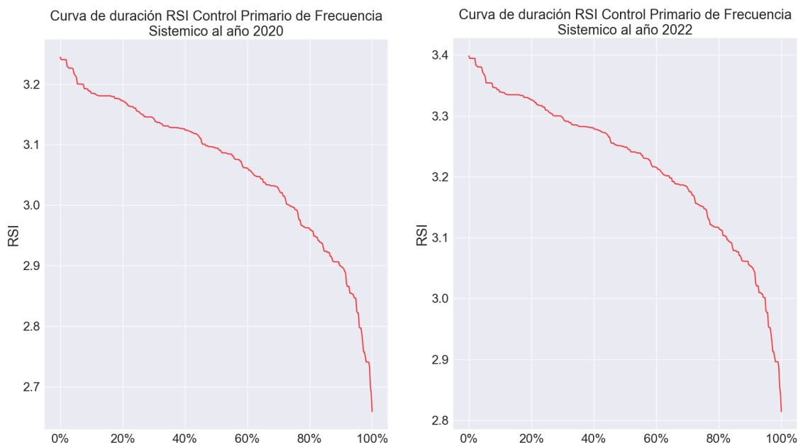
Figura 28. Curva de duración RSI del Control Primario de Frecuencia a nivel Sistémico al año 2020 (izquierda) y 2022 (derecha)
