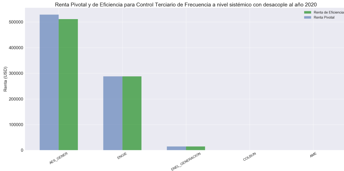
Figura 82. Renta Pivotal y de Eficiencia para Control Terciario de Frecuencia a nivel sistémico con desacople al año 2020
