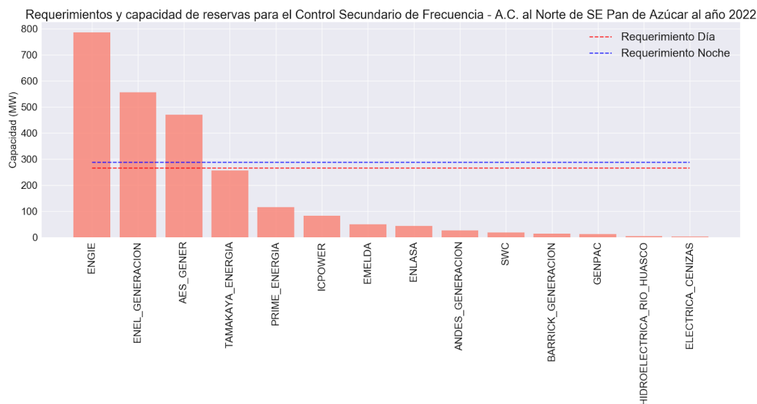
Figura A14. Requerimientos y capacidad de reservas para el Control Secundario de Frecuencia - Aumento de Carga al Norte de la S/E Pan de Azúcar al año 2022
