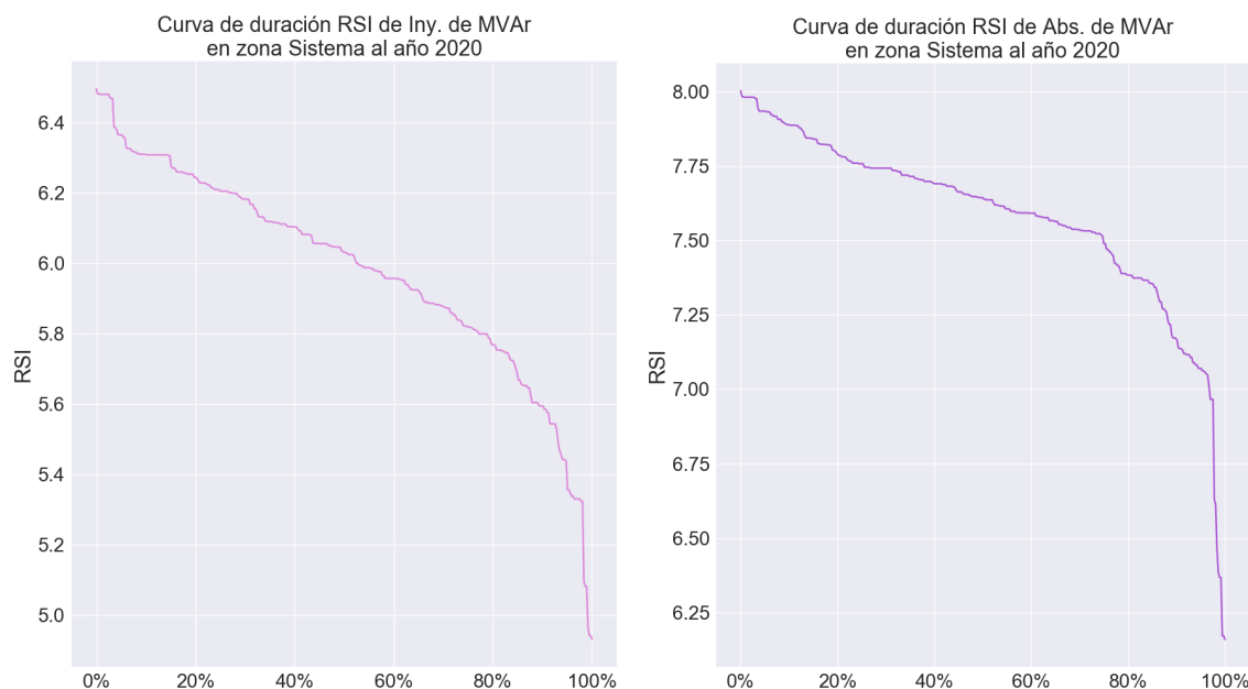
Figura 88. Curva de duración RSI para el Control de Tensión - Inyección de Reactivos (izquierda) y Absorción de Reactivos (derecha) a nivel Sistémico al año 2020
