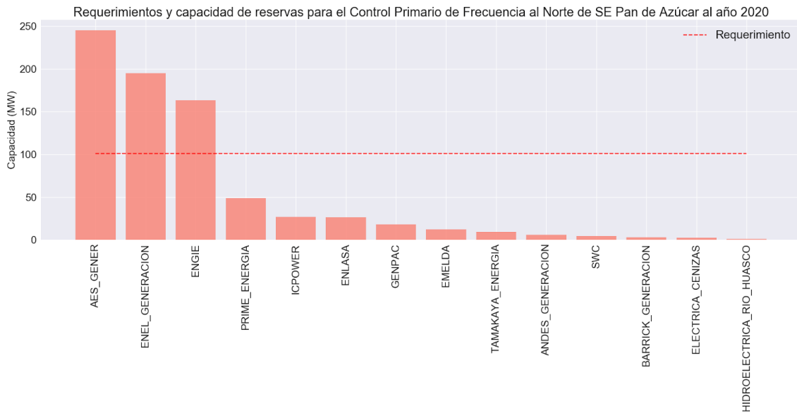
Figura A7. Requerimientos y capacidad de reservas para el Control Primario de Frecuencia al Norte de la S/E Pan de Azúcar al año 2020
