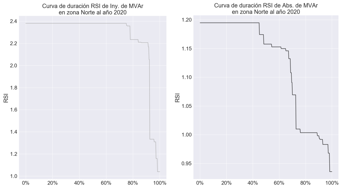
Figura 94. Curva de duración RSI para el Control de Tensión - Inyección de Reactivos (izquierda) y Absorción de Reactivos (derecha) en zona Norte al año 2020
