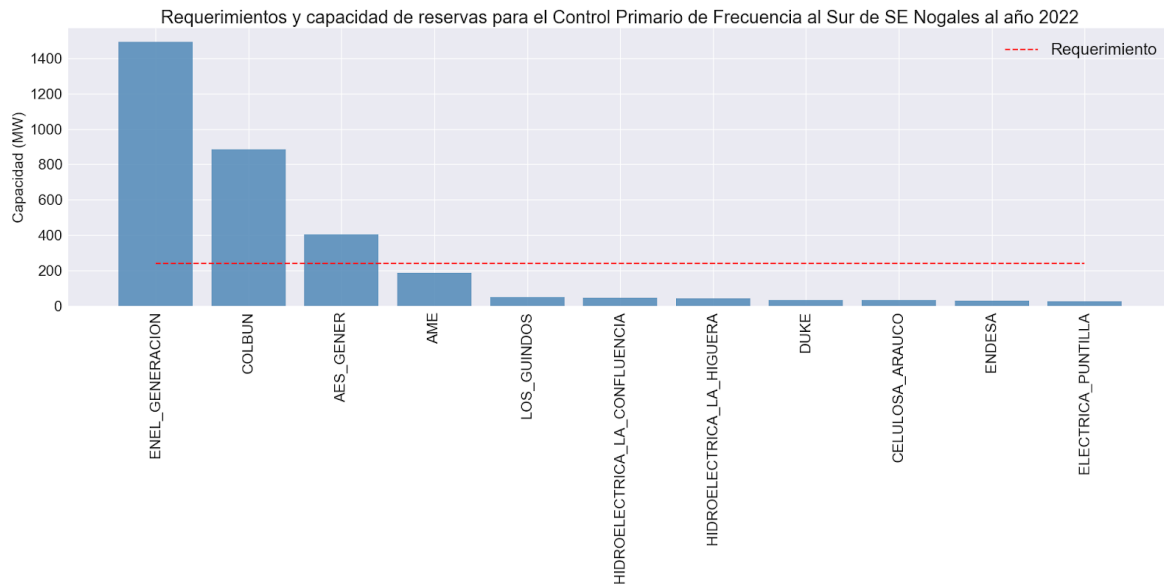
Figura 33. Requerimientos y capacidad de reservas para el Control Primario de Frecuencia al Sur de la S/E Nogales al año 2022
