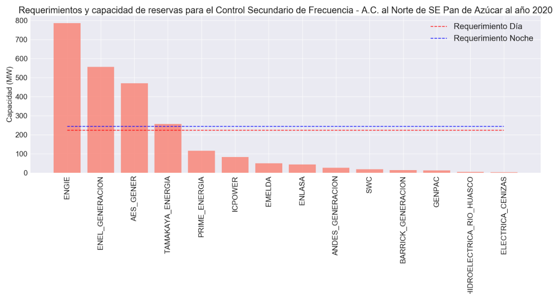
Figura A13. Requerimientos y capacidad de reservas para el Control Secundario de Frecuencia - Aumento de Carga al Norte de la S/E Pan de Azúcar al año 2020
