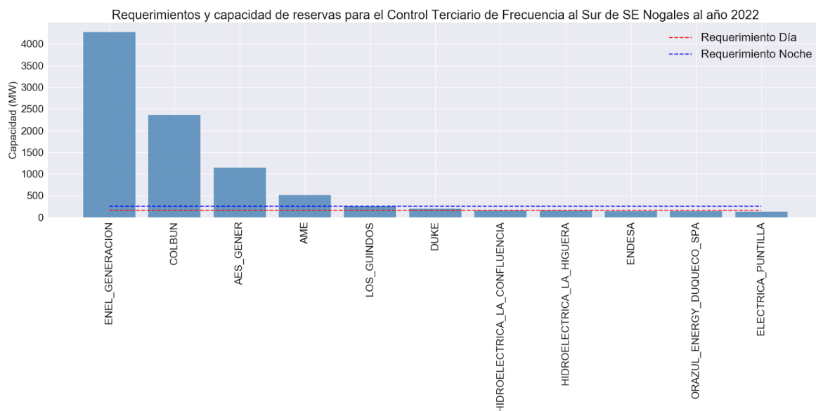
Figura 78. Requerimientos y capacidad de reservas para el Control Terciario de Frecuencia al Sur de la S/E Nogales al año 2022
