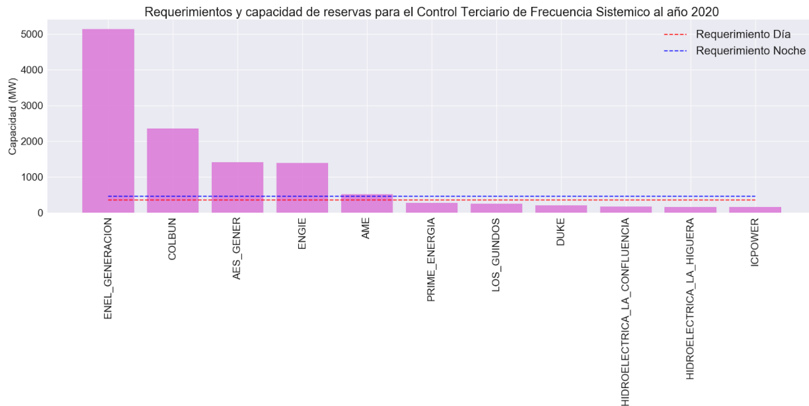
Figura 71. Requerimientos y capacidad de reservas para el Control Terciario de Frecuencia a nivel Sistémico al año 2020
