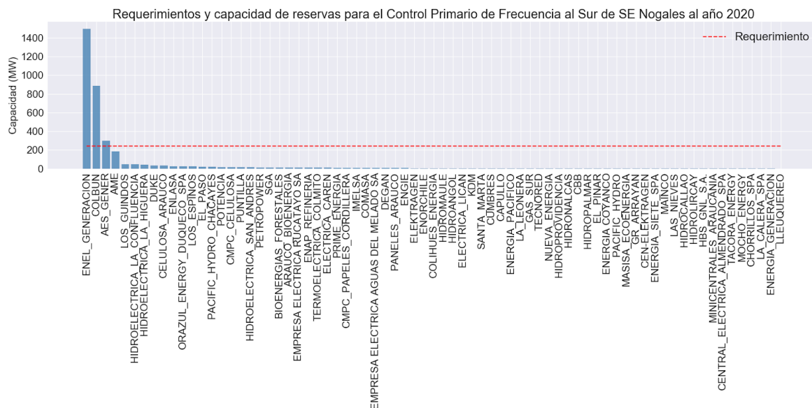
Figura A9. Requerimientos y capacidad de reservas para el Control Primario de Frecuencia al Sur de la S/E Nogales al año 2020
