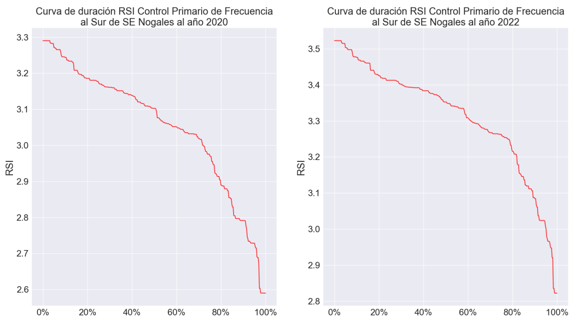
Figura 34. Curva de duración RSI del Control Primario de Frecuencia al Sur de la S/E Nogales al año 2020 (izquierda) y 2022 (derecha)
