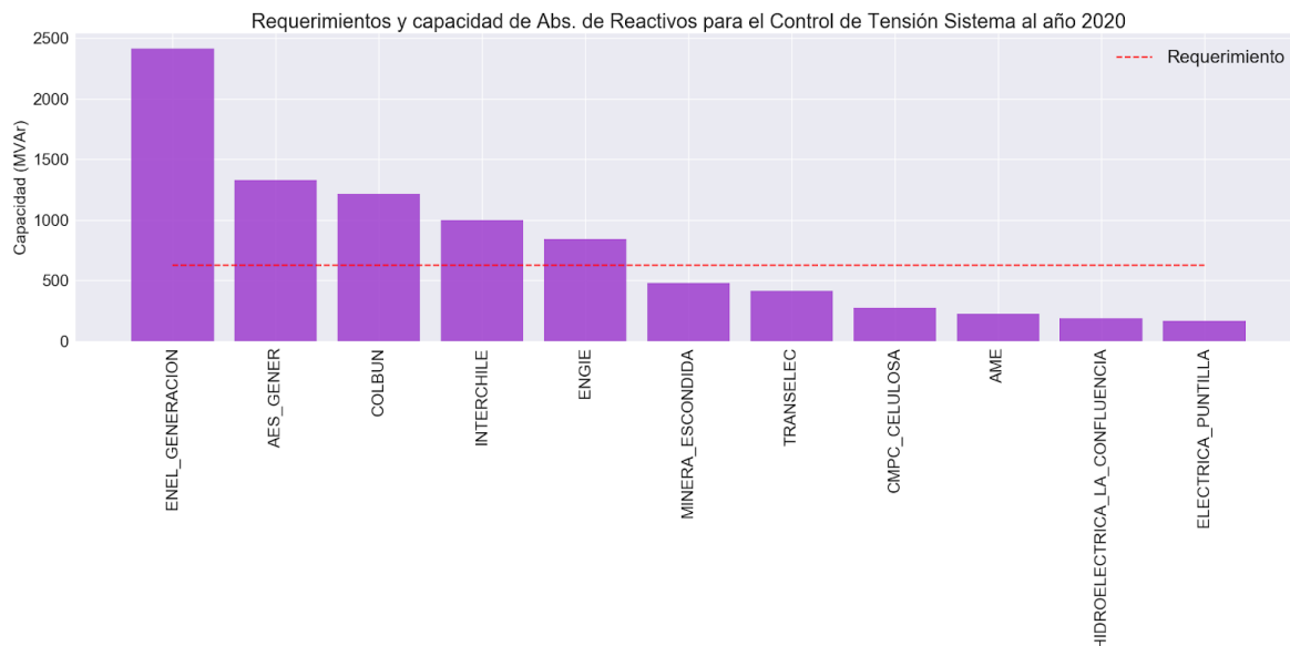
Figura 87. Requerimientos y capacidad de reservas para el Control de Tensión - Absorción de Reactivos a nivel Sistémico al año 2020
