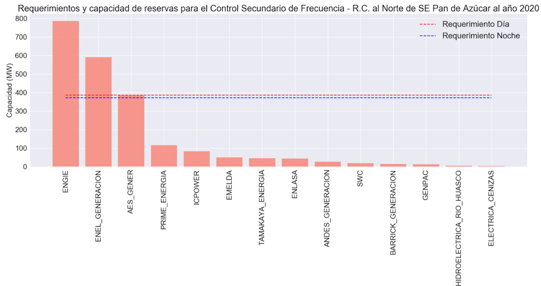
Figura A19. Requerimientos y capacidad de reservas para el Control Secundario de Frecuencia - Reducción de Carga al Norte de la S/E Pan de Azúcar al año 2020
