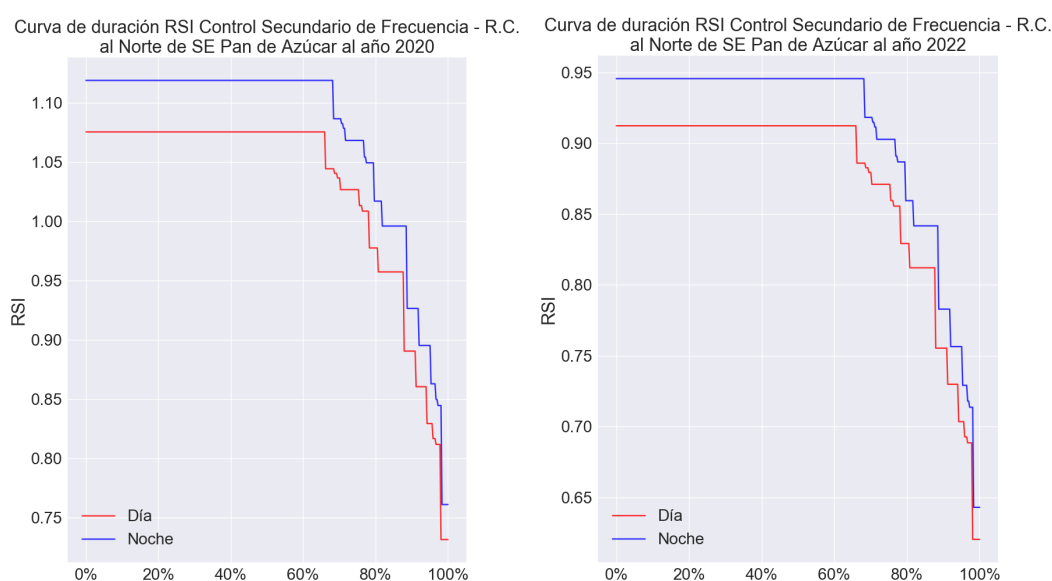
Figura 64. Curva de duración RSI del Control Secundario de Frecuencia - Reducción de Carga al Norte de la S/E Pan de Azúcar al año 2020 (izquierda) y 2022 (derecha)
