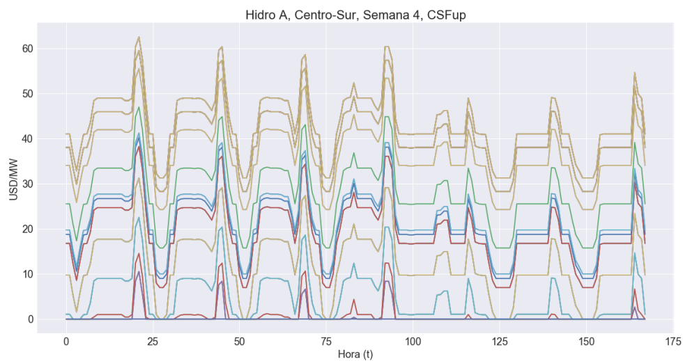
Figura 107. Banda de Precios de Reserva Secundaria - Aumento de Carga para unidades de Hidro A en zona Centro-Sur para la cuarta semana representativa.
