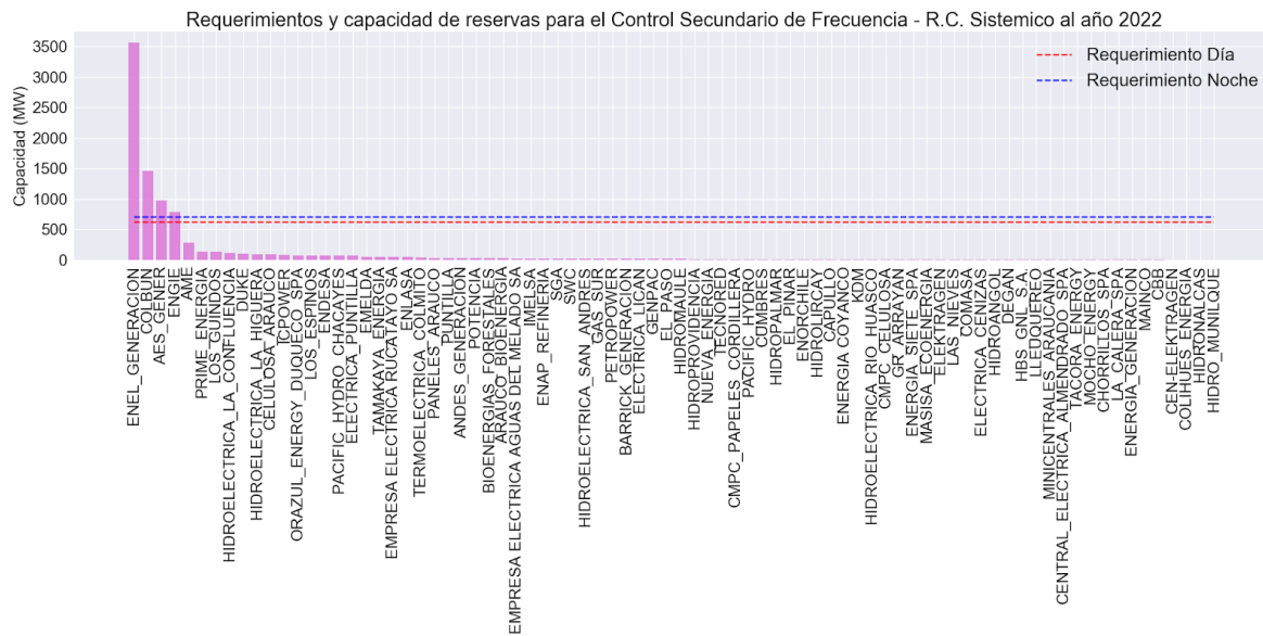
Figura A18. Requerimientos y capacidad de reservas para el Control Secundario de Frecuencia - Reducción de Carga a nivel Sistémico al año 2022
