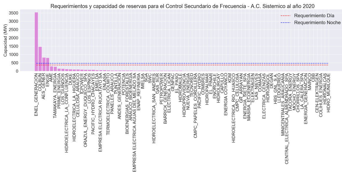
Figura A11. Requerimientos y capacidad de reservas para el Control Secundario de Frecuencia - Aumento de Carga a nivel Sistémico al año 2020
