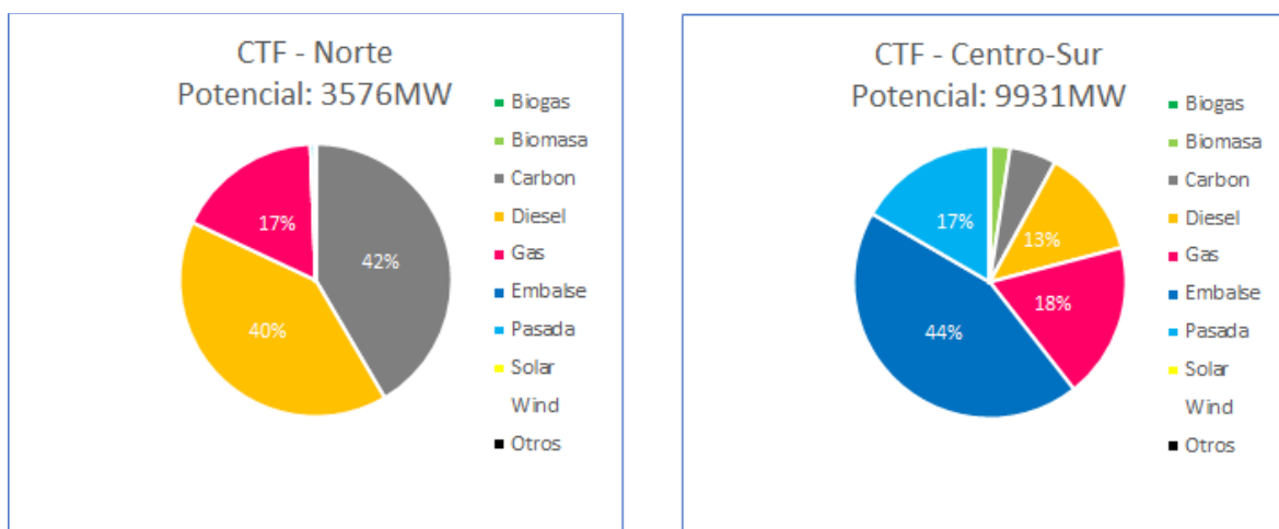
Figura 85. Potencial oferta CTF por zona y mix tecnológico
