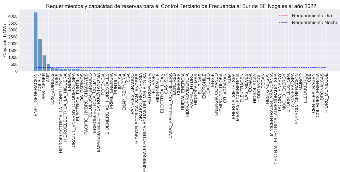
Figura A28. Requerimientos y capacidad de reservas para el Control Terciario de Frecuencia al Sur de la S/E Nogales al año 2022
