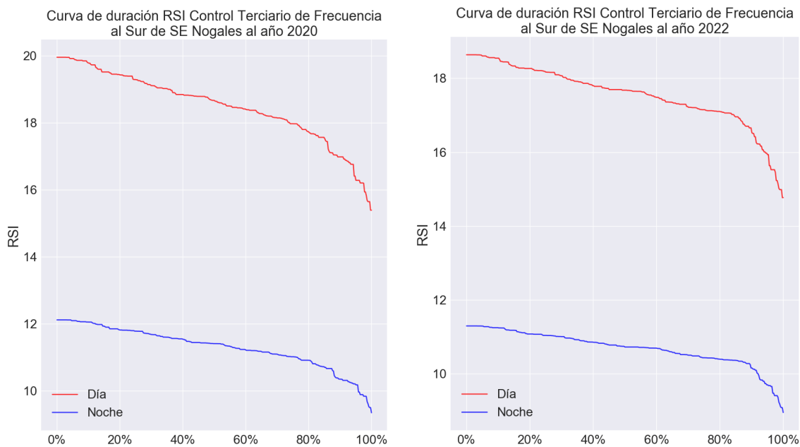
Figura 79. Curva de duración RSI del Control Terciario de Frecuencia al Sur de la S/E Nogales al año 2020 (izquierda) y 2022 (derecha)
