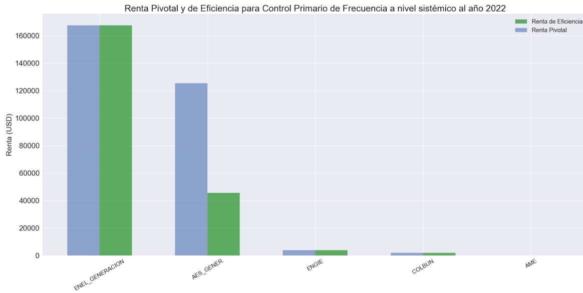
Figura 37. Renta Pivotal y de Eficiencia para el Control Primario de Frecuencia a nivel sistémico al año 2022
