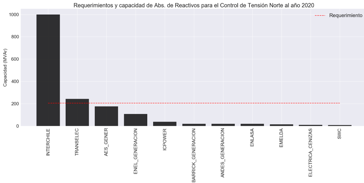
Figura 93. Requerimientos y capacidad de reservas para el Control de Tensión - Absorción de Reactivos en zona Norte al año 2020
