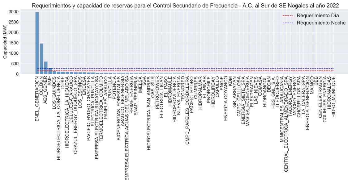
Figura A16. Requerimientos y capacidad de reservas para el Control Secundario de Frecuencia - Aumento de Carga al Sur de la S/E Nogales al año 2022
