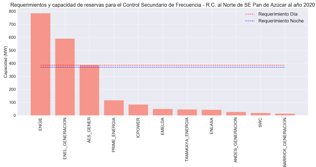
Figura 62. Requerimientos y capacidad de reservas para el Control Secundario de Frecuencia - Reducción de Carga al Norte de la S/E Pan de Azúcar al año 2020
