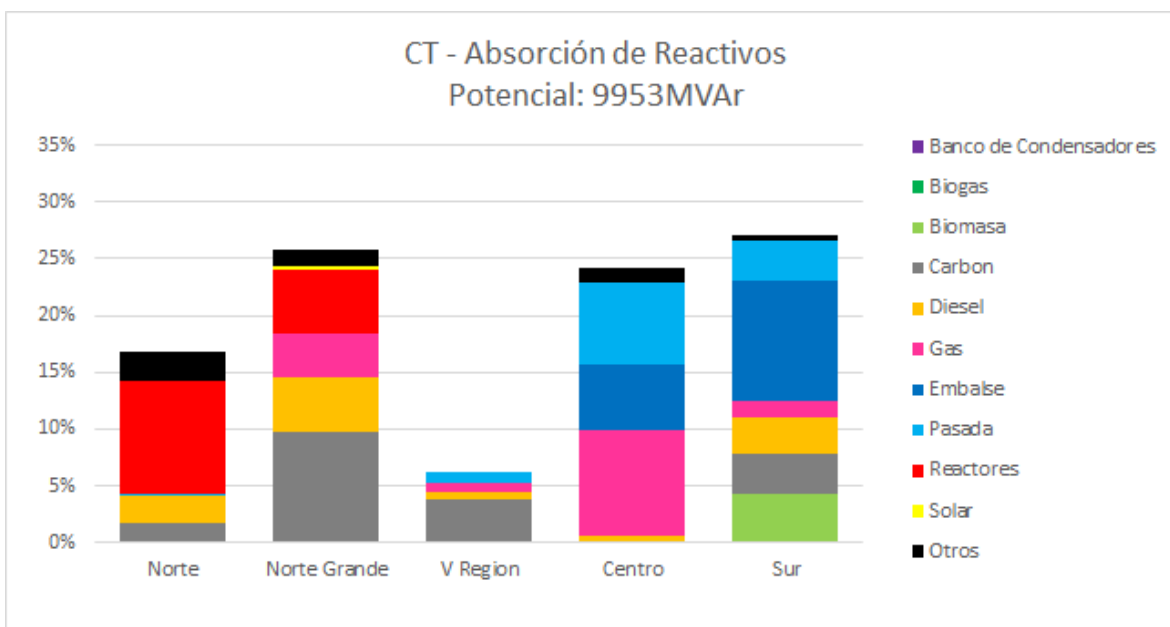
Figura 104. Potencial oferta CT - Absorción de Reactivos por zona y mix tecnológico
