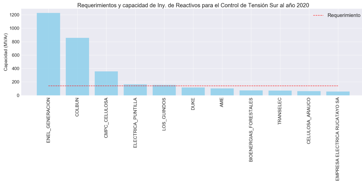
Figura 101. Requerimientos y capacidad de reservas para el Control de Tensión - Inyección de Reactivos en zona Sur al año 2020
