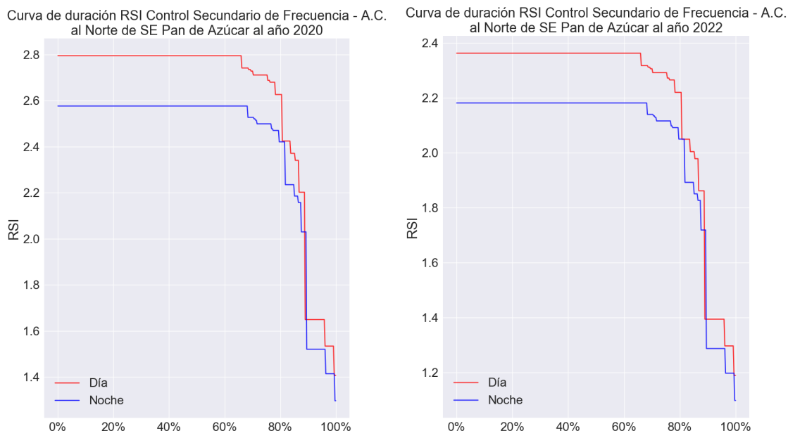
Figura 49. Curva de duración RSI del Control Secundario de Frecuencia - Aumento de Carga al Norte de la S/E Pan de Azúcar al año 2020 (izquierda) y 2022 (derecha)
