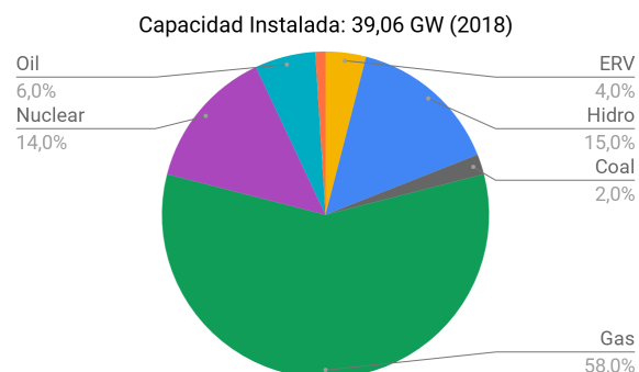
Figura 3: Composición de la matriz energética de NYISO
