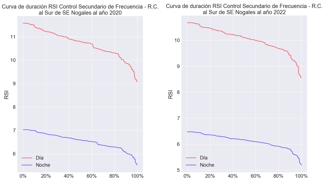
Figura 67. Curva de duración RSI del Control Secundario de Frecuencia - Reducción de Carga al Sur de la S/E Nogales al año 2020 (izquierda) y 2022 (derecha)
