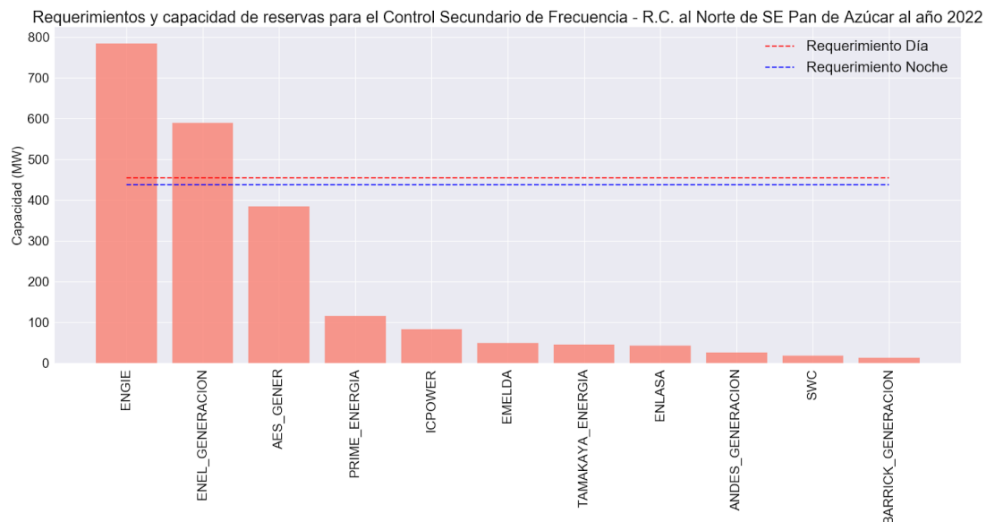
Figura 63. Requerimientos y capacidad de reservas para el Control Secundario de Frecuencia - Reducción de Carga al Norte de la S/E Pan de Azúcar al año 2022
