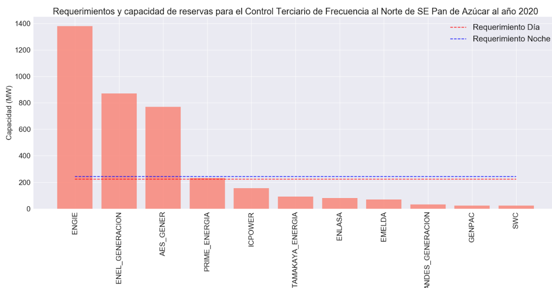
Figura 74. Requerimientos y capacidad de reservas para el Control Terciario de Frecuencia al Norte de la S/E Pan de Azúcar al año 2020
