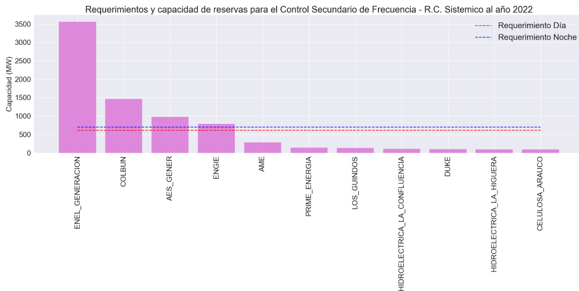
Figura 60. Requerimientos y capacidad de reservas para el Control Secundario de Frecuencia - Reducción de Carga a nivel Sistémico al año 2022
