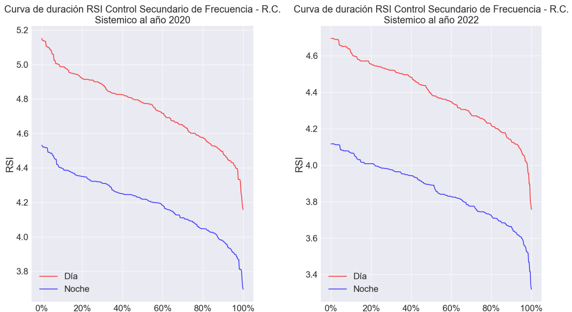
Figura 61. Curva de duración RSI del Control Secundario de Frecuencia - Reducción de Carga a nivel Sistémico al año 2020 (izquierda) y 2022 (derecha)
