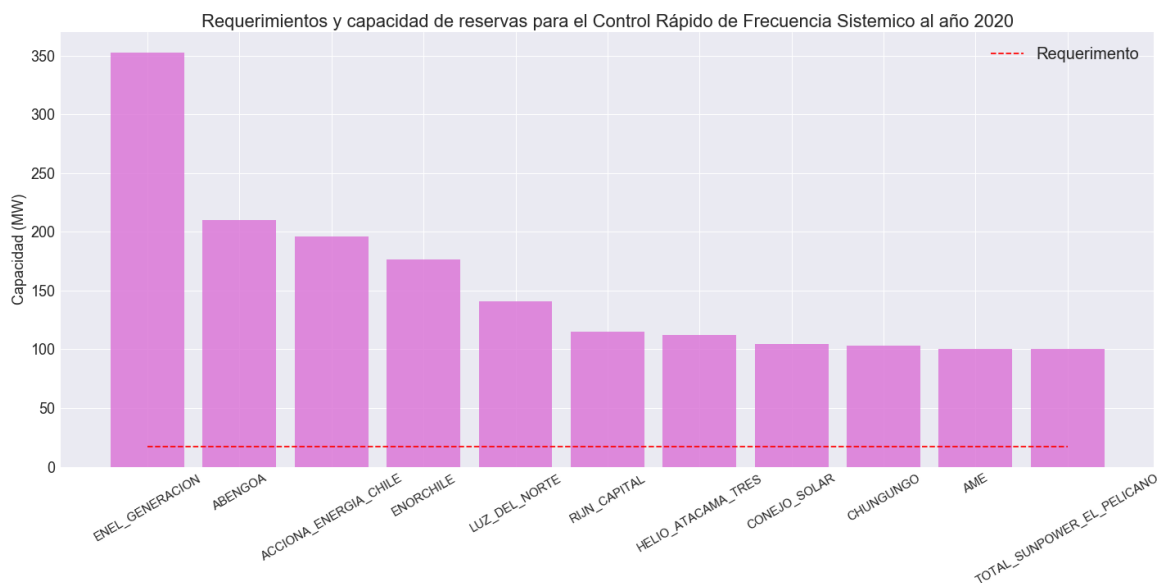
Figura 20. Requerimientos y Capacidad de Reservas para el Control Rápido de Frecuencia a Nivel Sistémico al año 2020
