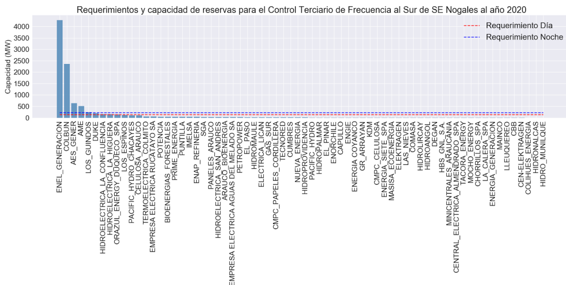
Figura A27. Requerimientos y capacidad de reservas para el Control Terciario de Frecuencia al Sur de la S/E Nogales al año 2020
