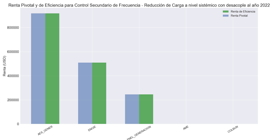
Figura 69. Renta Pivotal y de Eficiencia para el Control Secundario de Frecuencia - Reducción de Carga a nivel sistémico con desacople al año 2022
