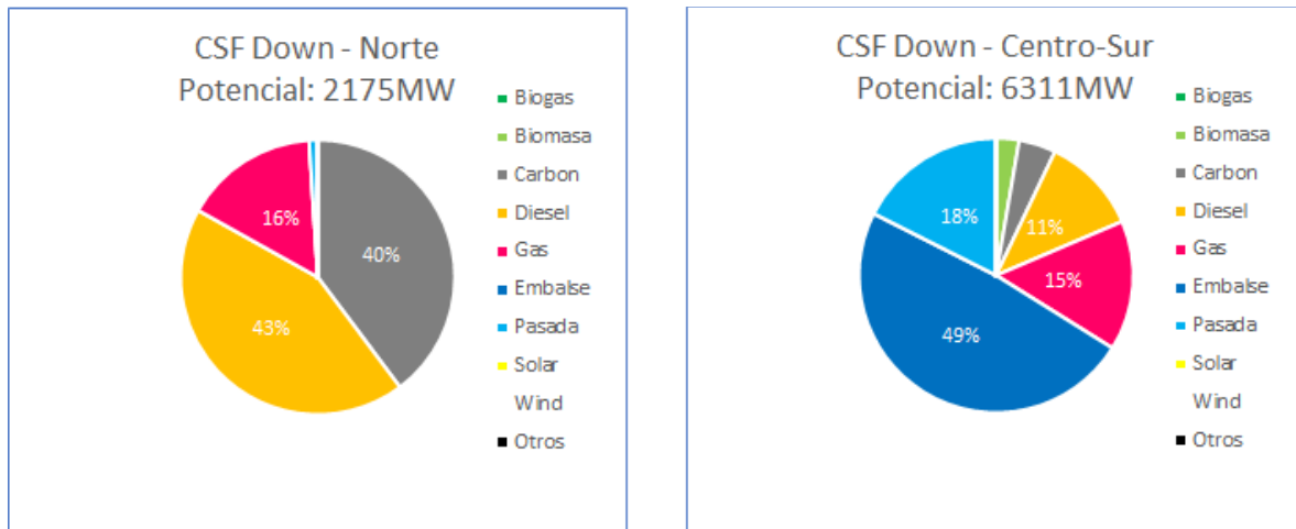
Figura 70. Potencial oferta CSF - Reducción de Carga por zona y mix tecnológico
