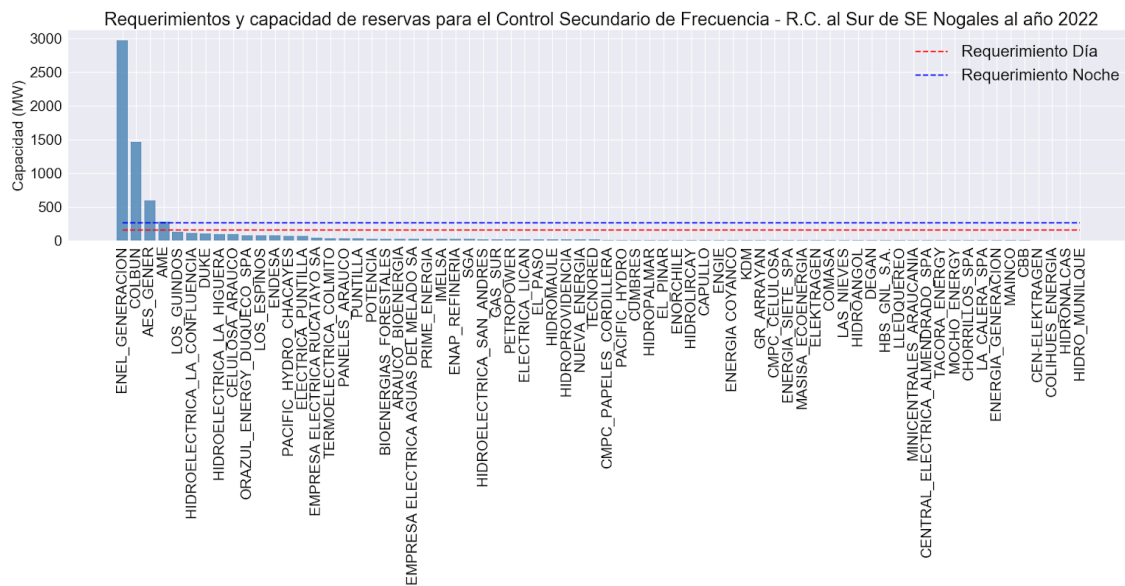
Figura A22. Requerimientos y capacidad de reservas para el Control Secundario de Frecuencia - Reducción de Carga al Sur de la S/E Nogales al año 2022
