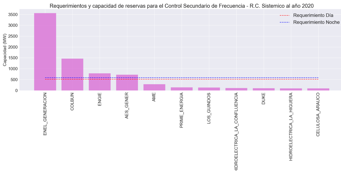
Figura 59. Requerimientos y capacidad de reservas para el Control Secundario de Frecuencia - Reducción de Carga a nivel Sistémico al año 2020
