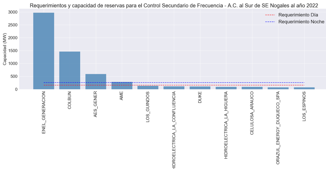
Figura 51. Requerimientos y capacidad de reservas para el Control Secundario de Frecuencia - Aumento de Carga al Sur de la S/E Nogales al año 2022
