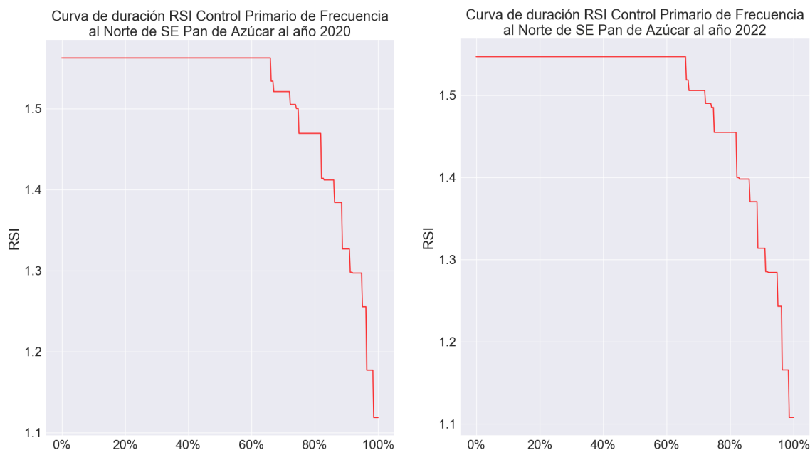
Figura 31. Curva de duración RSI del Control Primario de Frecuencia al Norte de la S/E Pan de Azúcar al año 2020 (izquierda) y 2022 (derecha)
