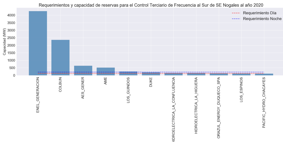
Figura 77. Requerimientos y capacidad de reservas para el Control Terciario de Frecuencia al Sur de la S/E Nogales al año 2020
