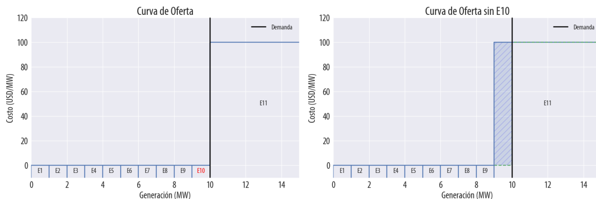
Figura A1. Curva de oferta del Ejemplo 1 con (izquierda) y sin (derecha) un generador.
