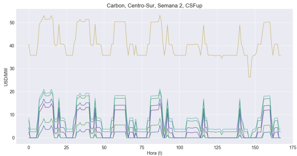
Figura 106. Banda de Precios de Reserva Secundaria - Aumento de Carga para unidades de Carbón en zona Centro-Sur para la segunda semana representativa.
