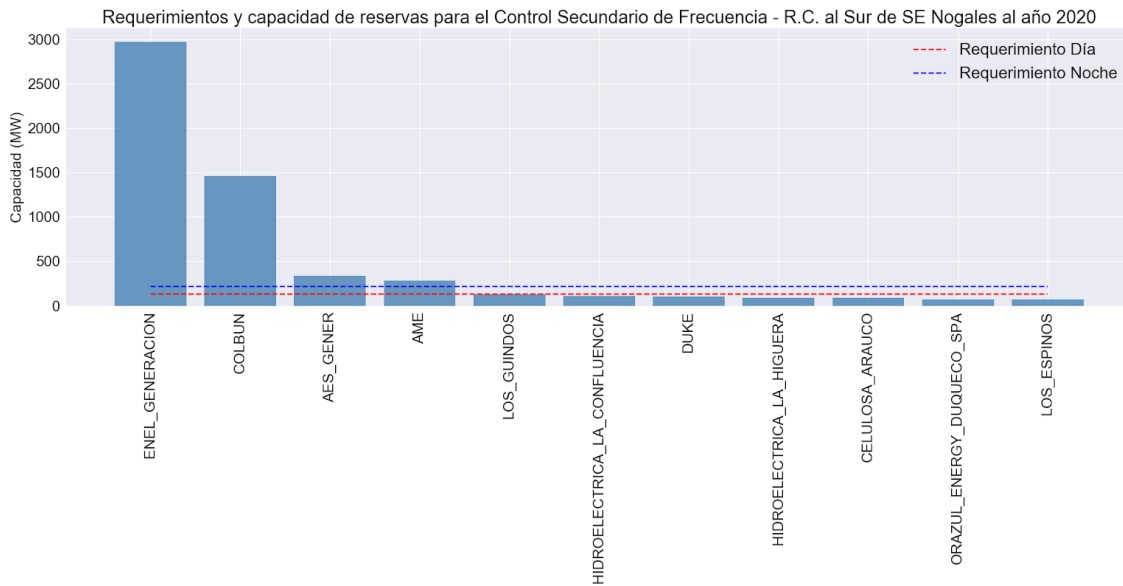
Figura 65. Requerimientos y capacidad de reservas para el Control Secundario de Frecuencia - Reducción de Carga al Sur de la S/E Nogales de Azúcar al año 2020
