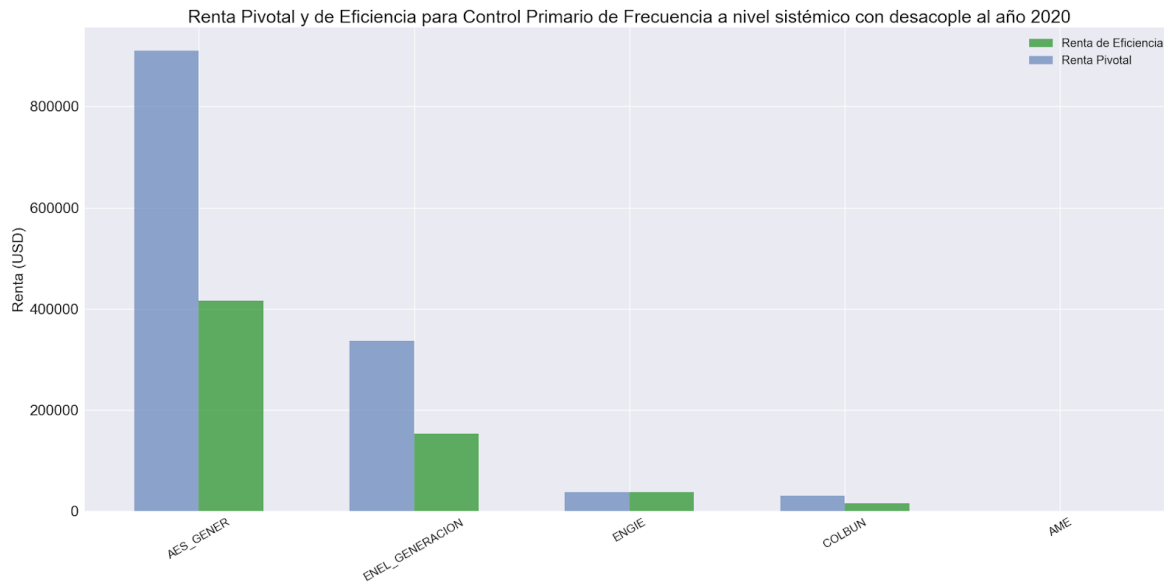
Figura 39. Renta Pivotal y de Eficiencia para el Control Primario de Frecuencia a nivel sistémico con desacople al año 2020
