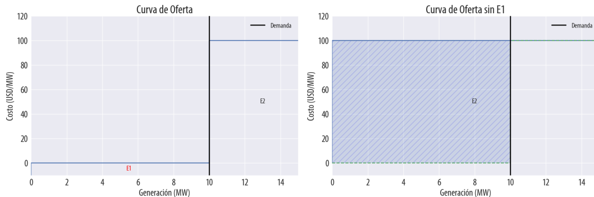
Figura A2. Curva de oferta del Ejemplo 2 con (izquierda) y sin (derecha) un generador.
