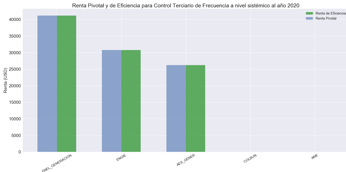
Figura 80. Renta Pivotal y de Eficiencia para Control Terciario de Frecuencia a nivel sistémico al año 2020
