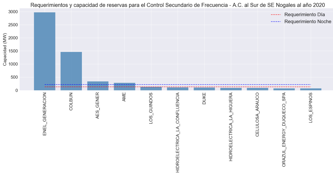
Figura 50. Requerimientos y capacidad de reservas para el Control Secundario de Frecuencia - Aumento de Carga al Sur de la S/E Nogales al año 2020
