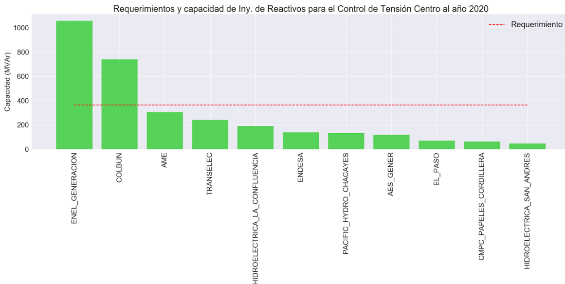
Figura 98. Requerimientos y capacidad de reservas para el Control de Tensión - Inyección de Reactivos en zona Centro al año 2020
