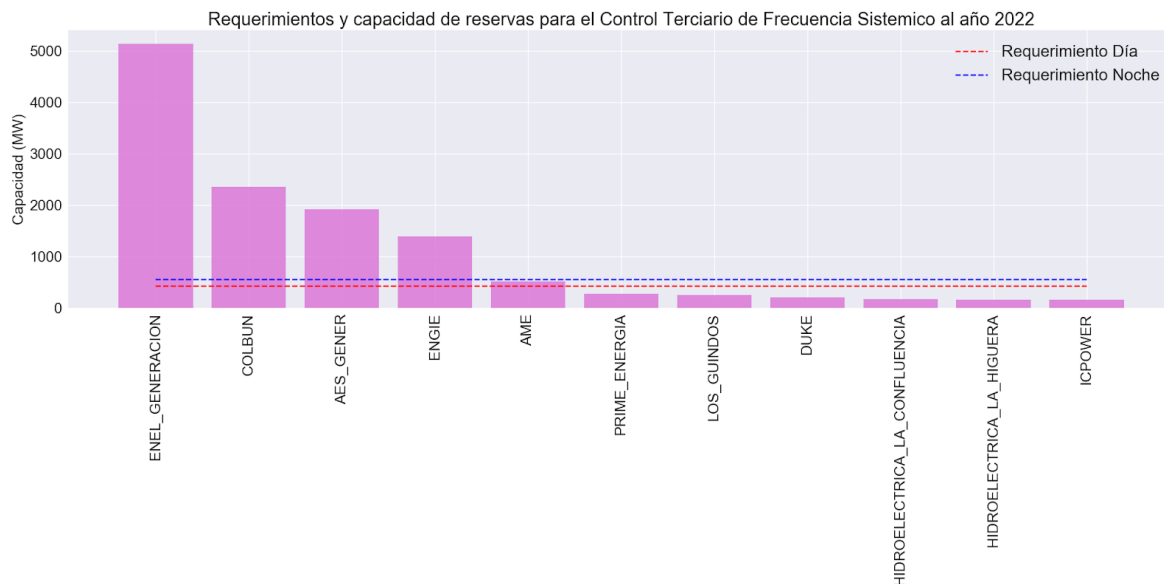
Figura 72. Requerimientos y capacidad de reservas para el Control Terciario de Frecuencia a nivel Sistémico al año 2022
