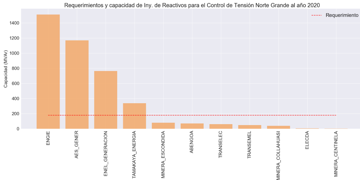
Figura 89. Requerimientos y capacidad de reservas para el Control de Tensión - Inyección de Reactivos en zona Norte Grande al año 2020
