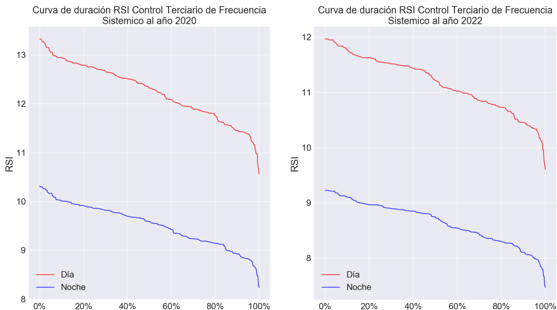
Figura 73. Curva de duración RSI del Control Terciario de Frecuencia a nivel Sistémico al año 2020 (izquierda) y 2022 (derecha)
