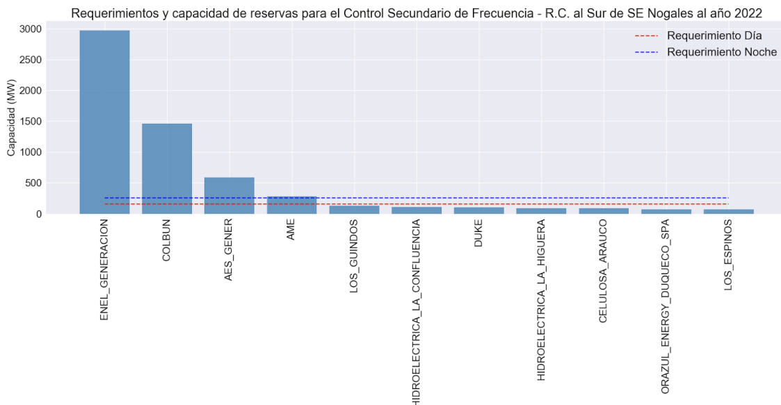
Figura 66. Requerimientos y capacidad de reservas para el Control Secundario de Frecuencia - Reducción de Carga al Sur de la S/E Nogales de Azúcar al año 2020
