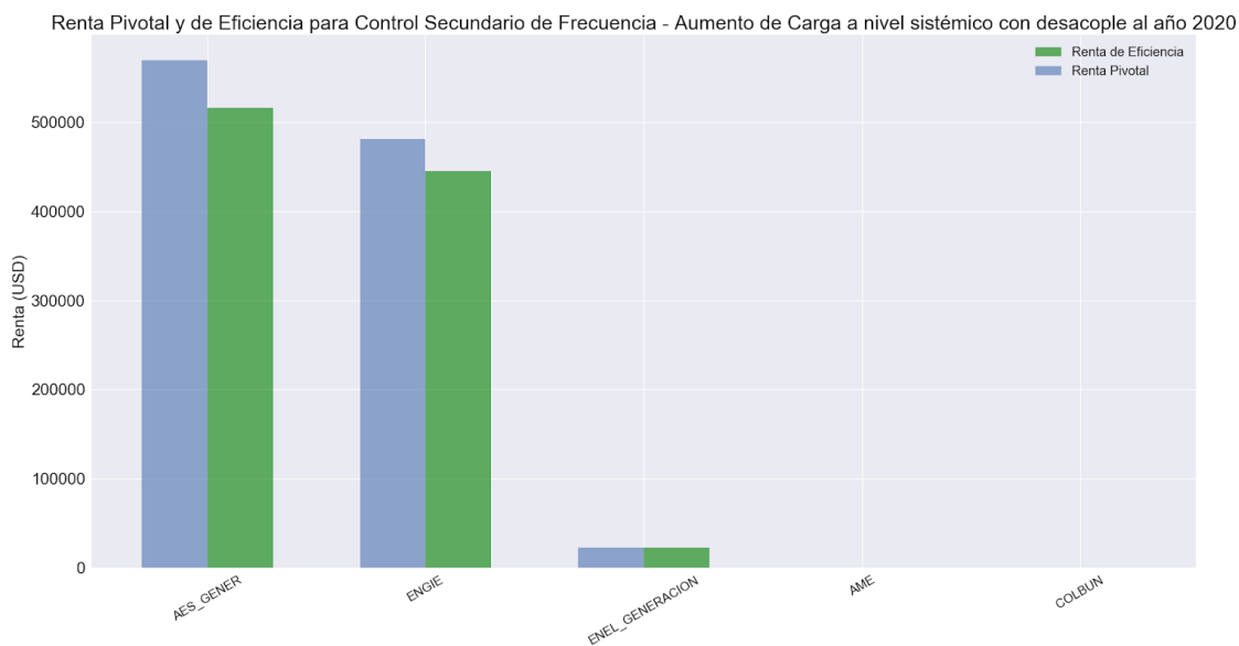
Figura 55. Renta Pivotal y de Eficiencia para el Control Secundario de Frecuencia - Aumento de Carga a nivel sistémico con desacople al año 2020
