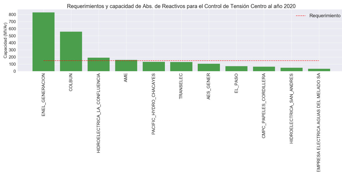
Figura 99. Requerimientos y capacidad de reservas para el Control de Tensión - Absorción de Reactivos en zona Centro al año 2020
