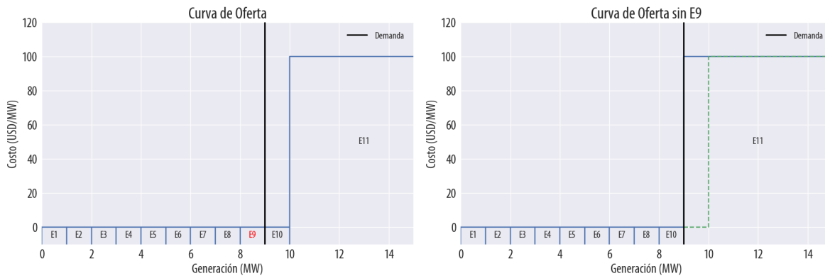
Figura A3. Curva de oferta del Ejemplo 3 con (izquierda) y sin (derecha) un generador.
