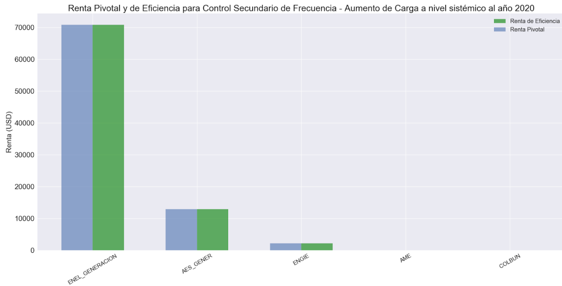
Figura 53. Renta Pivotal y de Eficiencia para el Control Secundario de Frecuencia - Aumento de Carga a nivel sistémico al año 2020
