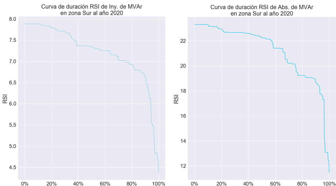
Figura 103. Curva de duración RSI para el Control de Tensión - Inyección de Reactivos (izquierda) y Absorción de Reactivos (derecha) en zona Sur al año 2020
