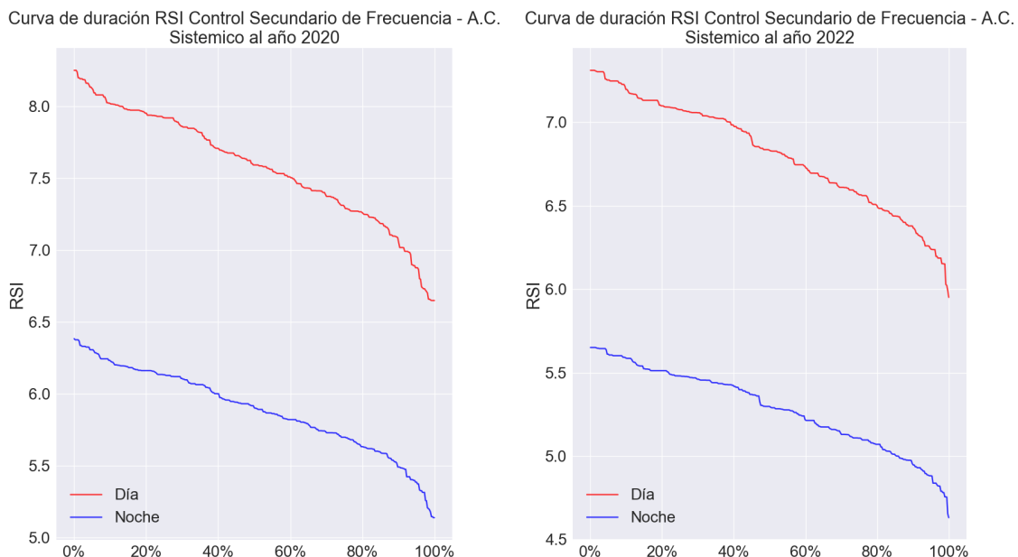
Figura 46. Curva de duración RSI del Control Secundario de Frecuencia - Aumento de Carga a nivel Sistémico al año 2020 (izquierda) y 2022 (derecha)
