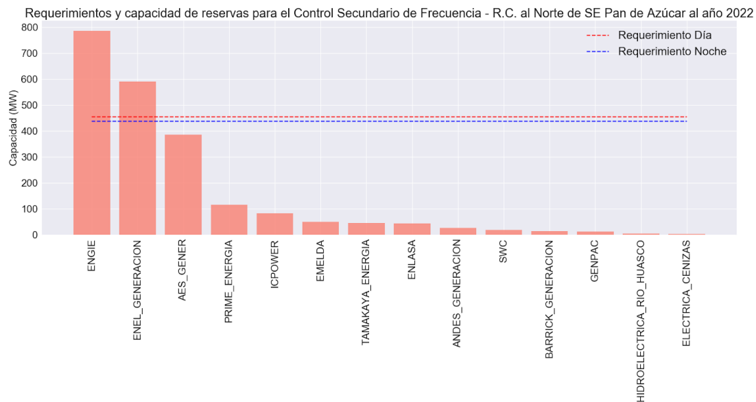
Figura A20. Requerimientos y capacidad de reservas para el Control Secundario de Frecuencia - Reducción de Carga al Norte de la S/E Pan de Azúcar al año 2022
