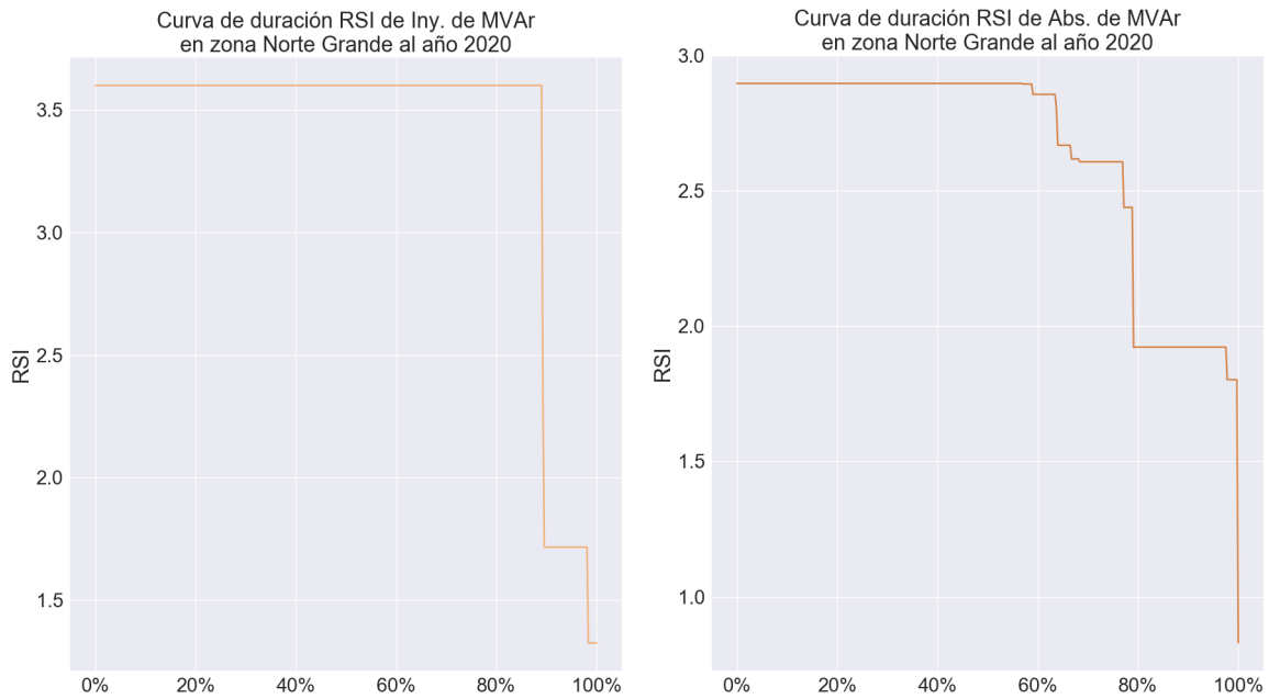
Figura 91. Curva de duración RSI para el Control de Tensión - Inyección de Reactivos (izquierda) y Absorción de Reactivos (derecha) en zona Norte Grande al año 2020
