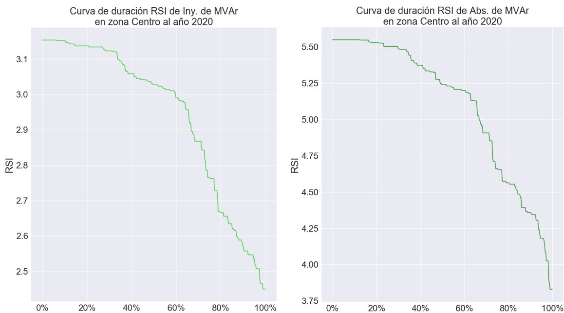
Figura 100. Curva de duración RSI para el Control de Tensión - Inyección de Reactivos (izquierda) y Absorción de Reactivos (derecha) en zona Centro al año 2020
