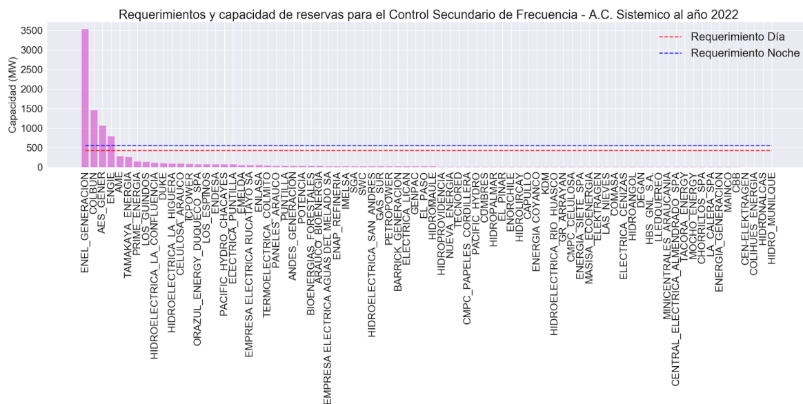
Figura A12. Requerimientos y capacidad de reservas para el Control Secundario de Frecuencia - Aumento de Carga a nivel Sistémico al año 2022
