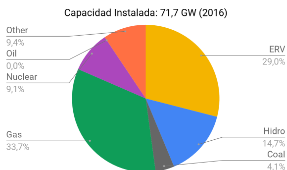
Figura 2: Composición de la matriz energética de CAISO
