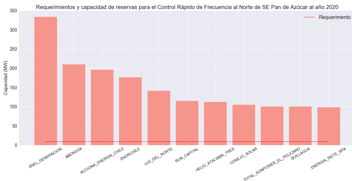
Figura 22. Requerimientos y Capacidad de Reservas Para el Control Rápido de Frecuencia al Norte de la S/E Pan de Azúcar al año 2020
