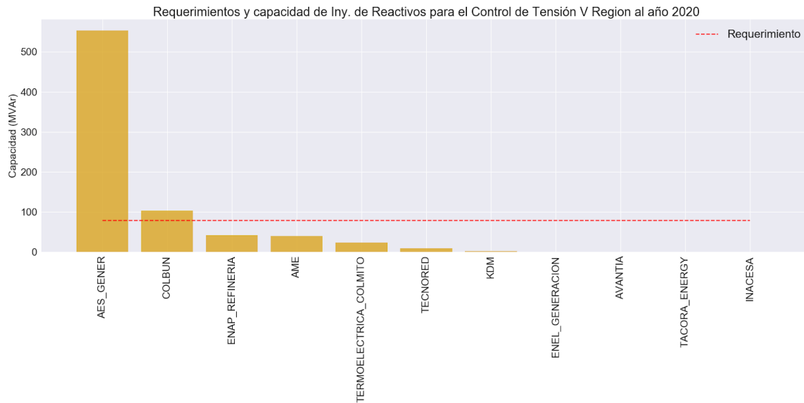
Figura 95. Requerimientos y capacidad de reservas para el Control de Tensión - Inyección de Reactivos en zona V Región al año 2020
