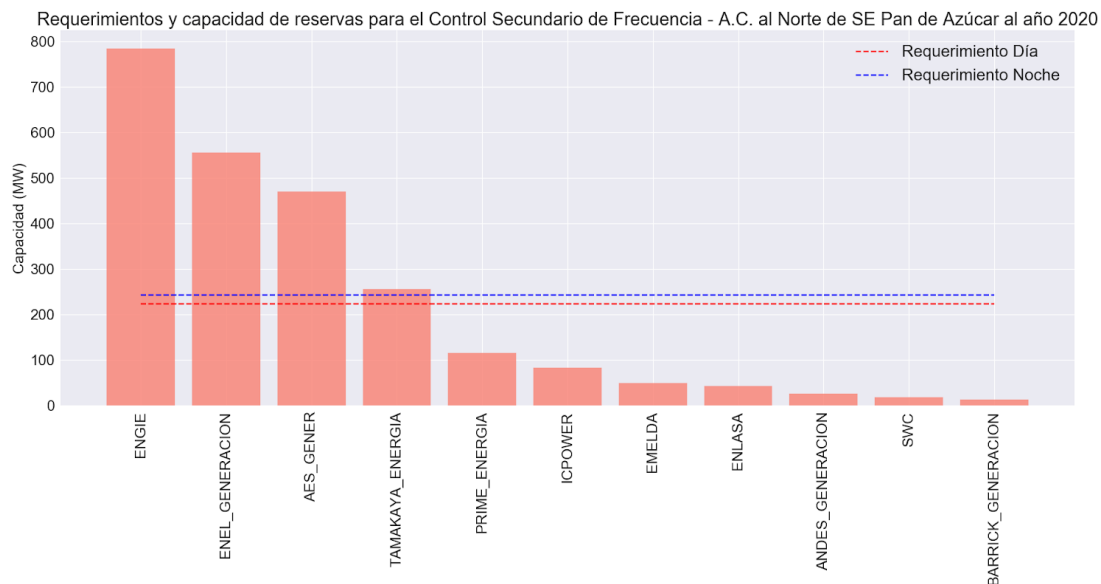
Figura 47. Requerimientos y capacidad de reservas para el Control Secundario de Frecuencia - Aumento de Carga al Norte de la S/E Pan de Azúcar al año 2020
