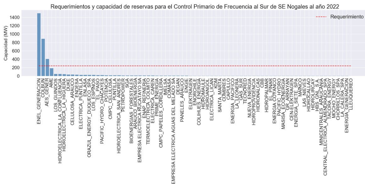
Figura A10. Requerimientos y capacidad de reservas para el Control Primario de Frecuencia al Sur de la S/E Nogales al año 2022
