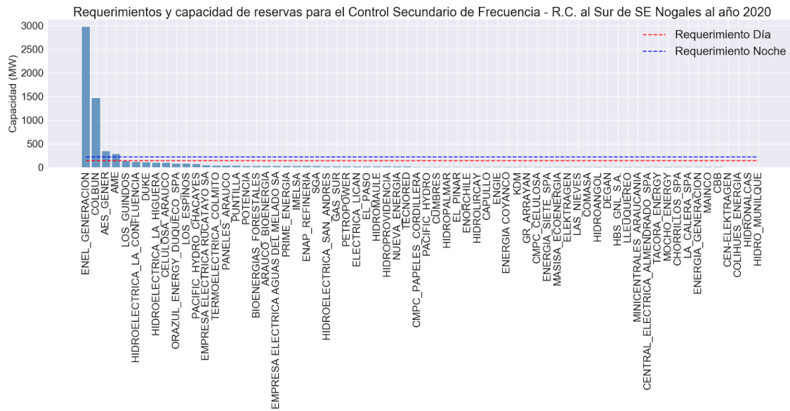
Figura A21. Requerimientos y capacidad de reservas para el Control Secundario de Frecuencia - Reducción de Carga al Sur de la S/E Nogales al año 2020
