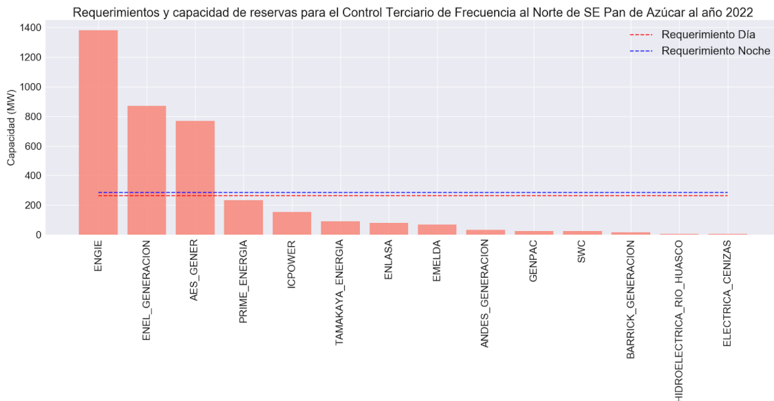
Figura A26. Requerimientos y capacidad de reservas para el Control Terciario de Frecuencia al Norte de la S/E Pan de Azúcar al año 2022
