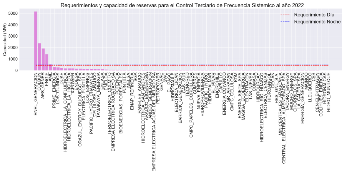
Figura A24. Requerimientos y capacidad de reservas para el Control Terciario de Frecuencia a nivel Sistémico al año 2022
