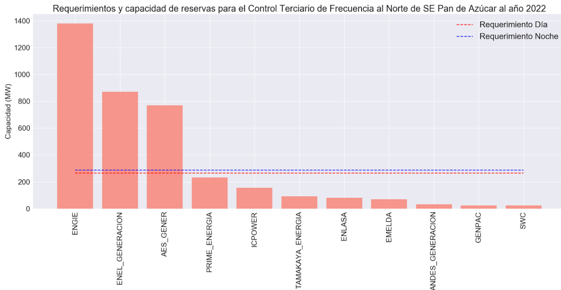
Figura 75. Requerimientos y capacidad de reservas para el Control Terciario de Frecuencia al Norte de la S/E Pan de Azúcar al año 2022
