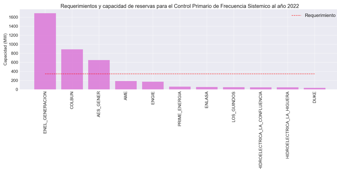
Figura 27. Requerimientos y capacidad de reservas para el Control Primario de Frecuencia a nivel Sistémico al año 2022
