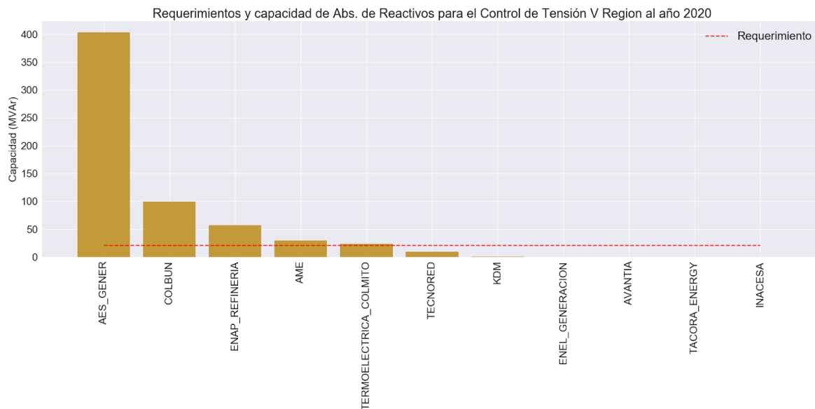
Figura 96. Requerimientos y capacidad de reservas para el Control de Tensión - Absorción de Reactivos en zona V Región al año 2020
