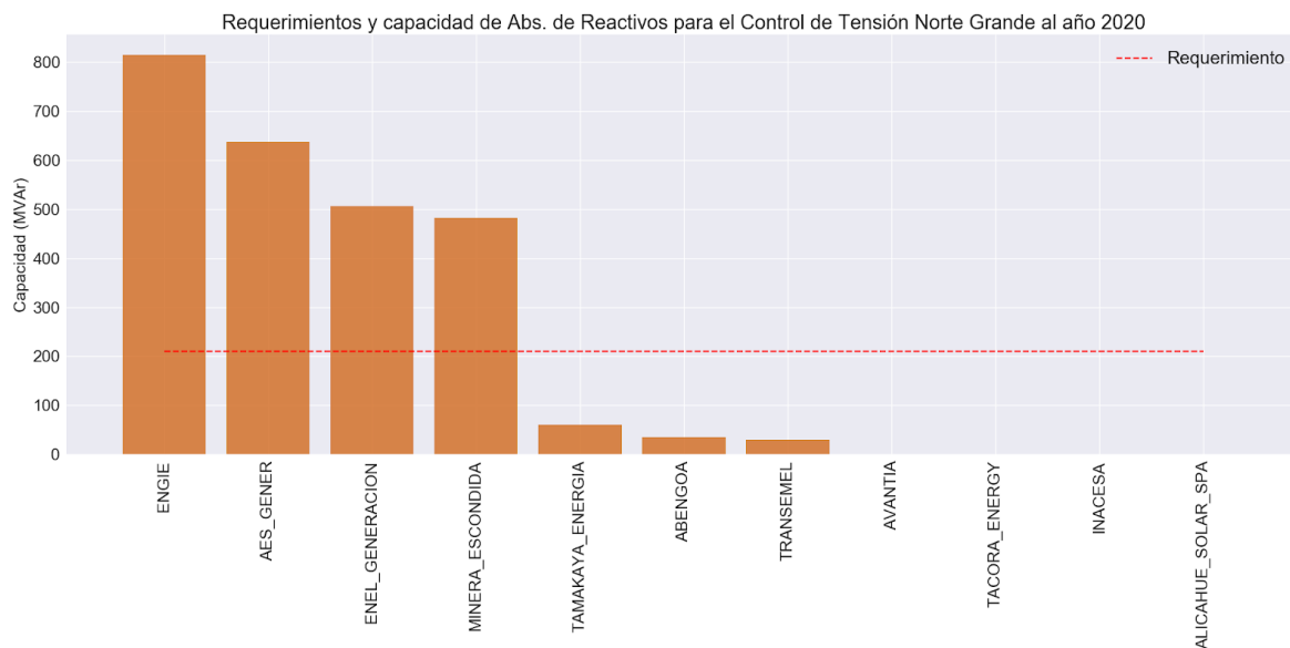
Figura 90. Requerimientos y capacidad de reservas para el Control de Tensión - Absorción de Reactivos en zona Norte Grande al año 2020
