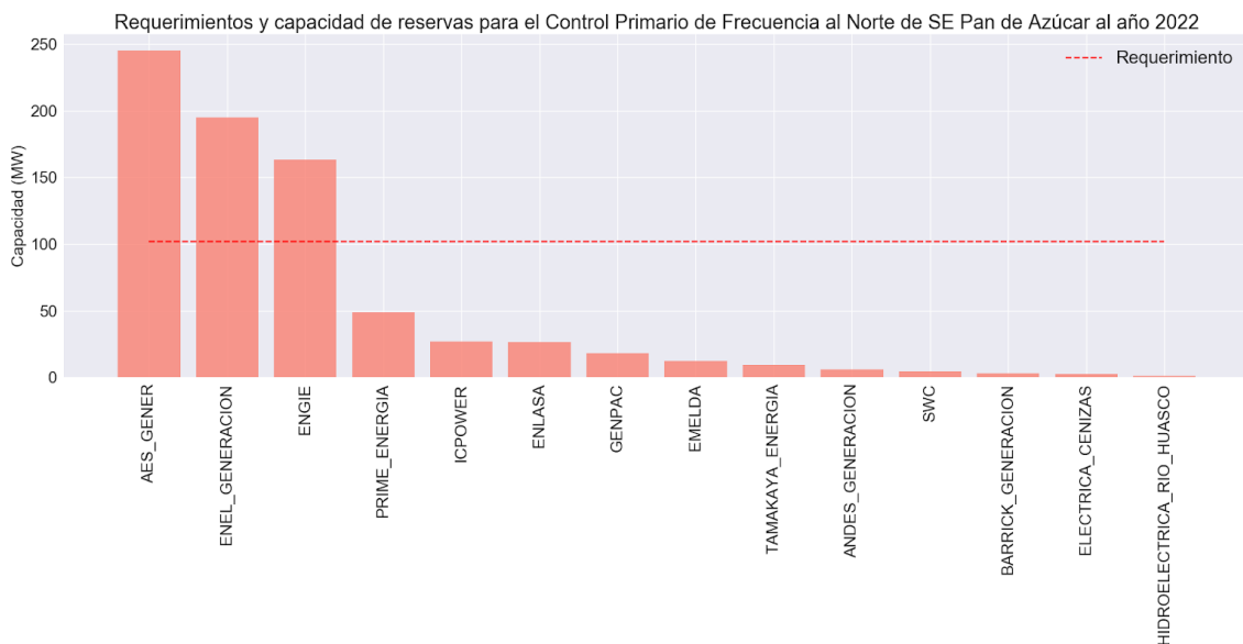
Figura A8. Requerimientos y capacidad de reservas para el Control Primario de Frecuencia al Norte de la S/E Pan de Azúcar al año 2022
