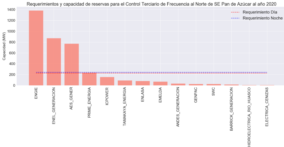
Figura A25. Requerimientos y capacidad de reservas para el Control Terciario de Frecuencia al Norte de la S/E Pan de Azúcar al año 2020
