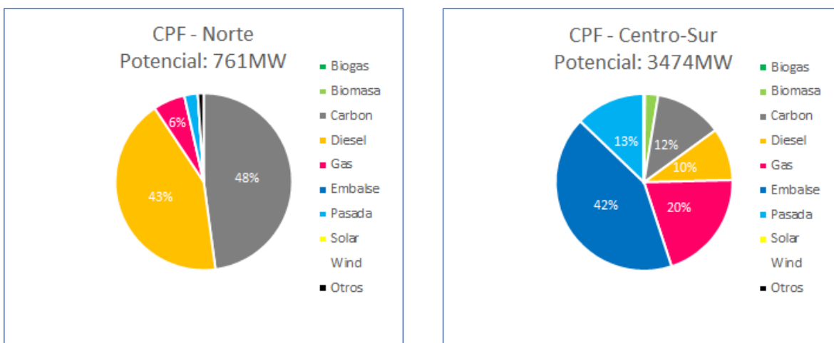
Figura 43. Potencial oferta CPF por zona y mix tecnológico
