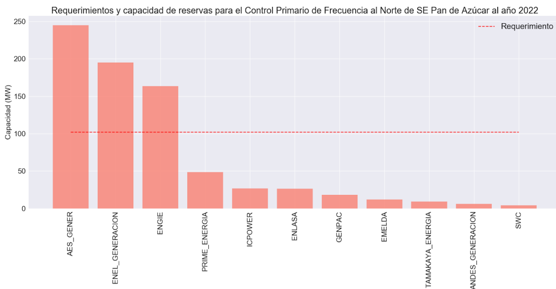
Figura 30. Requerimientos y capacidad de reservas para el Control Primario de Frecuencia al Norte de la S/E Pan de Azúcar al año 2022
