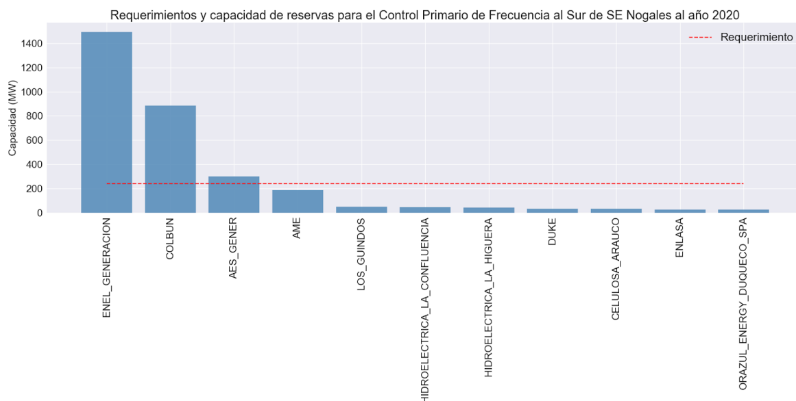
Figura 32. Requerimientos y capacidad de reservas para el Control Primario de Frecuencia al Sur de la S/E Nogales al año 2020
