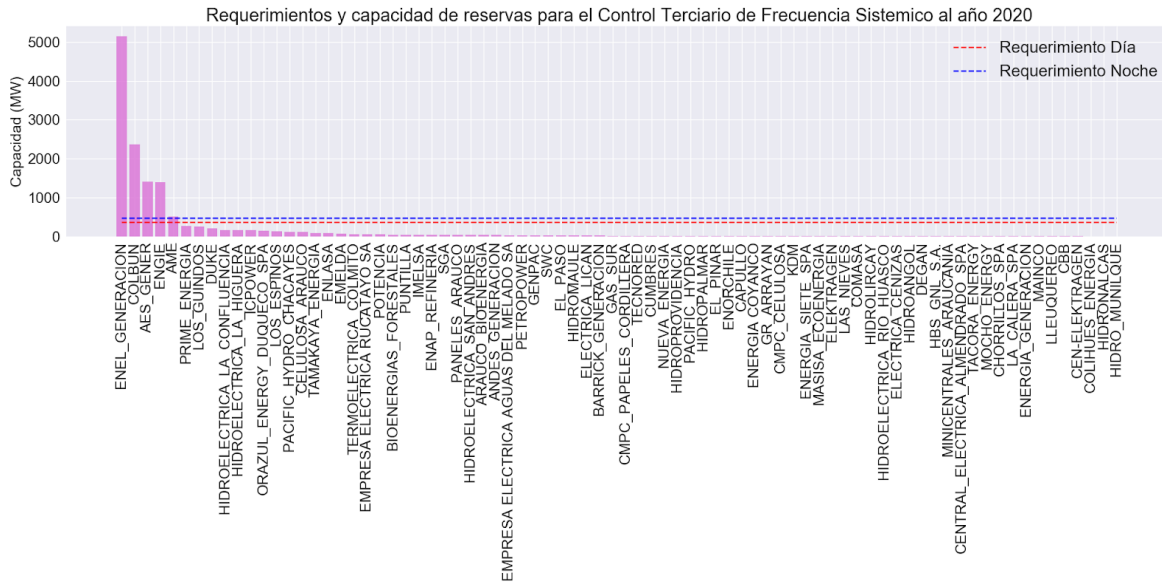
Figura A23. Requerimientos y capacidad de reservas para el Control Terciario de Frecuencia a nivel Sistémico al año 2020
