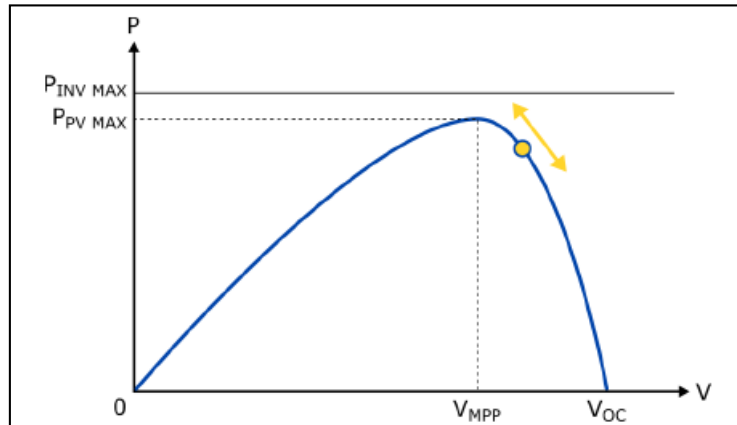
Imagen 3: Algoritmo MPPT. La máxima producción de energía se produce en el punto PPV MAX; VMPP.
