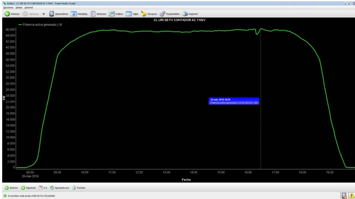
Imagen 5: Registro técnico potencia activa en S/E URIBE SOLAR (110 kV).
