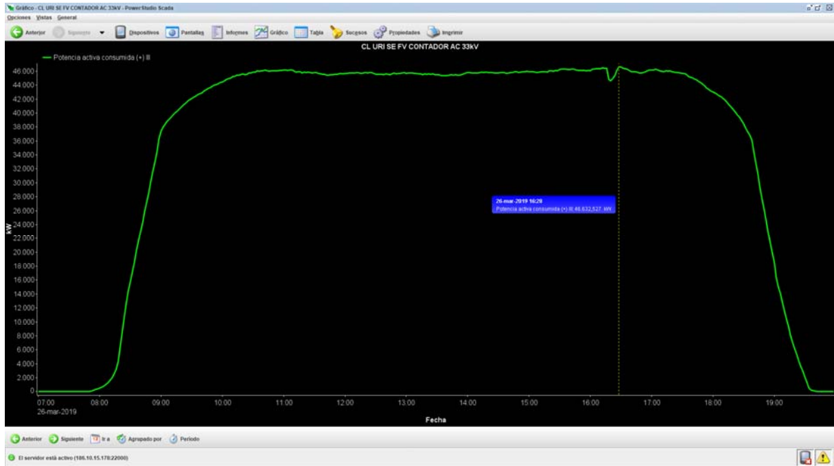
Imagen 6: Registro técnico potencia activa en S/E URIBE SOLAR (33 kV).
