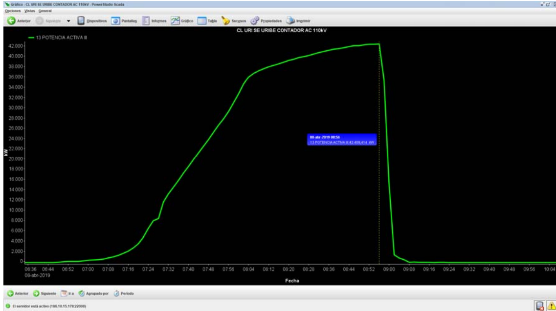
Imagen 4: Registro técnico Parque PV Uribe Solar.
