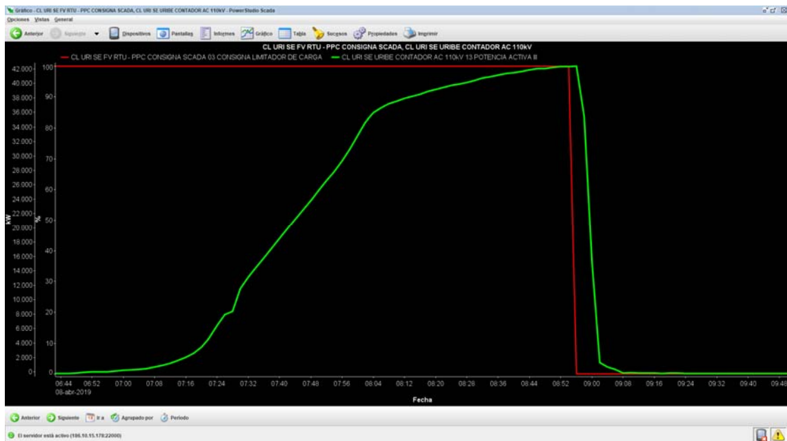
Imagen 2: Registros de mínimo técnico Parque PV Uribe Solar.
