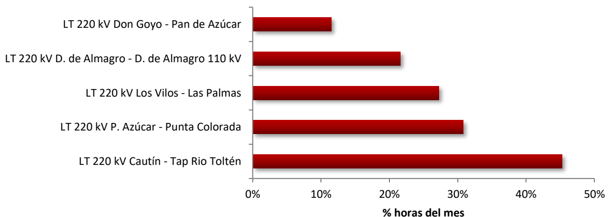
Figura 2: Mayores Tiempos de Desacople en el SEN mes actual.
