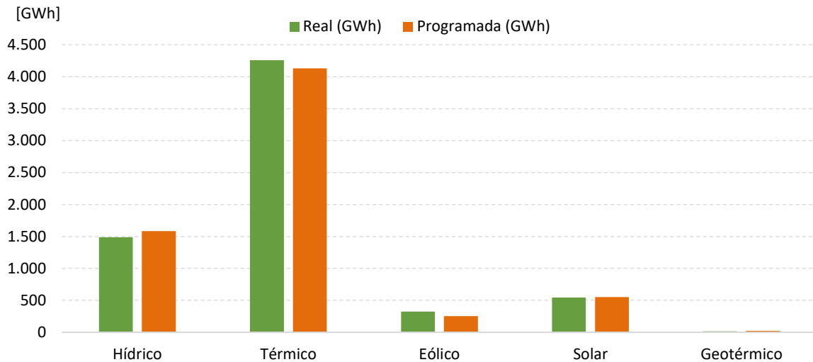
Figura 6: Comparación Generación Real y Programada por fuente.
