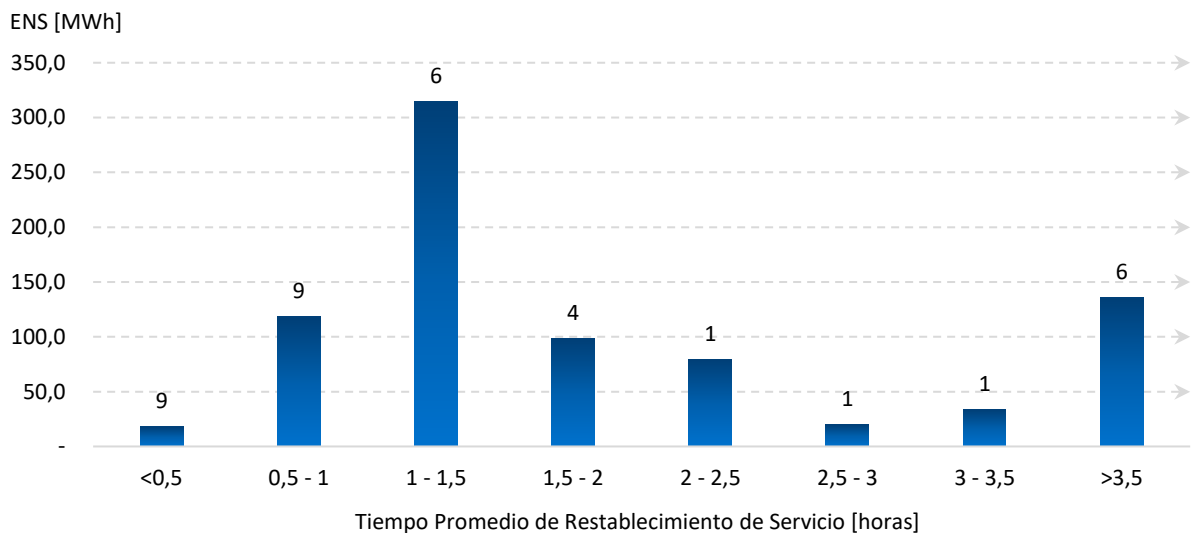
Figura 12: ENS según duración de falla marzo-19 (resultados preliminares).
