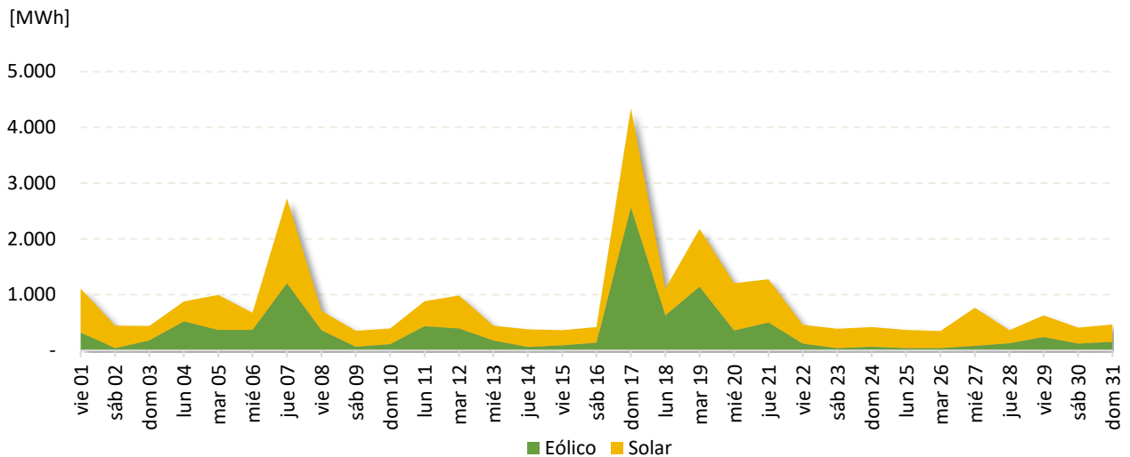
Figura 3: Reducción ERNC mes actual.
