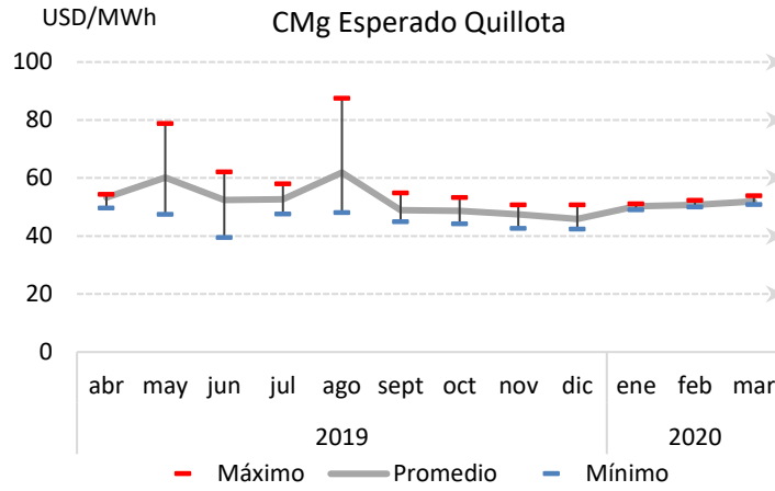
Figura 21: Costo marginal esperado en S/E 220 kV Quillota.
