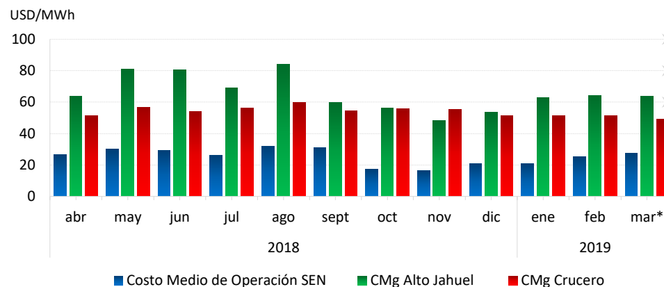
Figura 5: Costos Medios de Operación y Costos Marginales de Crucero y Alto Jahuel 220 kV. Marzo valor estimado.
