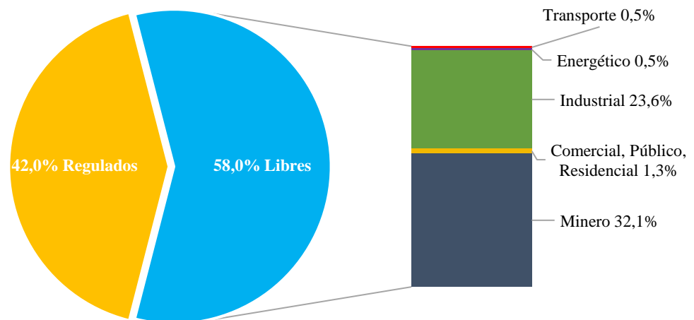
Figura 11: Retiros físicos por sector SEN febrero-19.
