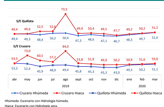
Figura 2.9. CMg Proyectado Mensual [USD/MWh]: SS/EE Quillota y Cruceiro
