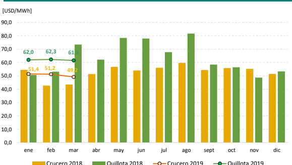
Figura 2.8. CMg Promedio Mensual [USD/MWh]: SS/EE Quillota y Cruceiro
