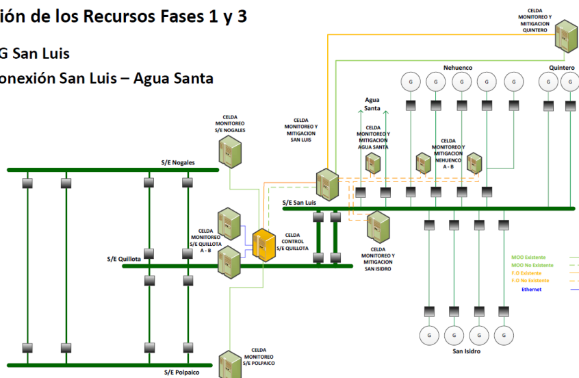
Figura 1: Esquema de implementación de recursos EDAG San Luis y Desconexión vínculo San Luis-Agua Santa
