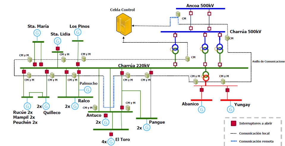
Figura 3: Esquema de implementación de recursos EDAG Charrúa
