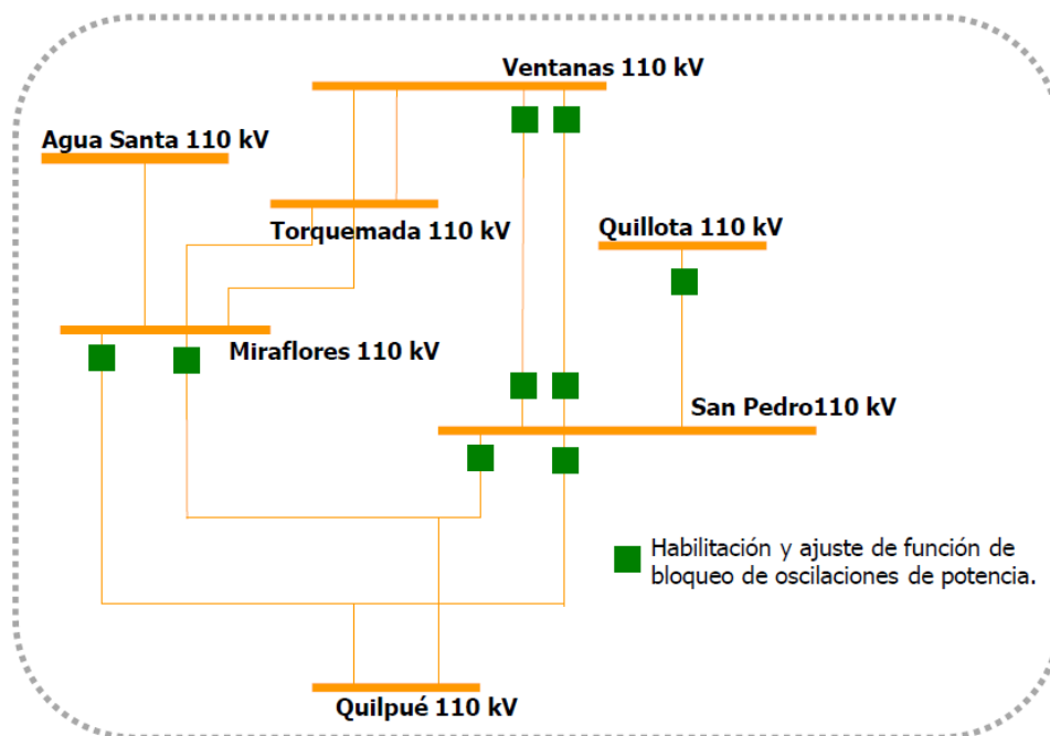
Figura 2: Ajuste Protecciones (Fase 3)
