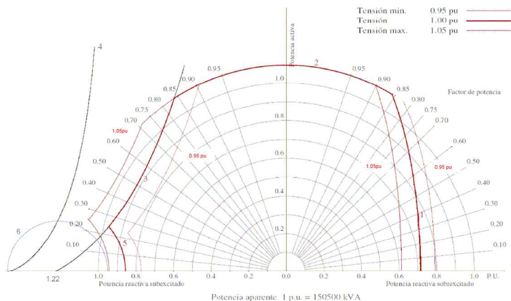
Figura 1: Diagrama PQ Angostura 2.
