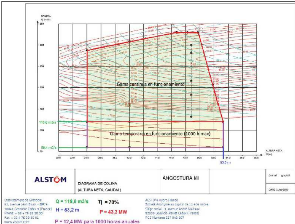
Figura 2: Curva de colina Angostura 2.
