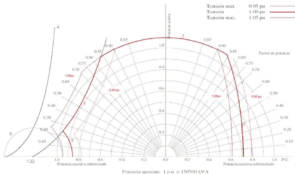
Figura 1: Diagrama PQ Angostura 1.
