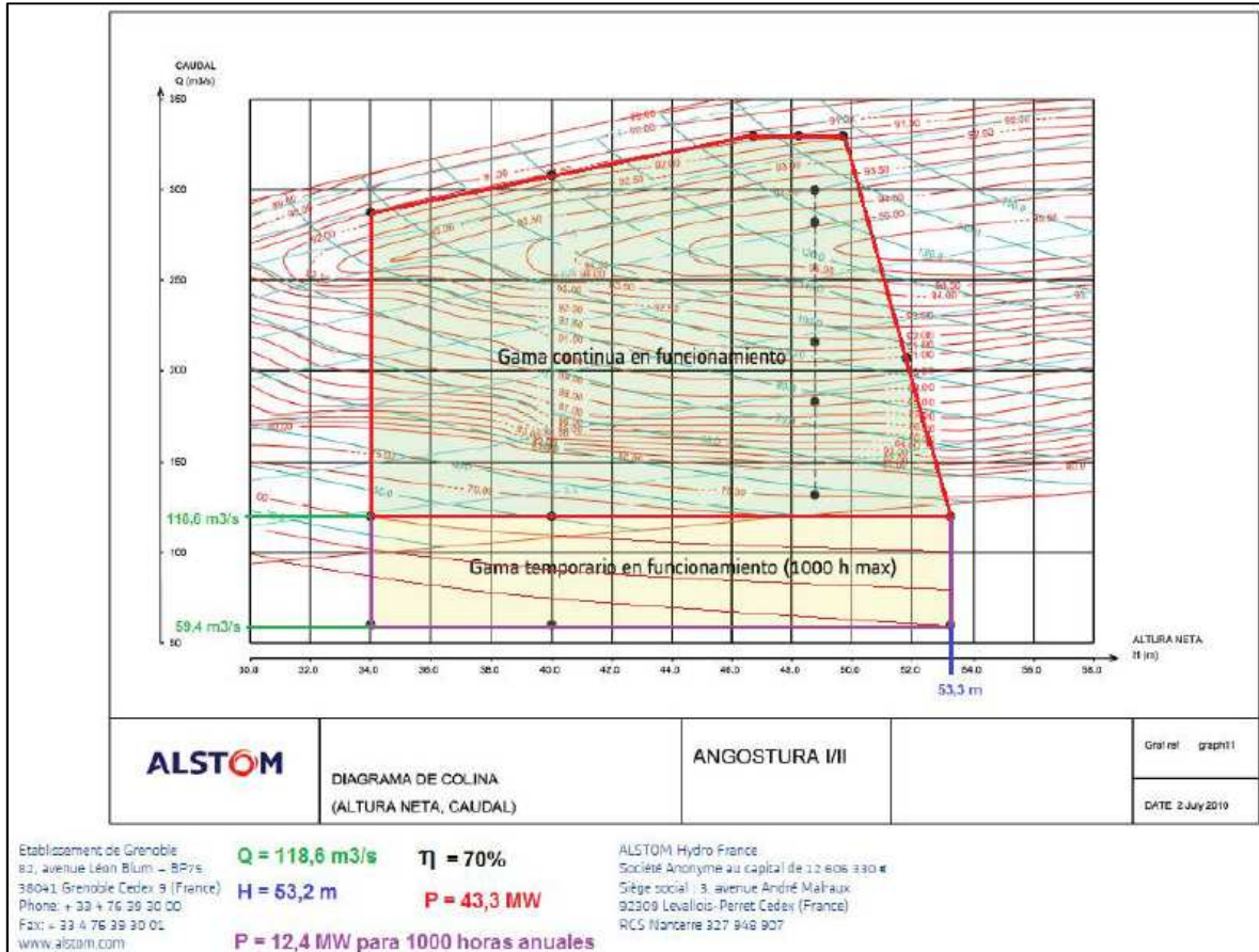
Figura 2: Curva de colina Angostura 1.
