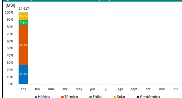
Figura 2.1. Capacidad Instalada de Generación [MW]
