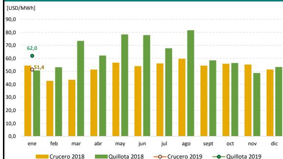
Figura 2.7. CMg Promedio Mensual [USD/MWh]: SS/EE Quillota y Crucero
