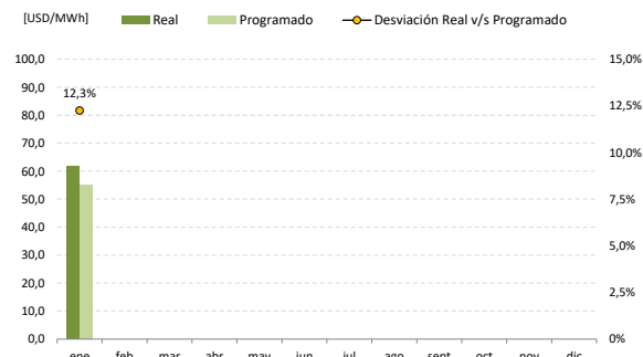
Figura 1.8. CMg Promedio Mensual [USD/MWh]: S/E Quillota 220 kV
