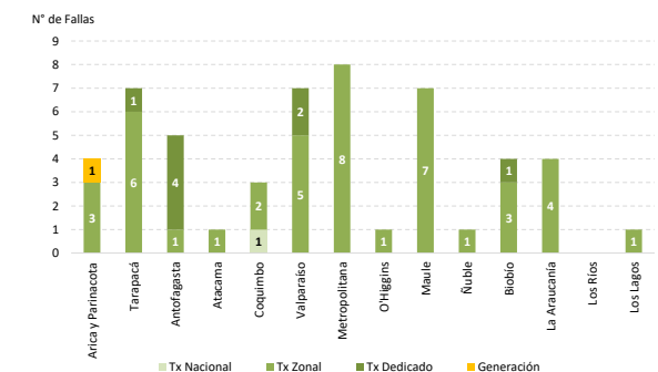
Figura 1.9. Fallas en el SEN (por Región y Segmento de Origen)
