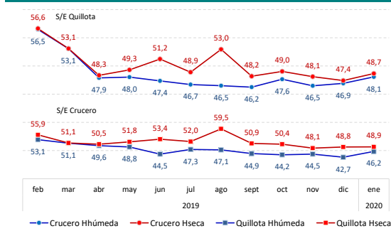
Figura 2.8. CMg Proyectado Mensual [USD/MWh]: SS/EE Quillota y Crucero
