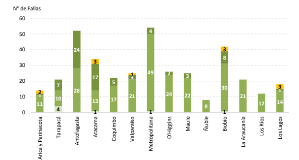
Figura 1.9. Fallas en el SEN (por Región y Segmento de Origen)
