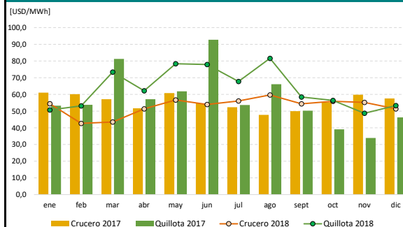
Figura 2.7. CMg Promedio Mensual [USD/MWh]: SS/EE Quillota y Cruceo
