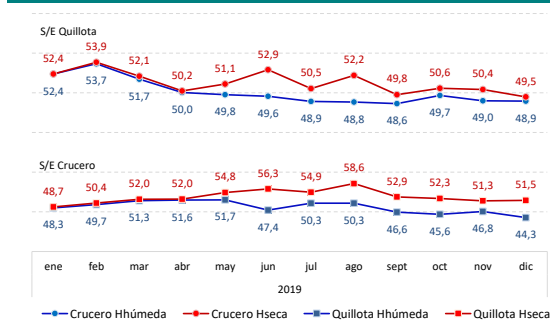
Figura 2.8. CMg Proyectado Mensual [USD/MWh]: SS/EE Quillota y Cruceo
