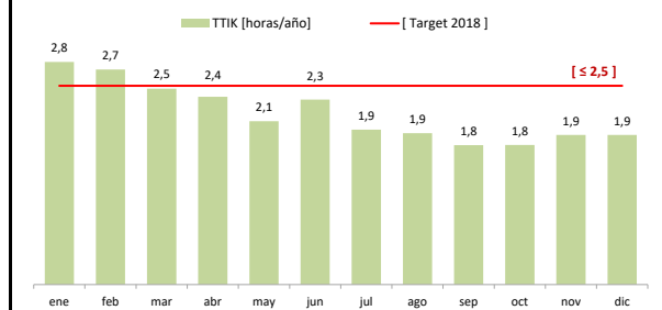
Figura 1.4. Tiempo Total de Interrupciones de Suministro - TTIK
